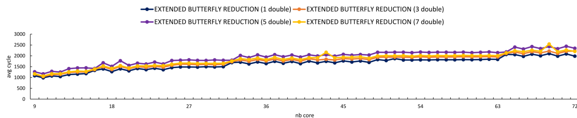
Figure 4.15 – Coût moyen de la réductions de 1, 3 et 7 valeurs sur le processeur KNL avec le compilateur Intel 21.4.
