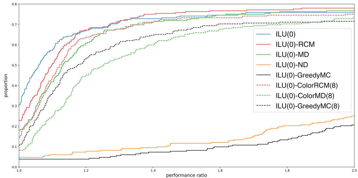
Figure 2.7 – Représentations des performance profiles des différentes renumérations par rapport à leur nombre d’itérations. Le nombre de matrices total est de 232 matrices avec 11 configurations soit 2552 tests. Les courbes en pointillés sont les coloriages avec limitation de la taille des couleurs (COLORRCM(8), COLORMD(8) et GREEDYMC(8)).
