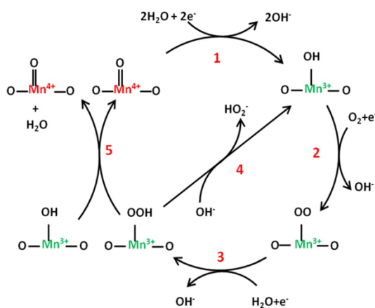
Fig. 1. Mécanisme de l'ORR proposé par Rybova et al. [2].
