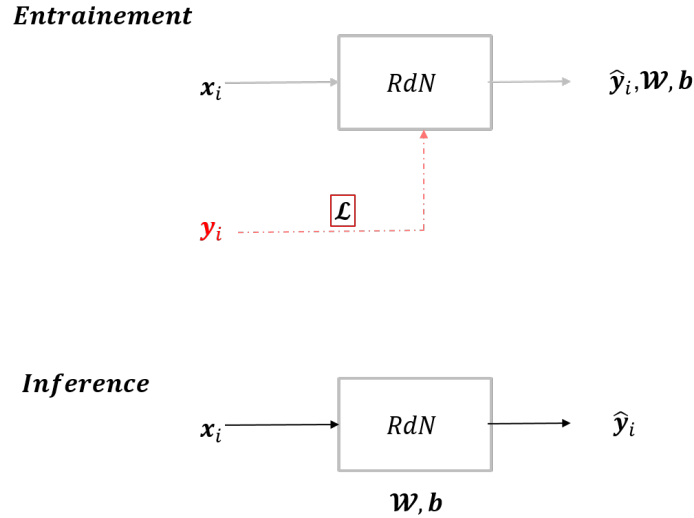
FIGURE 4.3 – Deux modes de fonctionnement du RdN : le mode d’entraînement qui vient minimiser les paramètres du réseau pour le calibrer en comparant la prédiction de sortie \hat{y} avec la vérité terrain y grâce à la fonction de coût \mathcal{L} ; et le mode d’inférence qui correspond au mode d’utilisation opérationnel du RdN. Il associe une prédiction \hat{y} à une entrée x
