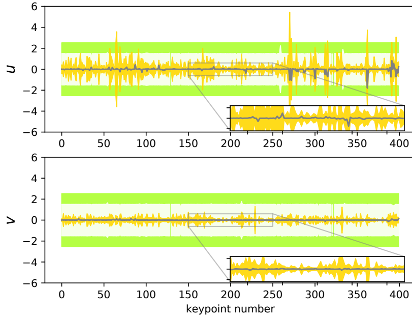
FIGURE 5.12 – Comparaison des prédictions de DUNE à l’état de l’art - La ligne grise représente l’erreur dans les directions u et v d’un scénario avec un mouvement rectiligne, \blacksquare décrit la méthode Fix-C à 3\sigma , \square fait référence à [WM17] pour 3\sigma et \blacksquare représente les prédictions d’incertitudes issues de DUNE à 3\sigma .
