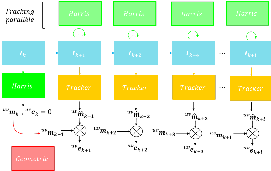
FIGURE 4.10 – Schéma fonctionnel du procédé de construction de la base de données d'apprentissage appliquée au dataset SYNTHIA
