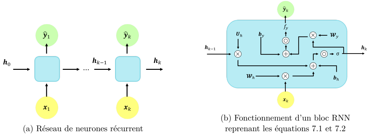
FIGURE 7.1 – Fonctionnement d'un réseau de neurones récurrent générique
