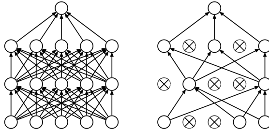
FIGURE 5.2 – Dropout aléatoire appliqué aux neurones d’entrée de chaque couche. Figure issue de [Sri+14]
