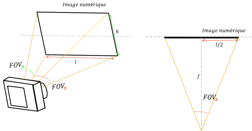
FIGURE 2.7 – Représentation des champs de vue selon les axes x et y
