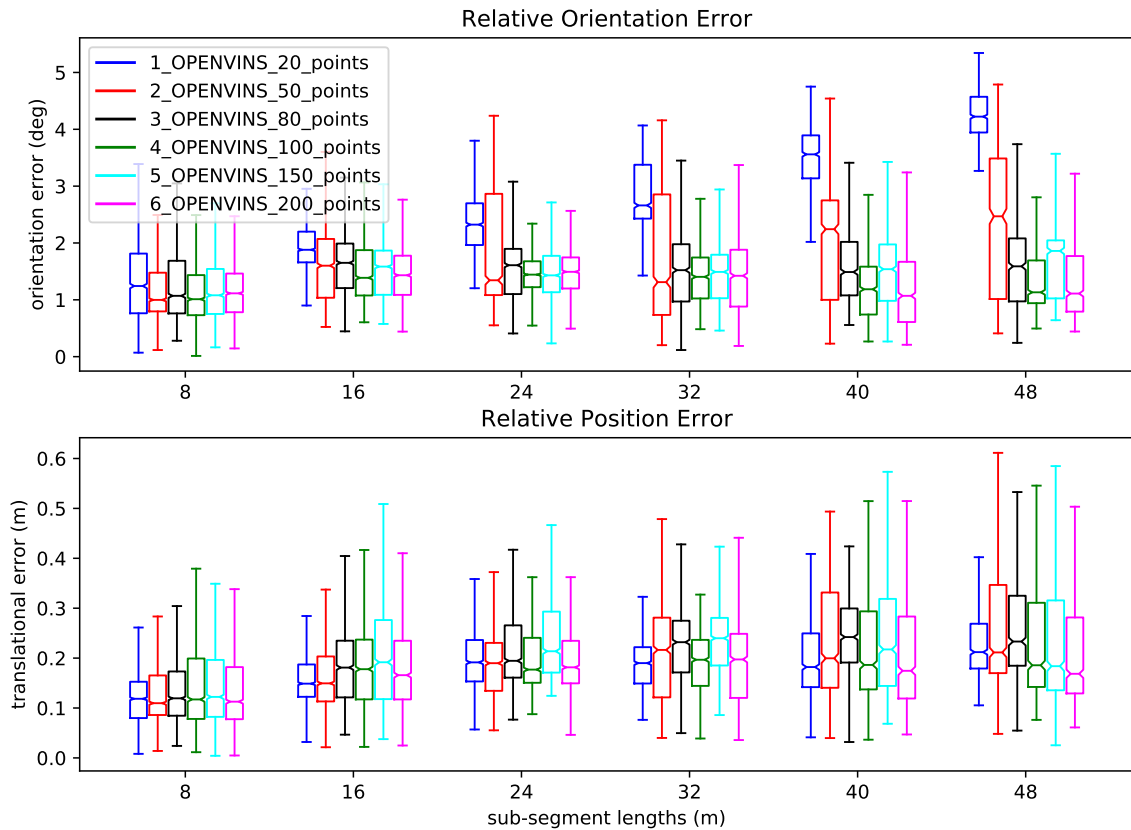
FIGURE 6.3 – Évaluation de RPE(deg/m) sur l'influence du nombre de points dans OpenVINS
