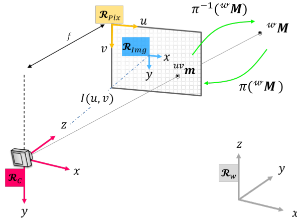
FIGURE 2.4 – Modèle sténopé
