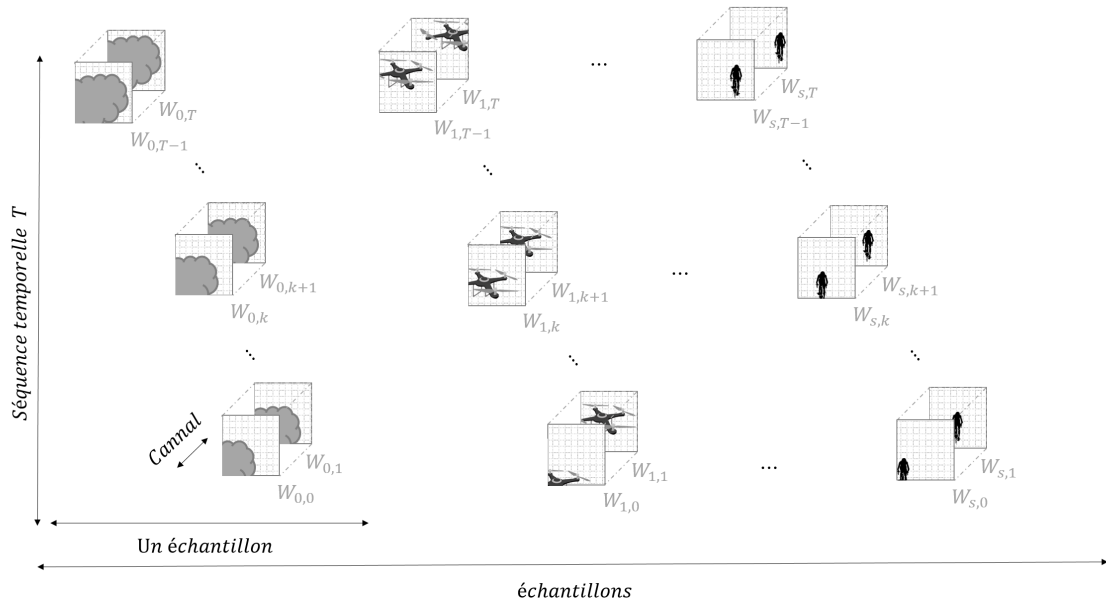
FIGURE 7.5 – Format des données de DUNE-M - concatenation des fenêtres centrées en {}^{uv}\tilde{\mathbf{m}}_k et {}^{uv}\tilde{\mathbf{m}}_{k+1} , \forall k \in \llbracket 0; T \rrbracket . Un échantillon est composé de l'ensemble des paires de fenêtres d'une séquence temporelle relative au suivi d'un même point dans le temps. L'ensemble des échantillons s constituent le jeu de données \mathcal{D} .
