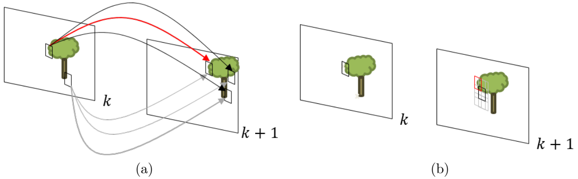
FIGURE 2.12 – Comparaison des méthodes de matching et tracking . (a) le matching compare la fenêtre descriptive d'un point d'intérêt à k à toutes les fenêtres associés aux points détectés en k+1 . (b) le tracking concentre la recherche du point en k+1 dans le voisinage de la position du point en k .
