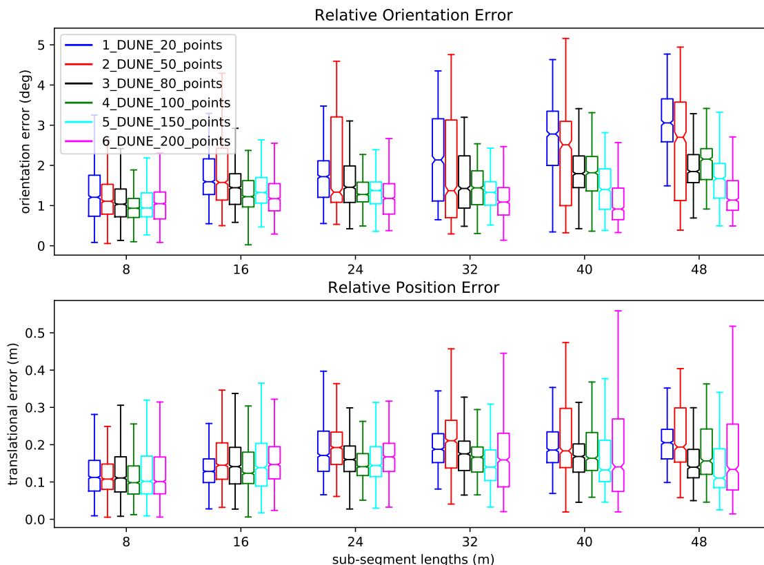
FIGURE 6.4 – Évaluation de RPE(deg/m) sur l'influence du nombre de points avec l'intégration des covariances estimées par DUNE
