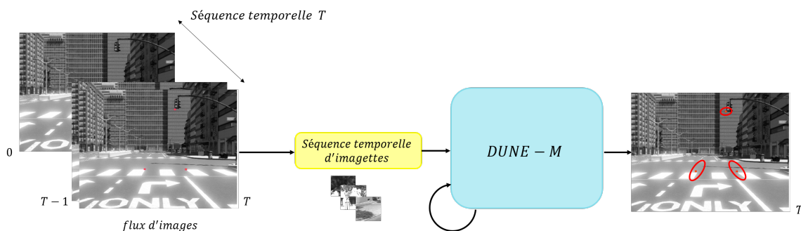
FIGURE 7.4 – Deep UNcertainty Estimation avec Mémoire (DUNE-M). Le système prend en entrée une séquence temporelle d'images (§ 4.3.2) envoyées itérativement à DUNE-M pour prédire la covariance sur la position des points d'intérêt relative à l'image finale de la séquence temporelle T .
