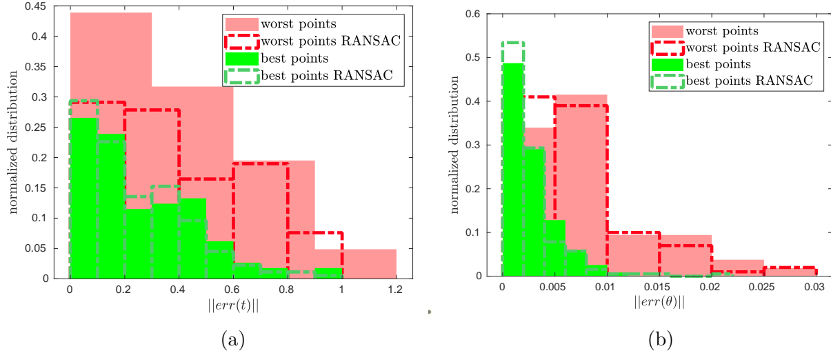
FIGURE 5.13 – Impact sur l'estimation du mouvement - (a) Erreur sur la translation (en m) ; (b) Erreur sur la rotation (en deg).
