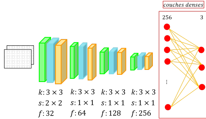
FIGURE 5.6 – Structure de l’estimateur d’incertitude sur la position des points d’intérêt DUNE - k indique la dimension des Kernels; s la dimension des strides; et f le nombre de filtres. Les couches vertes représentent les convolutions, les bleues les couches de normalisation et les jaunes les dropouts.
