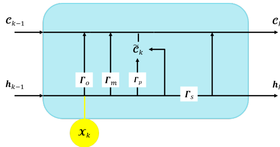
FIGURE 7.2 – Schéma bloc d'une cellule mémoire LSTM
