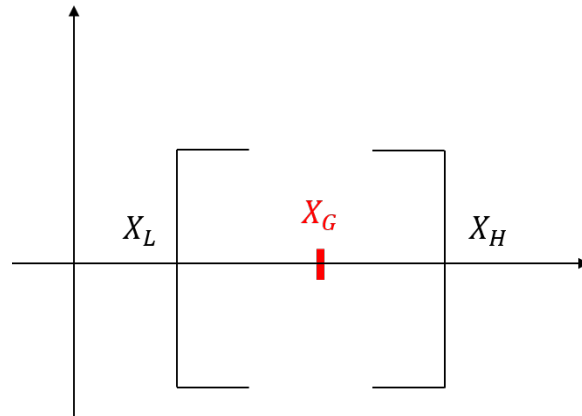
FIGURE 2.15 – Intervalle de confiance [X_L; X_H] encadrant la vérité terrain X_G
