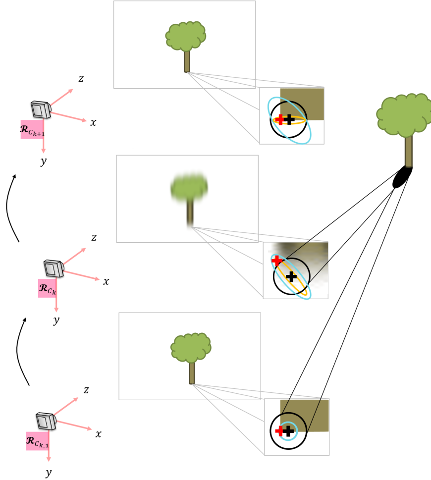
FIGURE 6.1 – Évolution de la covariance proposé par OpenVINS et DUNE entre k-1 et k+1 - + représente la vérité terrain du point d'intérêt et + le point détecté par KLT ; \mathbf{O} la covariance associée à OpenVINS fixée à 1 pixel ; \mathbf{O} la covariance sortante de DUNE \Sigma_i^{(j)} = \mathbf{R}_{i|i-1}^{(j)} et \mathbf{O} la covariance cumulée de DUNE \mathbf{R}_i^{(j)}
