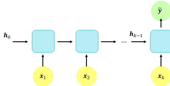
FIGURE 7.3 – Type de RNN many to one avec T_x > 1 et T_y = 1
