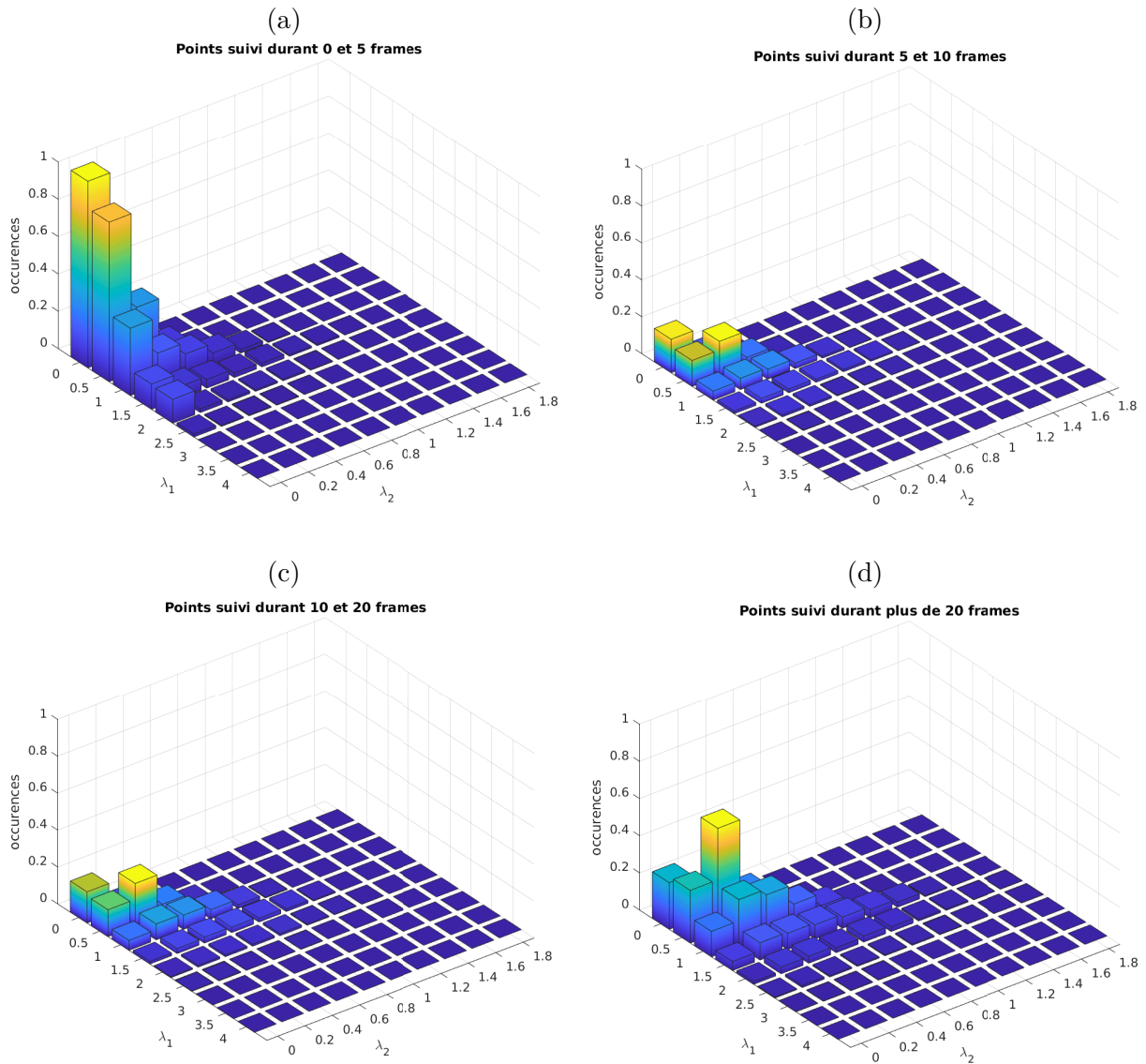
FIGURE 5.7 – Corrélation de la durée de vie du suivi d’un point d’intérêt avec les paramètres de Harris \lambda_i - (a) points suivis entre 0 et 5 images consécutives ; (b) points suivis entre 5 et 10 images consécutives ; (c) points suivis entre 10 et 20 images consécutives ; (d) points suivis sur plus de 20 images consécutives.
