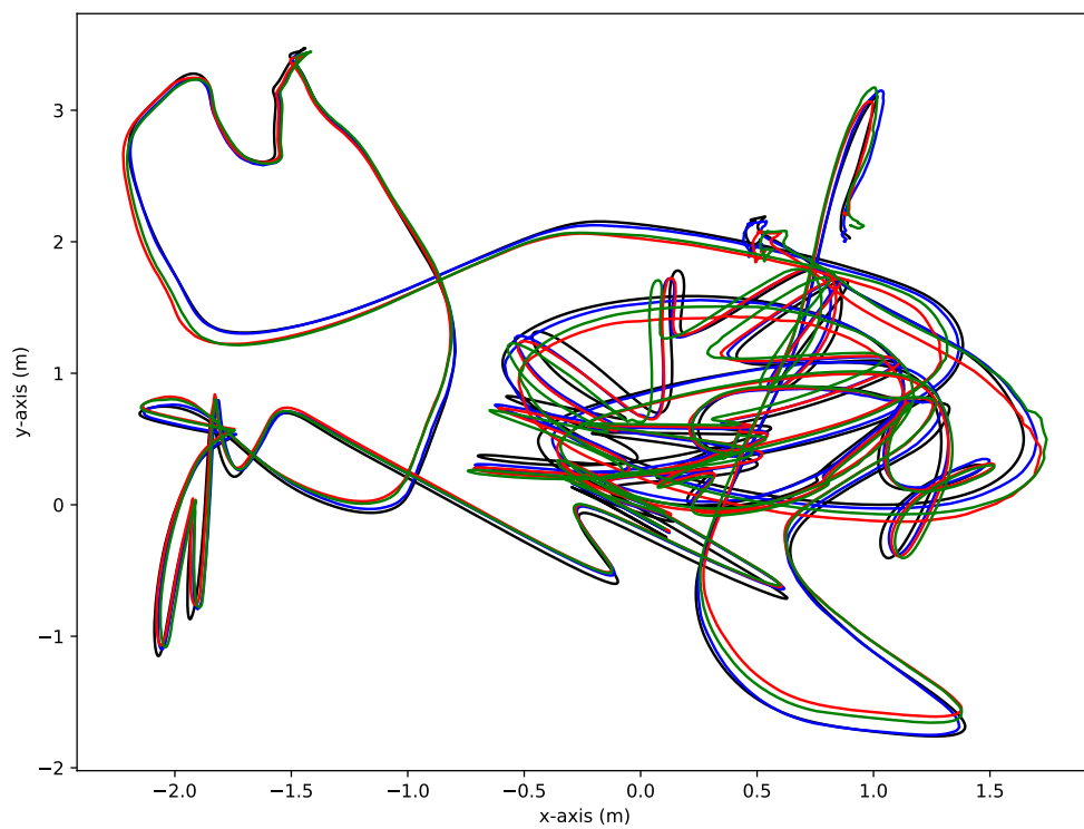
FIGURE 6.7 – Trajectoire globale du scénario V1_03_difficult - en noire la vérité terrain ; en bleu DUNE_best ; en rouge DUNE_150 et en vert OpenVINS
