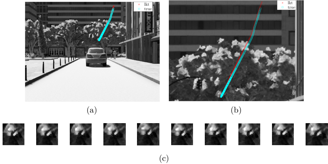
FIGURE 4.12 – Piste de tracking d’un point d’intérêt suivi au cours de X images - (a) Évolution du point dans la scène ; (b) Zoom sur la piste ; (c) Imagettes centrées sur le point suivi {}^{uv}\tilde{\mathbf{m}} observées sur les X images
