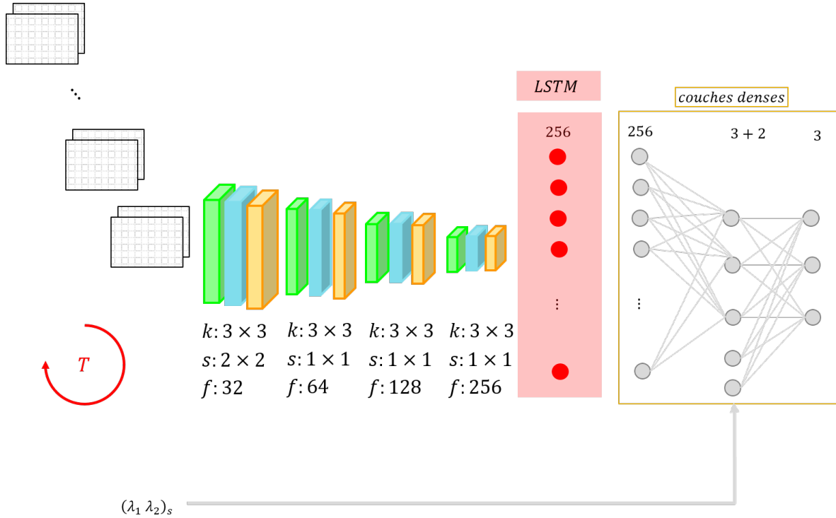
FIGURE 7.7 – Structure de l'estimateur DUNE-M d'incertitude de la position du suivi des points d'intérêt d'une séquence temporelle intégrant les paramètres de Harris (\lambda_1, \lambda_2)_i - T est la taille de la séquence temporelle, i un échantillon, k indique la dimension des Kernels; s la dimension des strides; et f le nombre de filtres. Les couches vertes représentent les convolutions, les bleues les couches de normalisation et les jaunes les dropouts. Chaque couche du RdN, à l'exception de la dernière, est suivie d'une fonction d'activation leakyrelu
