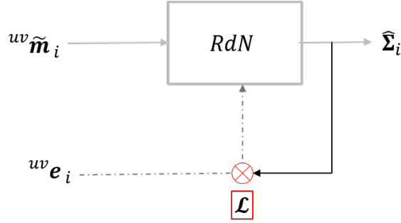
FIGURE 4.5 – RdN minimisant la fonction de coût \mathcal{L} telle que la matrice de covariance prédite \hat{\Sigma}_i associée au point d'intérêt {}^{uv}\mathbf{m}_i maximise la probabilité d'obtenir l'erreur {}^{uv}\mathbf{e}_i .
