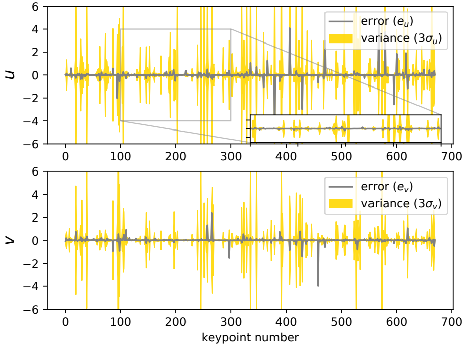
FIGURE 5.15 – Évolution de l'incertitude sur la position des points d'intérêt prédite par DUNE et comparaison à l'erreur de tracking.
