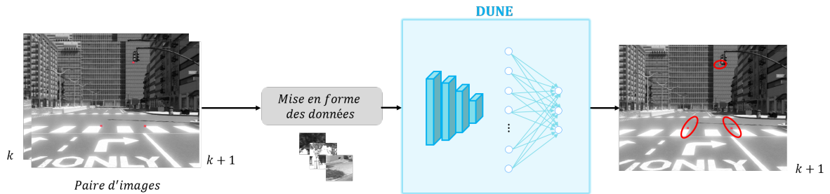
FIGURE 5.3 – Deep UNcertainty Estimation (DUNE) pipeline. Le système prend en entrée une paire d'images, sur laquelle des points d'intérêt sont suivis. L'information est par la suite traitée (§ 4.3) afin d'extraire des imagettes centrées sur la position des points estimée par KLT. Ces imagettes sont fournies au RdN DUNE qui estime les matrices de covariance de chacun des points d'intérêt suivis.
