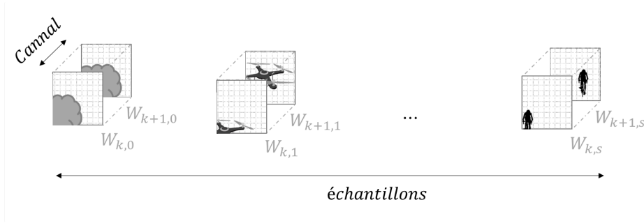
FIGURE 5.4 – Format des données - concaténation des fenêtres centrées en {}^{uv}\tilde{\mathbf{m}}_k et {}^{uv}\tilde{\mathbf{m}}_{k+1} . L'ensemble des échantillons s constituent le jeu de données \mathcal{D} .
