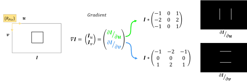
FIGURE 2.10 – Exemple d'application d'un filtre de Sobel sur l'image I
