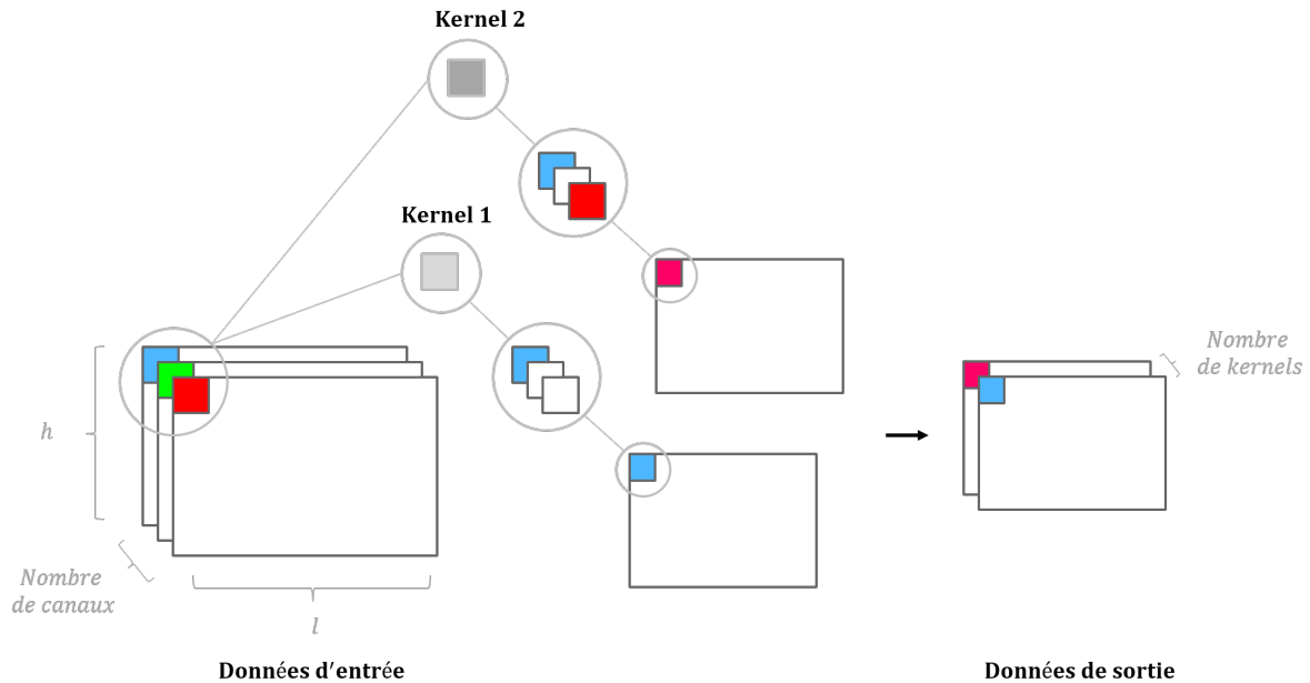
FIGURE 5.1 – Illustration du principe de fonctionnement d’un CNN, avec en entrée une image RVB convolutionnée avec deux filtres de Kernel de dimension 1 pixel. Le premier kernel filtre le rouge et le vert produisant un pixel bleu, le second kernel filtre uniquement le vert et aboutit en un pixel rose. L’image résultante est le résultat de chaque convolution concaténée.
