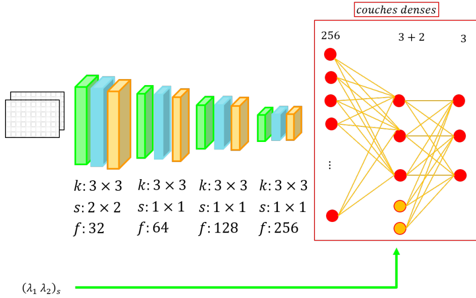
FIGURE 5.9 – Structure de l’estimateur d’incertitude sur la position des points d’intérêt DUNE intégrant les paramètres de Harris (\lambda_1, \lambda_2) - k indique la dimension des Kernels; s la dimension des strides; et f le nombre de filtres. Les couches vertes représentent les convolutions, les bleues les couches de normalisation et les jaunes les dropouts.
