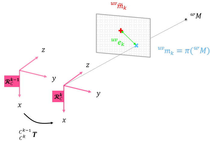
FIGURE 2.18 – Définition de l’erreur représentée par la distance verte entre le point estimé {}^{uv}\tilde{\mathbf{m}}_k en rouge et la vérité terrain {}^{uv}\mathbf{m}_k en bleu, entre deux images consécutives \mathcal{R}_C^{k-1} et \mathcal{R}_C^k
