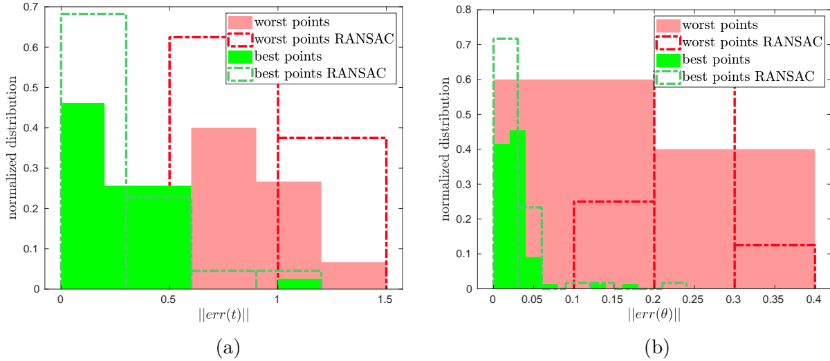
FIGURE 7.12 – Impact sur l'estimation du mouvement - (a) Erreur sur la translation (en m) ; (b) Erreur sur la rotation (en deg).
