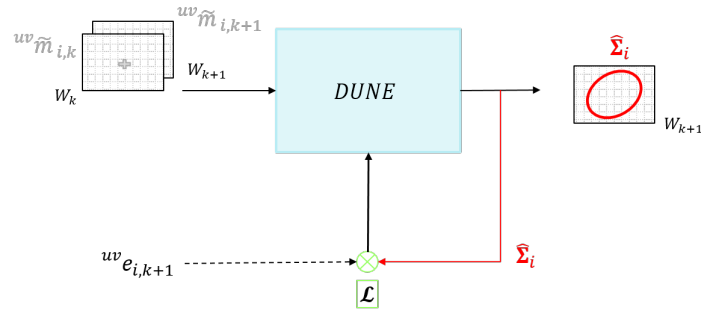
FIGURE 5.5 – Ajustement du réseau de neurones DUNE pendant la phase d’apprentissage - DUNE prend en entrée un échantillon i de deux imageries concaténées [^{uv}\mathbf{W}_k; ^{uv}\mathbf{W}_{k+1}]_i centrées en ^{uv}\tilde{\mathbf{m}}_k et ^{uv}\tilde{\mathbf{m}}_{k+1} , et prédit la matrice de covariance \tilde{\Sigma}_i associée à ^{uv}\mathbf{W}_{k+1,i} . La fonction de coût appliquée \mathcal{L} compare l’erreur mesurée à k + 1 ^{uv}e_{i,k+1} avec la matrice de covariance prédite \tilde{\Sigma}_i
