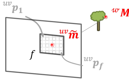
FIGURE 2.13 – Fenêtre f centrée en {}^{uv}\tilde{m} la position du point tracké par KLT issue de {}^wM . Les points autour de {}^{uv}\tilde{m} contenus dans f sont notés de {}^{uv}p_1 à {}^{uv}p_f, f \in \mathbb{N}
