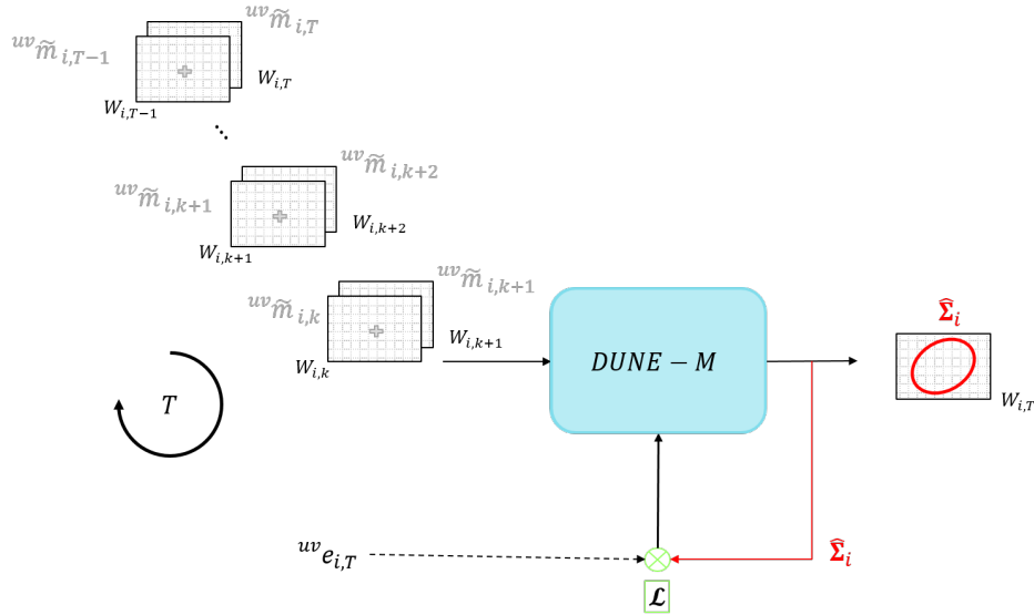
FIGURE 7.6 – Ajustement des poids du RNN DUNE-M pendant la phase d'apprentissage - DUNE-M prend en entrée un échantillon i décrit par une séquence d'imagettes concaténées [{}^{uv}\mathbf{W}_{i,k}; {}^{uv}\mathbf{W}_{i,k+1}] centrées en {}^{uv}\tilde{\mathbf{m}}_{i,k} et {}^{uv}\tilde{\mathbf{m}}_{i,k+1} \forall k \in \llbracket 0; T \rrbracket , et prédit la matrice de covariance \tilde{\Sigma}_i associée à {}^{uv}\mathbf{W}_{i,T} . La fonction de coût appliquée \mathcal{L} compare l'erreur mesurée à T {}^{uv}\mathbf{e}_{i,T} avec la matrice de covariance prédite \tilde{\Sigma}_i
