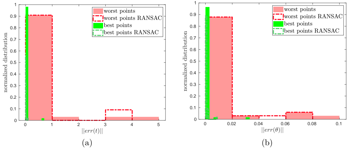
FIGURE 5.16 – Impact sur l'estimation du mouvement - (a) Erreur sur la translation (en m) ; (b) Erreur sur la rotation (en deg).
