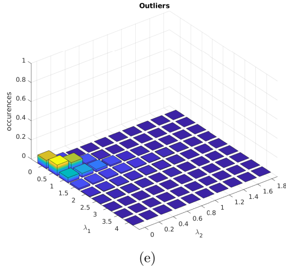
FIGURE 5.8 – Corrélation de la durée de vie du suivi d’un point d’intérêt avec les paramètres de Harris \lambda_i pour les points non suivis ou outliers
