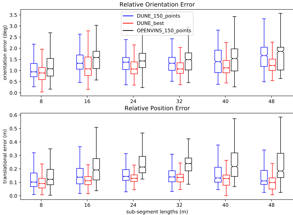
FIGURE 6.6 – Évolution de l’erreur RPE pour la sélection des meilleurs points
