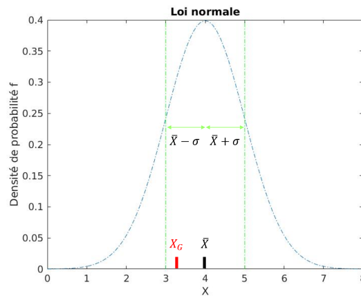
FIGURE 2.16 – Densité de probabilité f de la variable aléatoire X centré en \bar{X}
