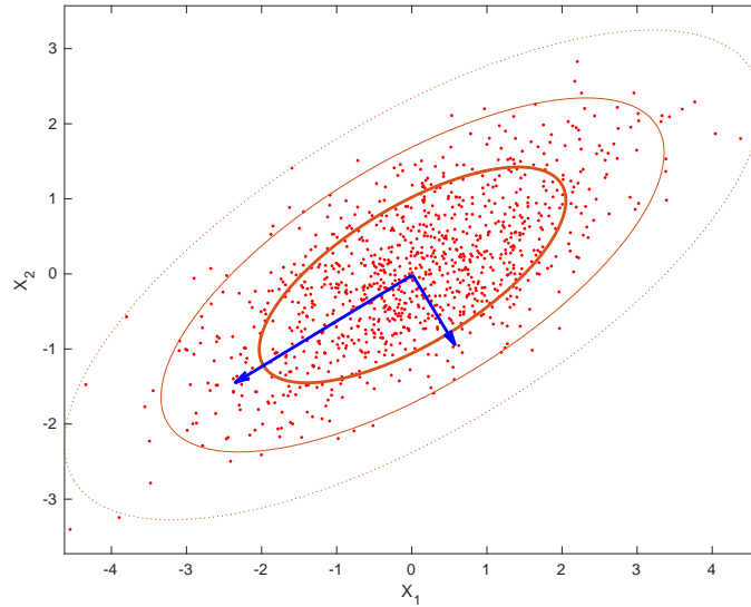
FIGURE 2.17 – Représentation des ellipses à 1\sigma , 2\sigma et 3\sigma d'une covariance bidimensionnelle issue d'une loi normale multivariée
