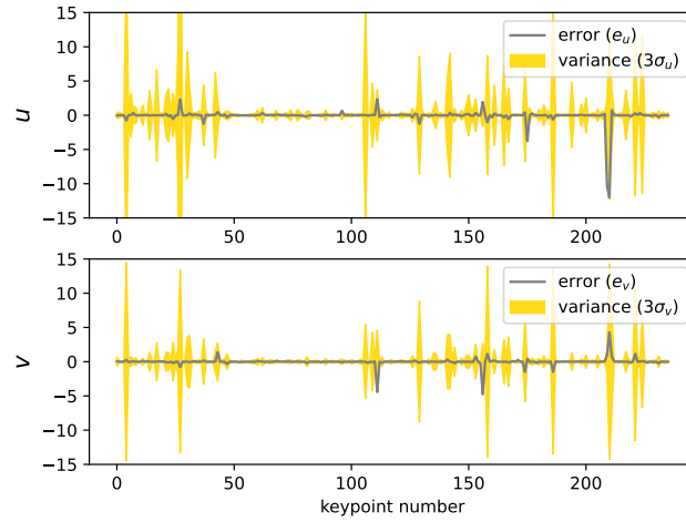
FIGURE 7.9 – Évolution de l'incertitude sur la position des points d'intérêt prédite par DUNE et comparaison à l'erreur de tracking.
