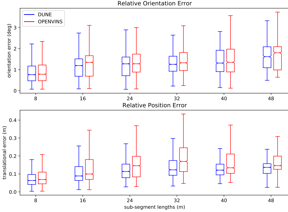
FIGURE 6.5 – Évolution de l’erreur moyenne RPE sur des segments de trajectoire.
