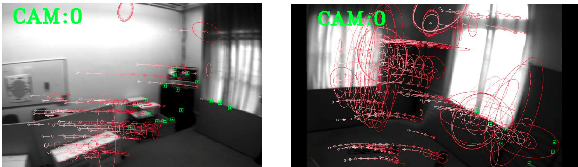
FIGURE 6.2 – Affichage des pistes d'évolution des matrices de covariance issues de DUNE appliquées à un système monoculaire sur deux points de vue d'un scénario Euroc [Bur+16] - Les ellipses sont augmentées d'un facteur 10 à des fins de visualisation
