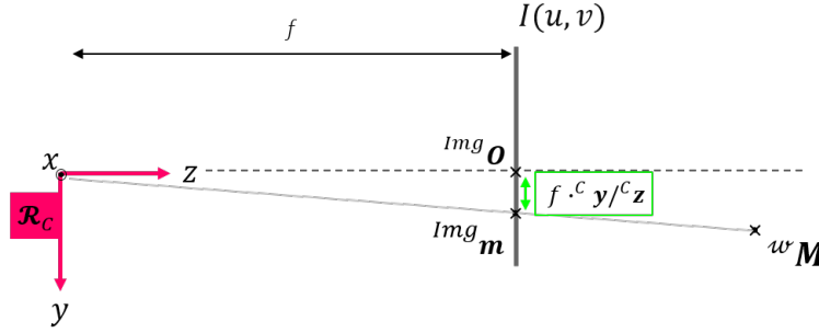
FIGURE 2.5 – Projection d'un point {}^w\mathbf{M} sur le plan image
