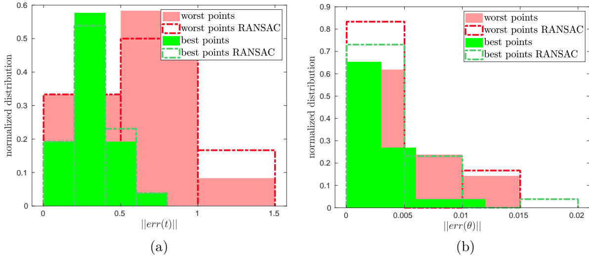
FIGURE 7.10 – Impact sur l'estimation du mouvement - (a) Erreur sur la translation (en m) ; (b) Erreur sur la rotation (en deg).
