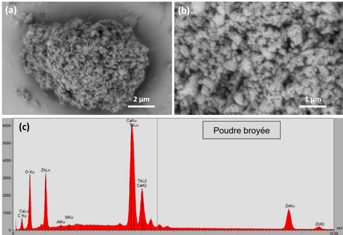
Figure III-15 : (a et b) Images MEB réalisées en électrons rétrodiffusés sur la poudre broyée BP-10mm-10min + BP-0,5mm-4min (avec métallisation au platine), avec deux grossissements différents.
