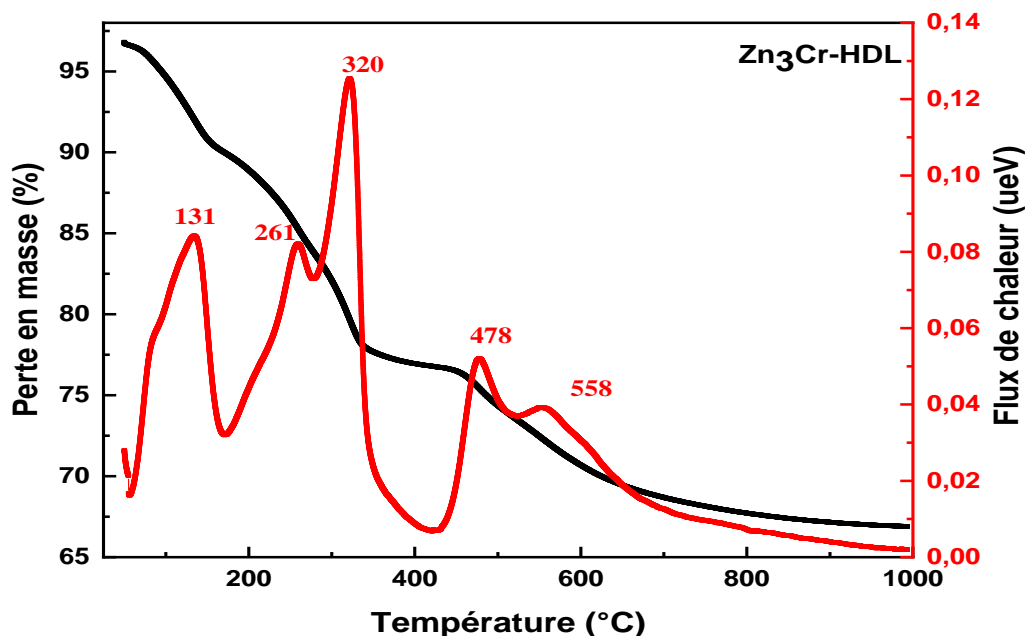
Figure 4.1. Thermogrammes ATG-ATD de l'échantillon Zn 3 Cr-HDL, réalisées sous air.
