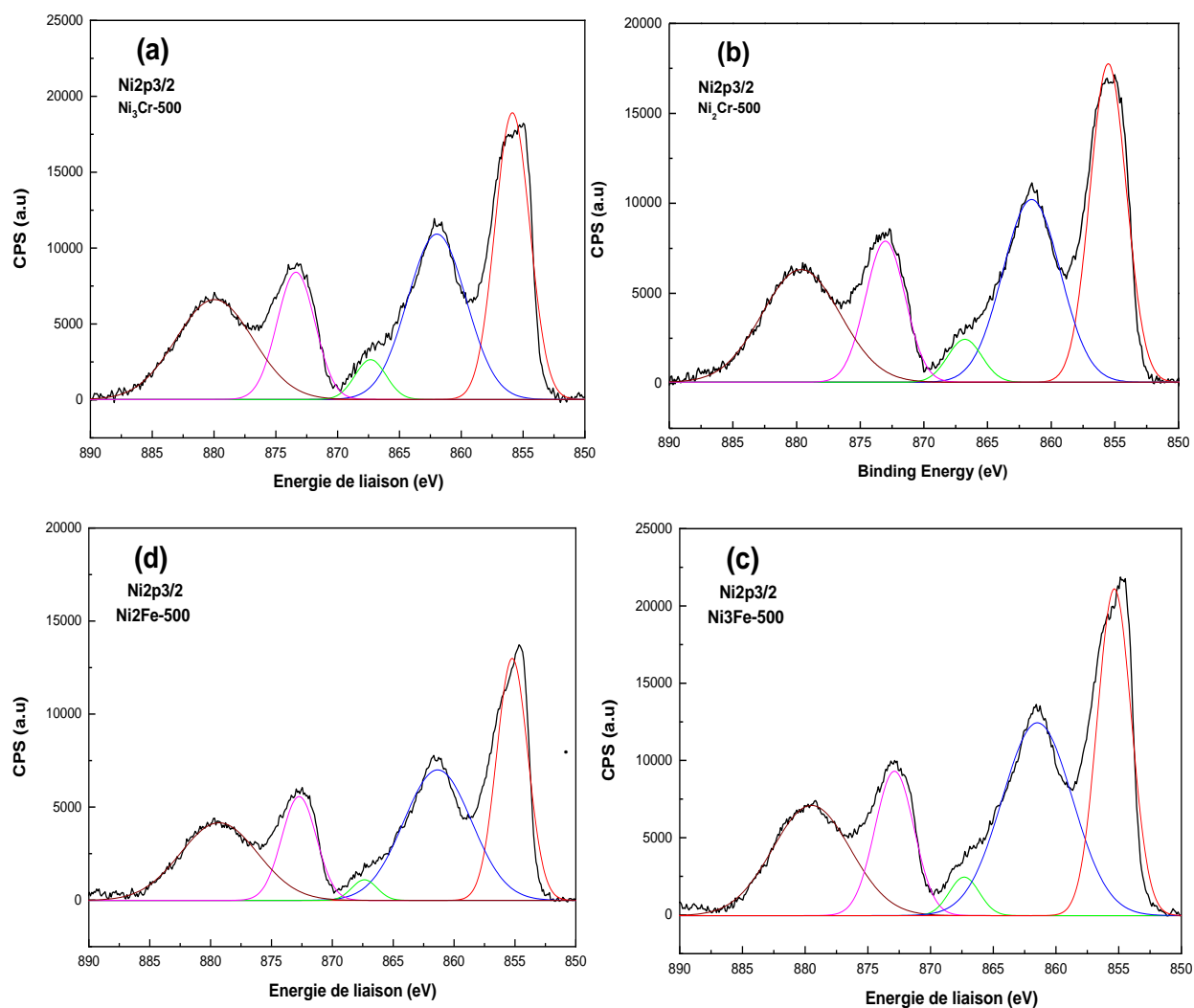
Figure 3.15. Spectres XPS de la raie Ni 2p 3/2 des catalyseurs Ni 2 Fe, Ni 3 Fe, Ni 2 Cr et Ni 3 Cr calcinés à 500 °C.
