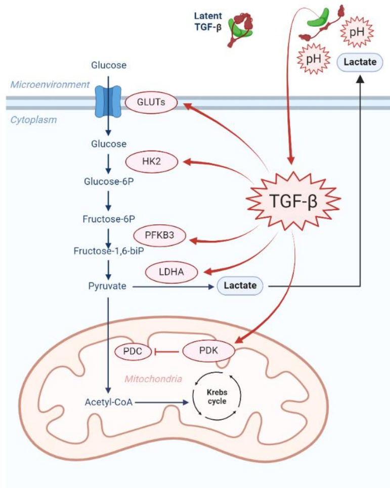
Figure 14 : Stimulation du métabolisme glycolytique par le TGF-β. Le TGF-β induit l'expression de plusieurs enzymes glycolytiques qui entraînent une forte production et sécrétion de lactates. L'acidification engendrée active le TGF-β latent en dénaturant le complexe LAP (Latent associated protein). GLUTs : Glucose transporters ; HK2 : Hexokinase-2 ; LDHA : lactate déshydrogénase A ; PFKB3 : 6-Phosphofructo-2-Kinase/Fructose-2,6-Biphosphatase 3 ; PDC : Pyruvate Dehydrogenase Complex ; PDK : Pyruvate dehydrogenase kinase. Par Tom Voisin, Biorender.
