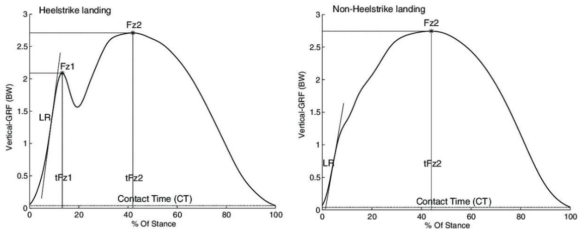
Figure 16 - Courbe représentative de la force verticale moyenne développée par un participant lors d'une course à allure sous-maximale pour un coureur à attaque talon (gauche) et un coureur à attaque médio-pied (d'après Kluitenberg et al., 2012). BW : poids de corps , Fz1 = pic passif, Fz2 = pic actif, LR = taux de charge
