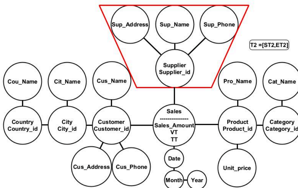
FIGURE 4.2 – Schéma logique de GAMM( t_2 )
