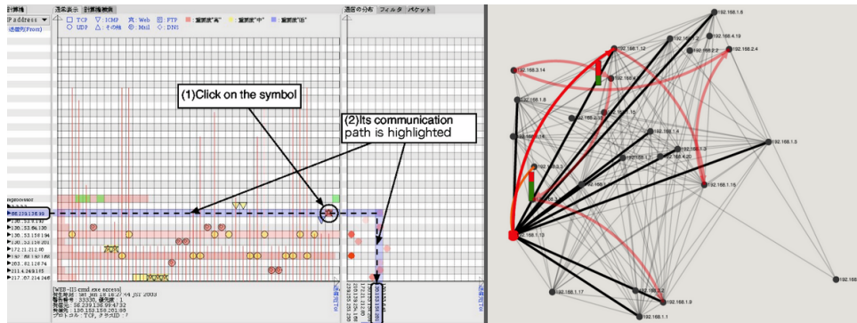
FIGURE 2.16 – Exemples de superposition. À gauche, Snortview [56] (2004, ©ACM) superpose les chemins d'accès avec les alertes sur une représentation matricielle. À droite, Percival [57] (2015, ©IEEE) superpose les chemins d'attaques et les contre-mesures disponibles sur un diagramme nœuds/liens .
