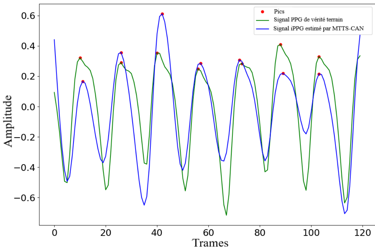
FIGURE 4.5 – Comparaison entre un signal prédit par MTTTS-CAN et le signal PPG correspondant de vérité terrain tiré de la base de données BP4D+.
