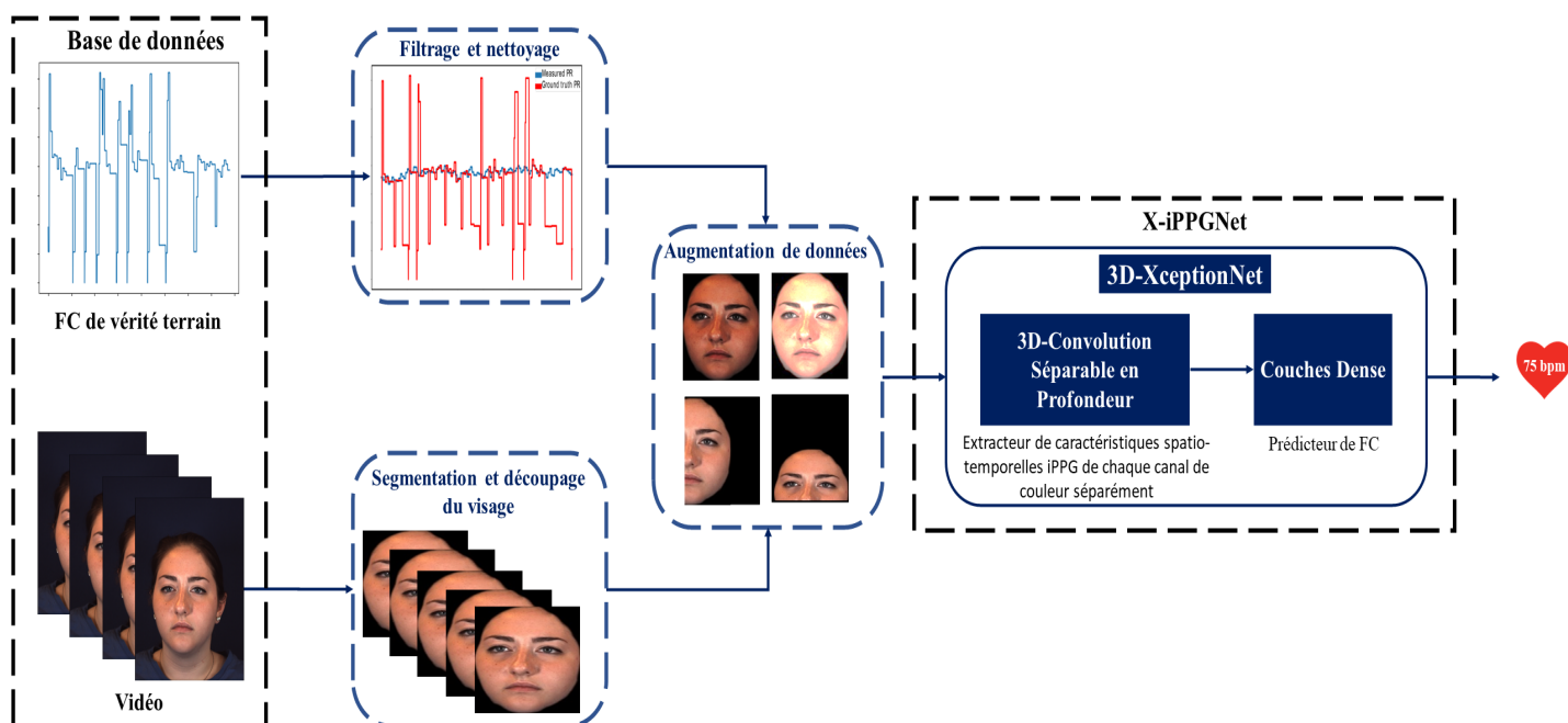
FIGURE 3.4 – Aperçu du système proposé pour l’estimation sans contact de la fréquence cardiaque instantanée. Une segmentation et un découpage du visage sont d’abord effectués sur les vidéos d’entrée pour éliminer les zones ne contenant pas de peau. Les signaux de fréquence cardiaque sont filtrés et nettoyés pour éliminer les données corrompues afin d’entraîner correctement le réseau de neurones (cf. sous-section 3.2.4). Les séquences d’images faciales sont ensuite introduites à un réseau de neurones profond (X-iPPGNet) composé de convolutions séparables en profondeur 3D pour l’extraction des caractéristiques spatiales et temporelles, et de couches denses pour la prédiction de la fréquence cardiaque.
