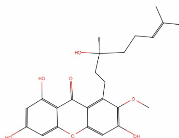
parvixanthone G (10)
