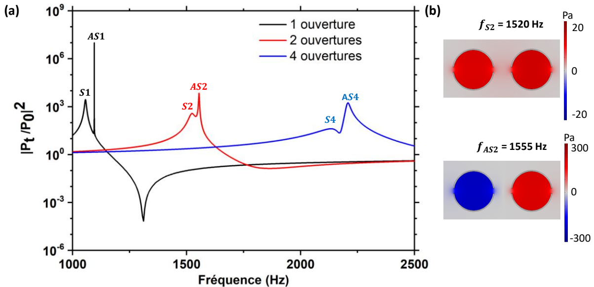
Figure II.2.5 (a) Évolution du module carré de la pression totale normalisée au point D en fonction de la fréquence pour des HR jumeaux face à face ( d = 10 mm) avec une, deux et quatre ouvertures. L'angle d'incidence est \theta = 0^\circ . (b) Distribution de la partie réelle de la pression totale pour le premier pic à f_{S_2} = 1520 Hz (haut) et le second pic à f_{AS_2} = 1555 Hz (bas).
