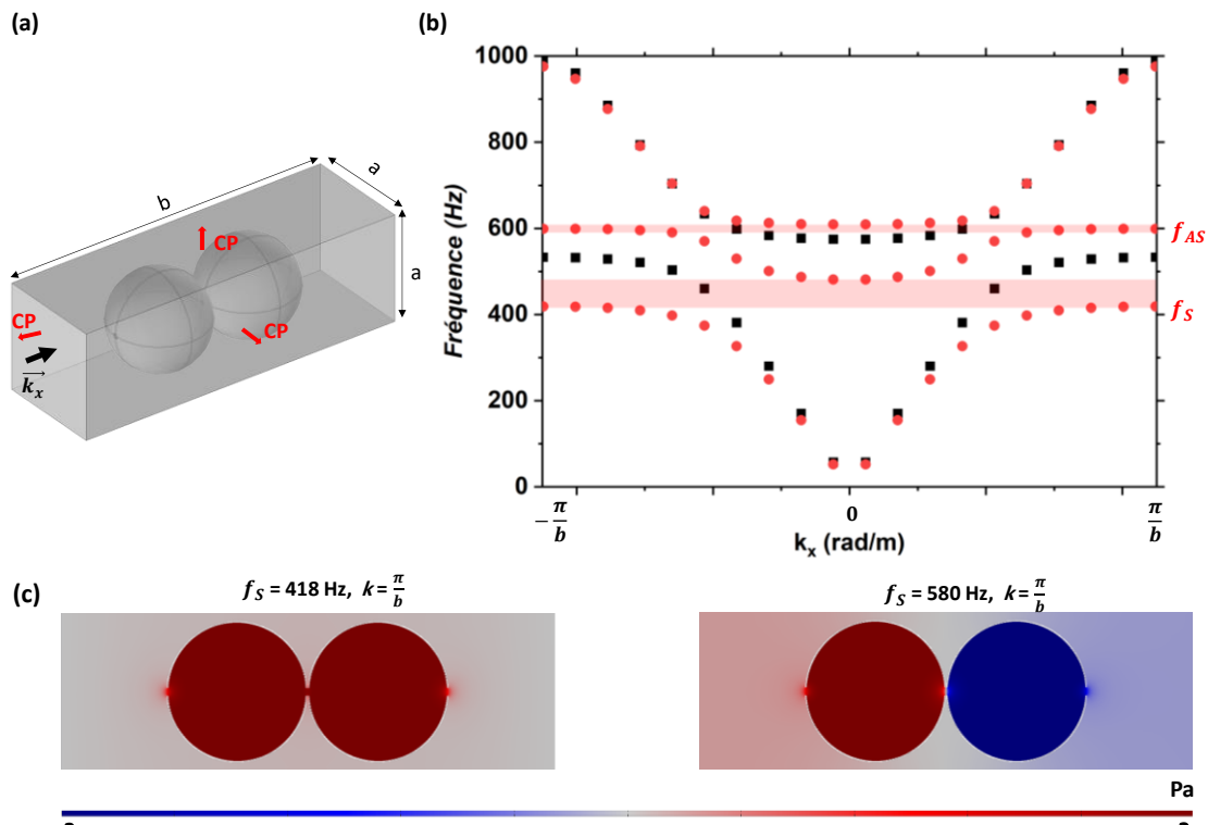
Figure IV.2.7 (a) Maille élémentaire contenant deux résonateurs, chacun percé en entrée et en sortie selon l'axe x . (b) Courbe de dispersion d'un réseau 3D d'une (noir) et deux (rouge) métasurfaces de paramètre de maille a = 4.5 cm avec b = 14 cm, et (b) et (b) les cartes de champ correspondantes aux fréquences f_S et f_{AS} pour k = \frac{\pi}{b} .
