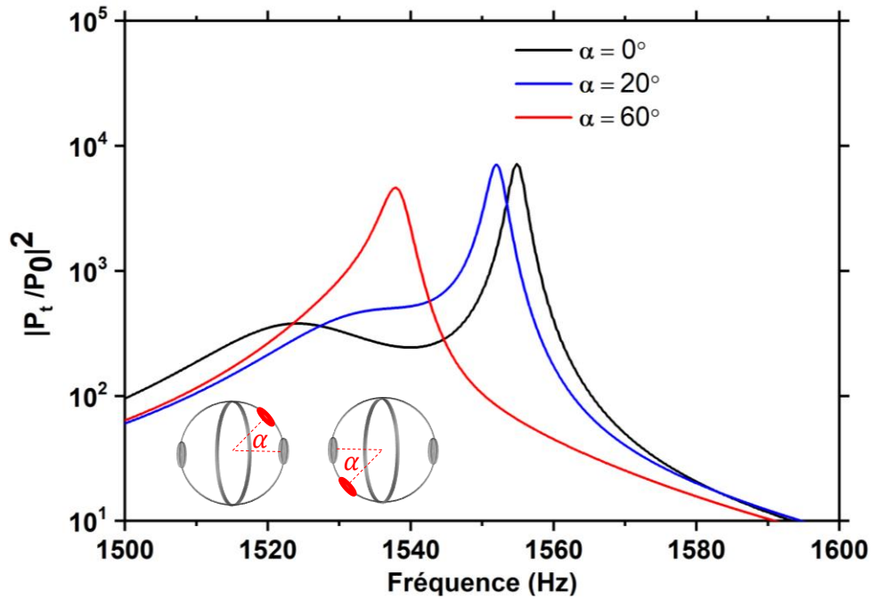
Figure II.2.9 Evolution du module carré de la pression totale normalisée en fonction de la fréquence pour des HR jumeaux à deux ouvertures, en faisant varier l'orientation des ouvertures face à face par \alpha (encart).
