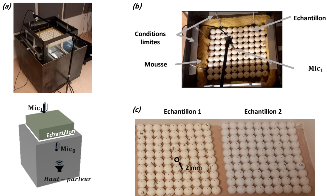
Figure V.1.1 (a) Photo de la boîte de réverbération (haut) et représentation schématique (bas), montrant le haut-parleur, la métasurface, le microphone intérieur ( Mic_1 ) et extérieur ( Mic_0 ). (b) Photo de l'installation depuis le haut montrant la mousse, la métasurface et le microphone extérieur ( Mic_1 ). (c) Matrices de balles de ping-pong ( 10 \times 9 ) percées d'un trou (échantillon 1) et de cinq trous (échantillon 2) d'un rayon de 2 mm.
