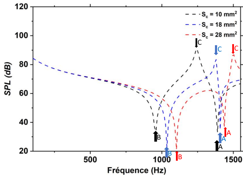
Figure V.2.12 Evolution du SPL à travers une métasurface de balles à 5 trous déposée sur une plaque en plexiglas rigide sans pertes thermo-visqueuses avec une surface de contact S_c de 10 \text{ mm}^2 (noire), 18 \text{ mm}^2 (bleue) et 28 \text{ mm}^2 (rouge). Le rayon du trou est de 2 mm et l'onde incidente est envoyée sous incidence normale sur la plaque de plexiglas avec un SPL = 91 dB.
