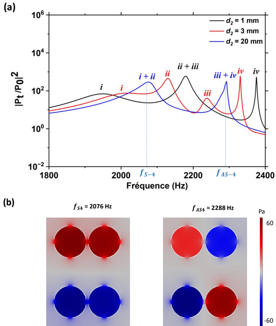
Figure II.2.12 (a) Evolution du module carré de la pression totale normalisée en fonction de la fréquence sous incidence 45° avec changement de la distance d_2 de 1 mm (noir), 3 mm (rouge) et 20 mm (bleu).
