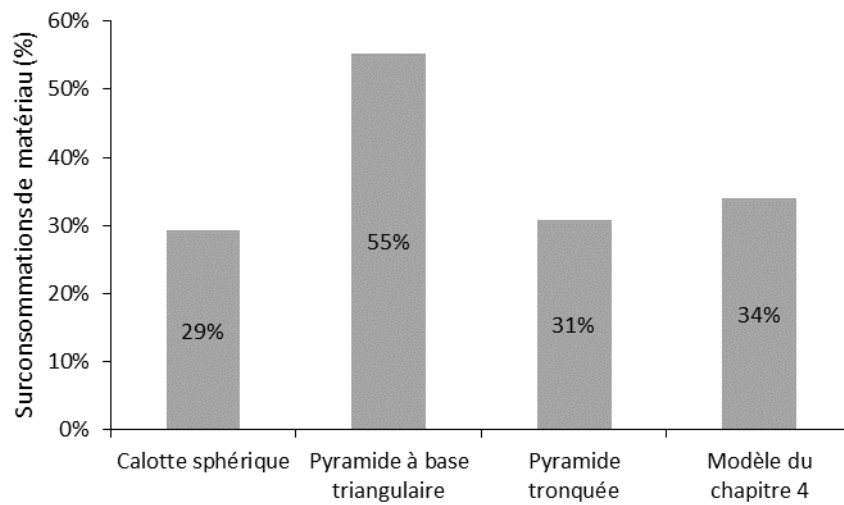
Figure 108 : Surconsommations de matériau calculées pour les différentes géométries étudiées.
