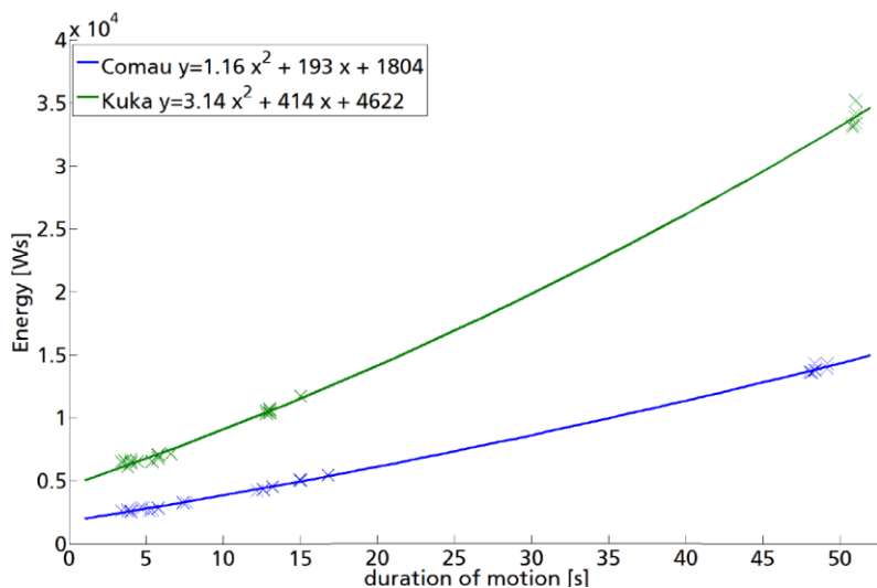
Figure 46 : Consommation d'énergie des bras robot pour réaliser un mouvement en fonction de la durée du mouvement [77].
