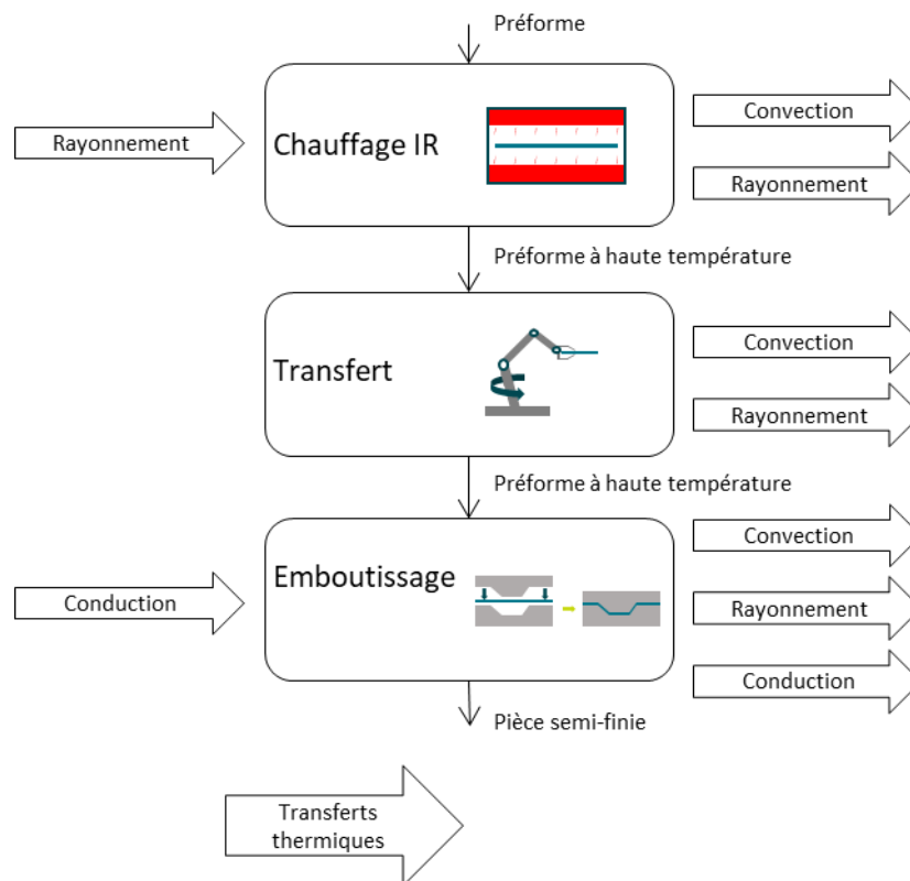
Figure 81 : Description du procédé de thermoformage-estampage et des transferts thermiques mis en jeux et modélisés.
