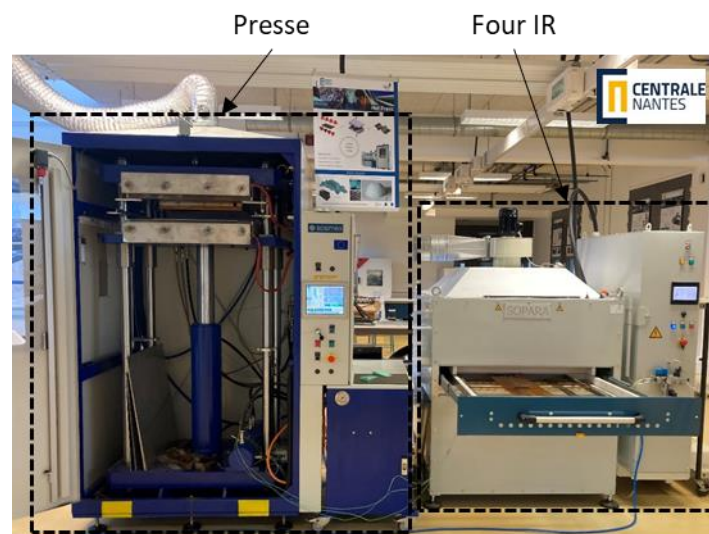
Figure 19 : Cellule de thermoformage-estampage de l'école Centrale de Nantes : Four IR SOPARA utilisé pour l'étape de chauffage et Presse SCAMEX de 75T utilisée pour l'étape d'emboutissage.
