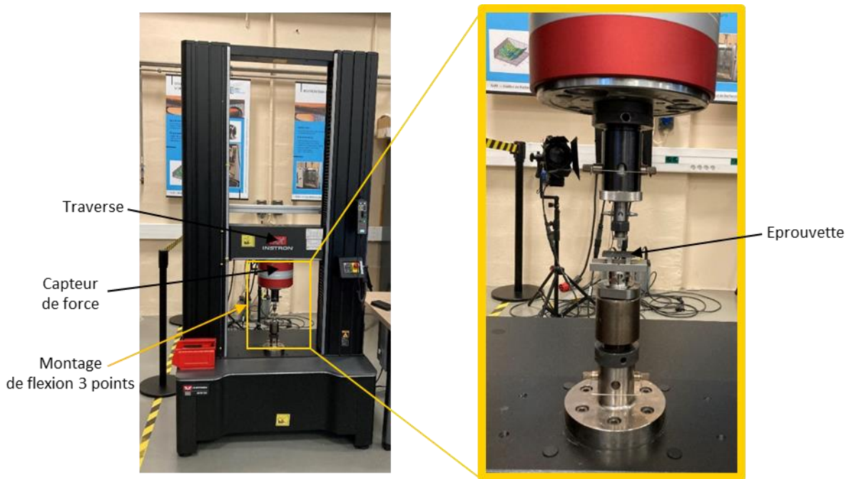
Figure 23 : Machine de traction-compression Instron 68FM - 300 équipée du montage de flexion trois points utilisés.
