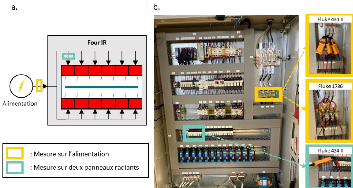
Figure 38 : Montage expérimental utilisé pour les relevés électriques sur le four IR : a. Représentation schématique des différents points de mesure ; b. Tableau électrique du four IR et emplacement des mesures électriques réalisées sur l'alimentation générale avec le Fluke 434 II (pinces i30s) et le Fluke 1736 (pinces iFlex 1500-12) ainsi que sur l'alimentation de deux panneaux radiants avec le Fluke 434 II (pinces i30s).
