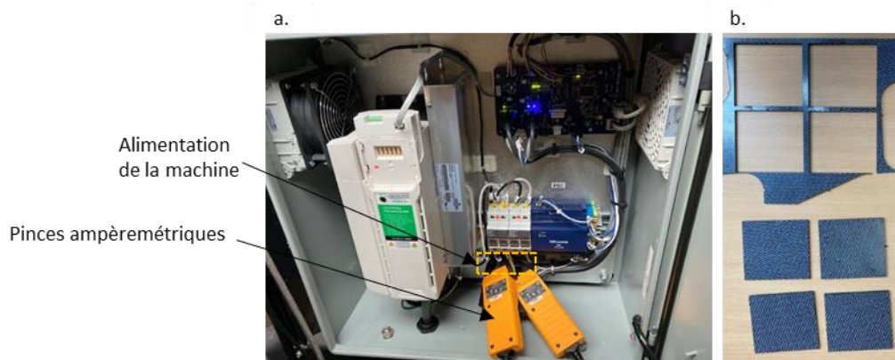
Figure 36 : a. Montage électrique pour les relevés de puissance active consommée par la machine de découpe jet d'eau ; b. Découpes réalisées lors des relevés électriques sur la machine de découpe jet d'eau.
