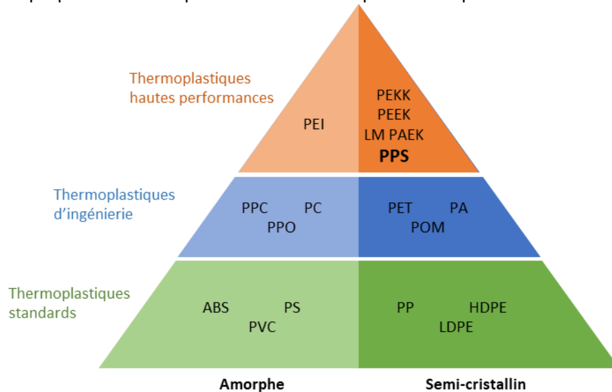
Figure 11 : Principales résines thermoplastiques utilisées dans les composites [13].
