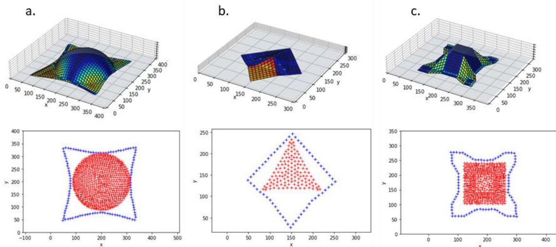
Figure 107 : Résultats de l'application de la procédure d'identification de la préforme minimale permettant de produire les pièces étudiées : a. Calotte sphérique ; b. Pyramide à base triangulaire ; c. Pyramide à base carrée tronquée.
