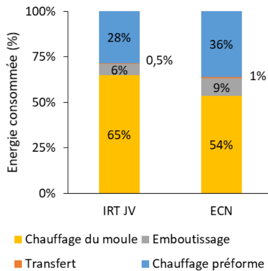
Figure 62 : Comparaison des consommations d'énergie électrique des procédés du laboratoire et de l'IRT Jules Verne pour la transformation d'1kg de matériau.
