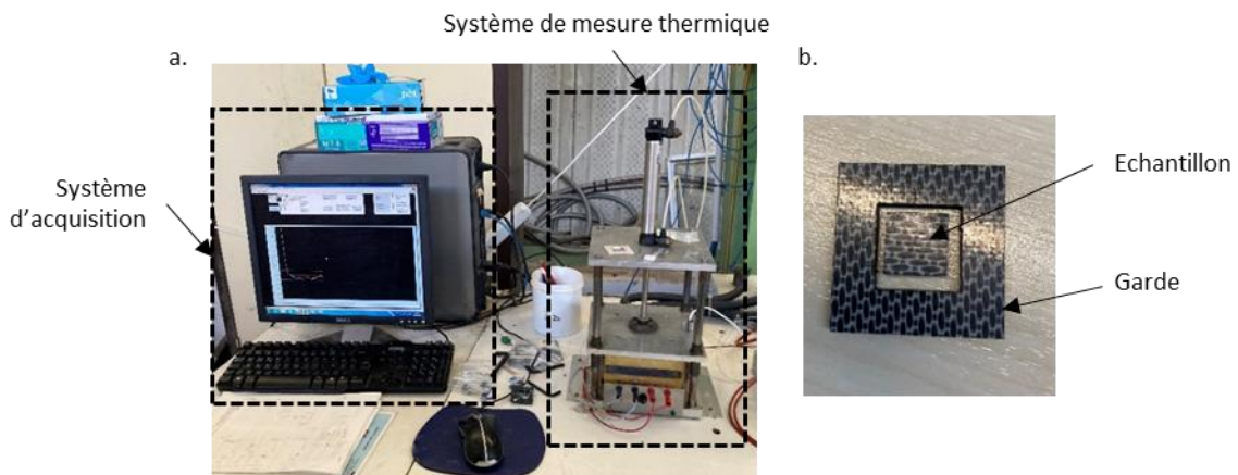
Figure 88 : a. Montage expérimental pour les essais de plaque chaude gardée ; b. Eprouvette de plaque chaude gardée.
