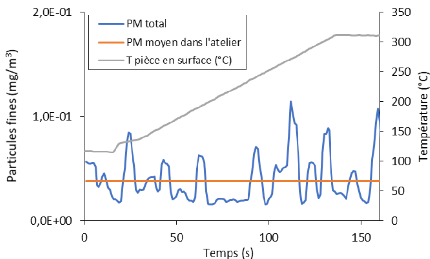
Figure 52 : Exemple de résultat des mesures d'émissions de particules fines totales lors d'un essai de chauffage dans le four IR à 100% de la puissance de chauffage.
