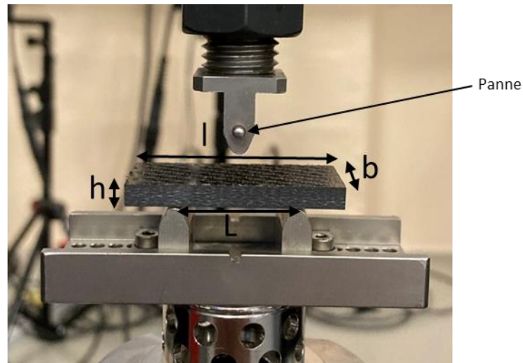
Figure 24 : Banc de flexion trois points utilisé.
