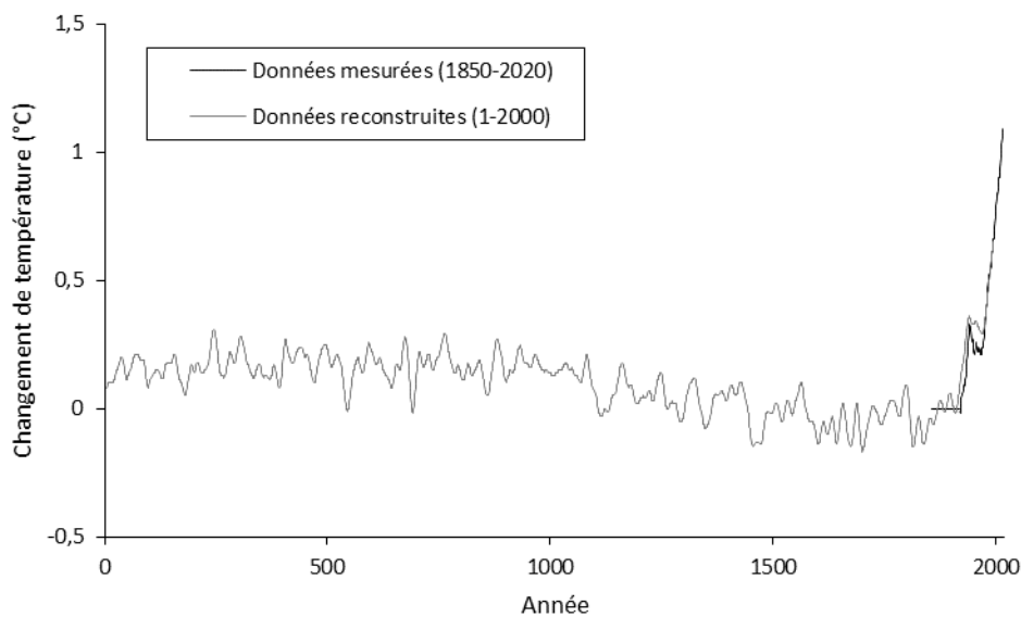
Figure 1 : Evolution de la température (moyenne décennale) à la surface du globe [2].
