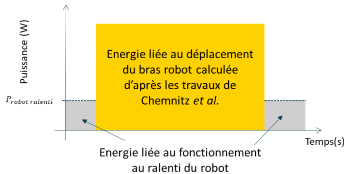
Figure 47 : Modèle proposé pour la consommation d'énergie électrique du bras robot d'après les travaux de Chemnitz et al. [77].
