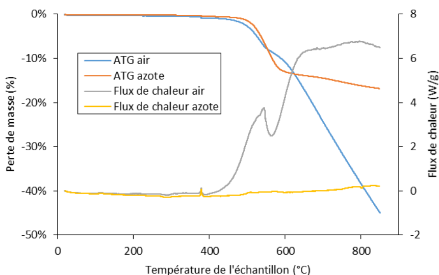
Figure 53 : Résultats des mesures ATG et DSC des essais 2 (sous air) et 4 (sous N 2 ).
