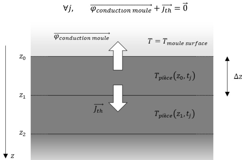
Figure 86 : Condition d'équilibre des flux thermiques à l'interface moule-pièce lors de l'étape d'emboutissage.
