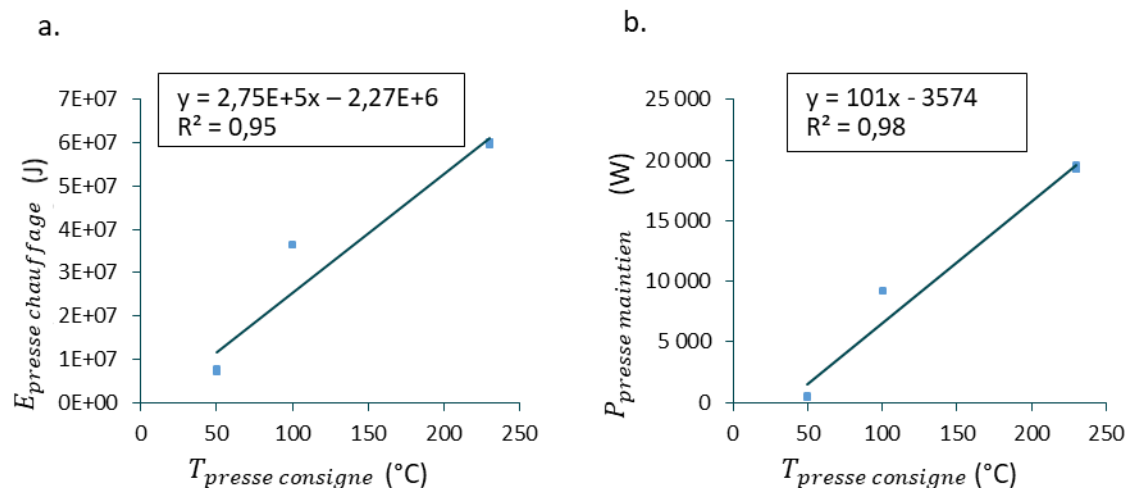
Figure 51 : Modélisation linéaire des coefficients du modèle de consommation électrique du système thermique de la presse en fonction de la température de consigne des plateaux chauffants T_{\text{presse consigne}} :
