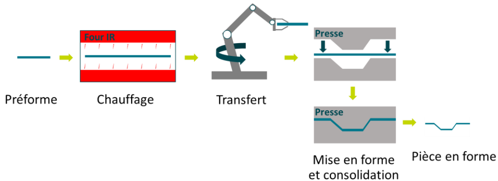
Figure 13 : Procédé de thermoformage-estampage.
