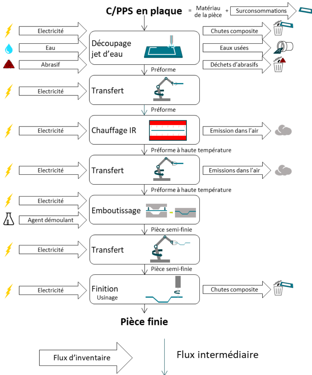
Figure 20 : Arbre des processus du procédé de thermoformage-estampage de C/PPS.
