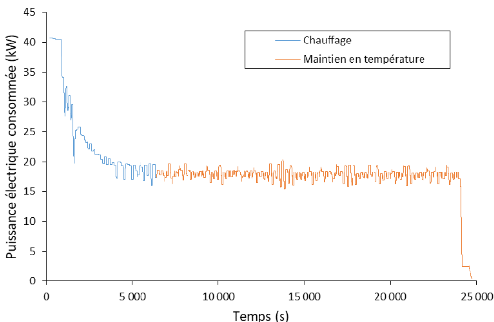
Figure 60 : Exemple de relevé de puissance électrique consommée par le thermorégulateur TT-388 Z lors de la mise en œuvre du procédé de l'IRT Jules Verne.
