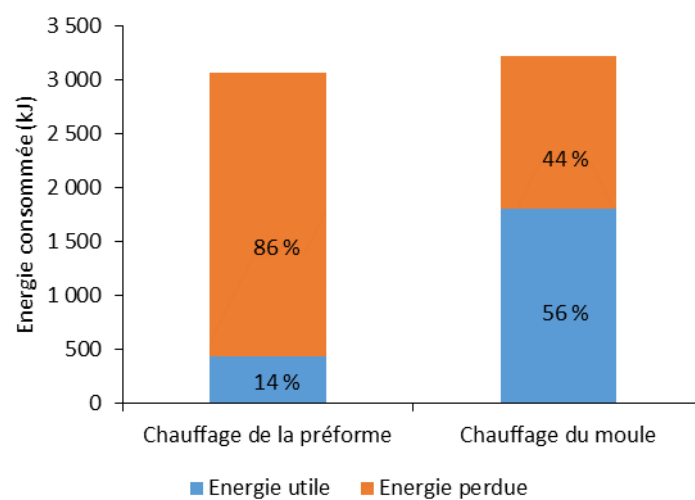
Figure 98 : Résultats de l'exploitation du modèle thermique et des données mesurées pour l'identification du potentiel de diminution de consommation d'énergie du procédé de thermoformage-estampage.
