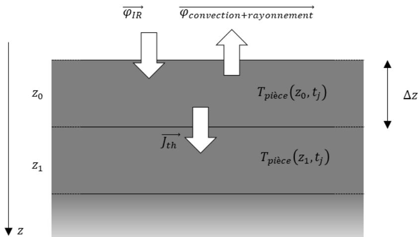
Figure 84 : Condition d'équilibre des flux thermiques sur la surface supérieure de la préforme lors de l'étape de chauffage infrarouge.
