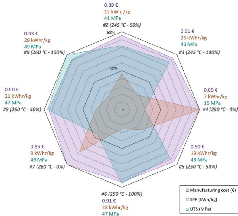
Figure 14 : Représentation sur un diagramme radar des résultats économiques, mécaniques et énergétiques des différentes configurations de paramètres testés pour aider à la décision [52].
