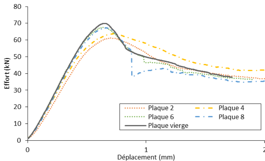
Figure 25 : Exemple de résultats d'essais de flexion pour des éprouvettes prises dans les plaques n°2, 4, 6, 8 et dans le matériau vierge.
