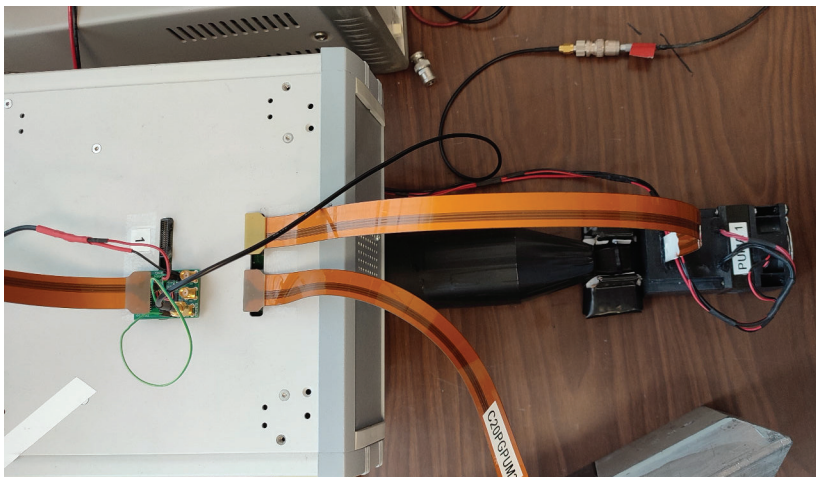
FIGURE 3.34 – Dispositif expérimental utilisé en laboratoire pour l'évaluation de la résolution en coïncidence temporelle (CTR) du système entre le signal externe du LaBr 3 et un module PUMA.
