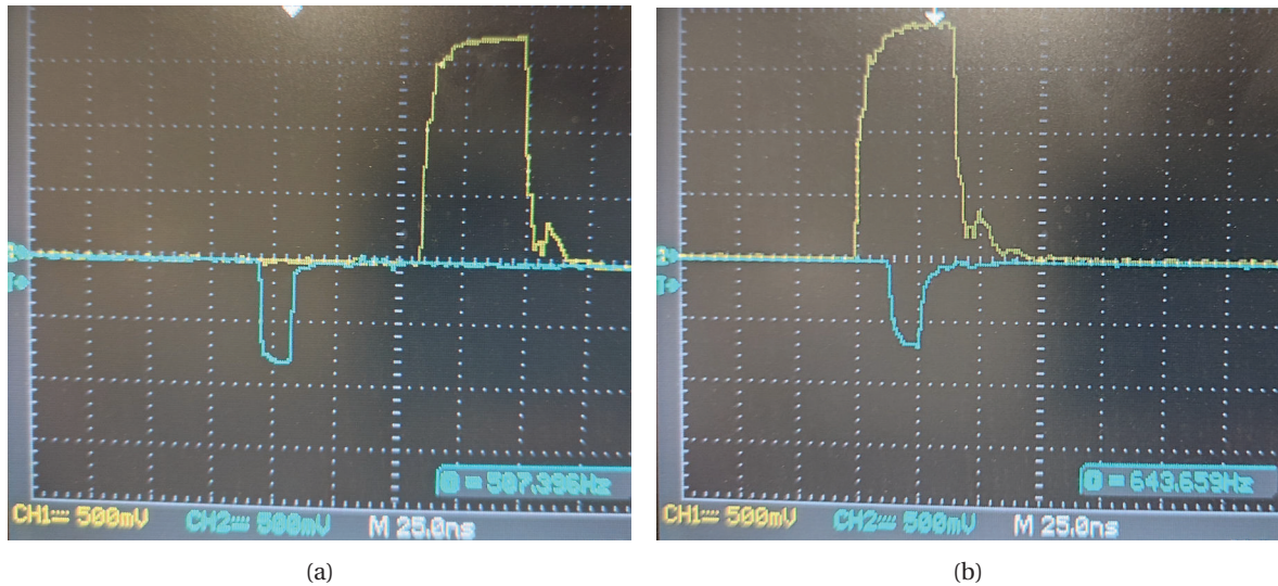
FIGURE 3.35 – Différences temporelles entre le signal « Gate out » (jaune) et le signal NIM retardé de 33 ns (a) et 98 ns (b) observées à l'oscilloscope.
