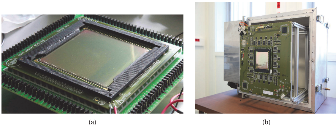
FIGURE 2.5 – (a) Détecteur silicium DSSD (Double-sided Silicon Strip Detector). (b) Enceinte réfrigérante accueillant les DSSDs.
