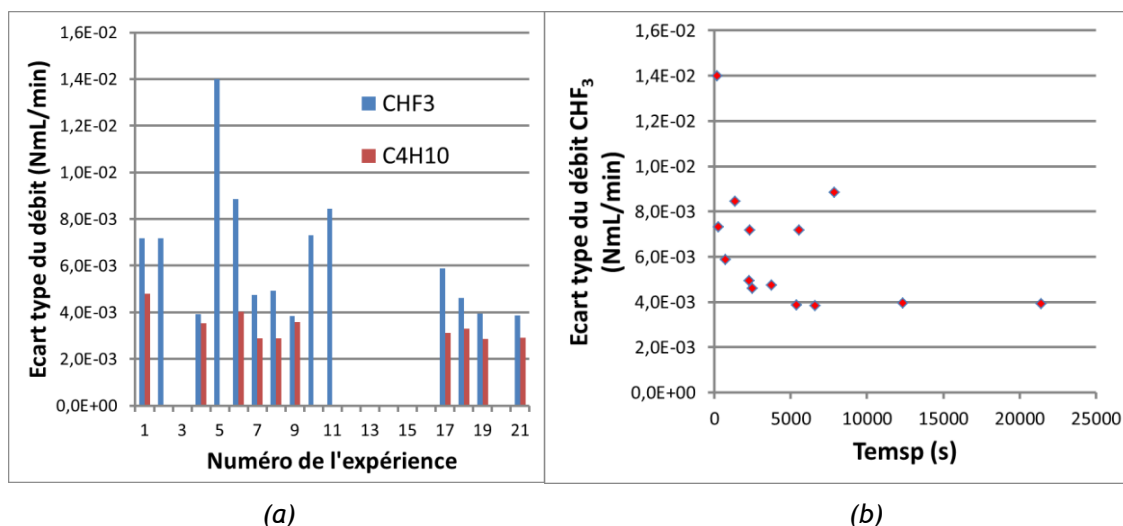
Figure 105. Ecart-type du débit mesuré lors de différentes expériences de répétabilité (a). Ecart-type du débit de \text{CHF}_3 en fonction de la durée des différentes expériences (b).
