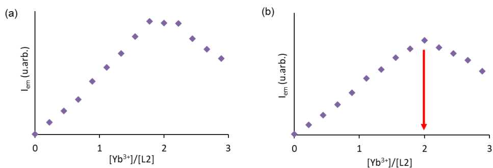
Figure III.5. Evolution de l'intensité d'émission de l'Yb(III) en fonction du rapport [Yb^{3+}]/[L2] pour des batchs d'une solution de L2 ( 4,82 \times 10^{-5} M ) avec différentes quantités d'une solution d' YbCl_3 \cdot 6H_2O ( 3,92 \times 10^{-4} M ) dans 10 mM TRIS/HCl, pH = 7,3 (a) après 5 jours à température ambiante (b) après 3 jours supplémentaires à 50°C ( \lambda_{exc} = 270 nm ).
