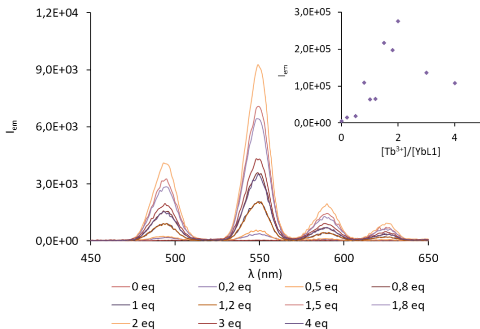
Figure II.18. Spectres d'émission mesurés lors du titrage par TbCl_3 \cdot 6H_2O d'une solution à 0,99 mM de [YbL1] dans D_2O ( \lambda_{exc} = 980 \text{ nm} , P_{980} = 1,08 \text{ W} , 10 scans). Encart : Évolution de l'intensité d'émission en fonction du rapport [Tb^{3+}]/[YbL1] .
