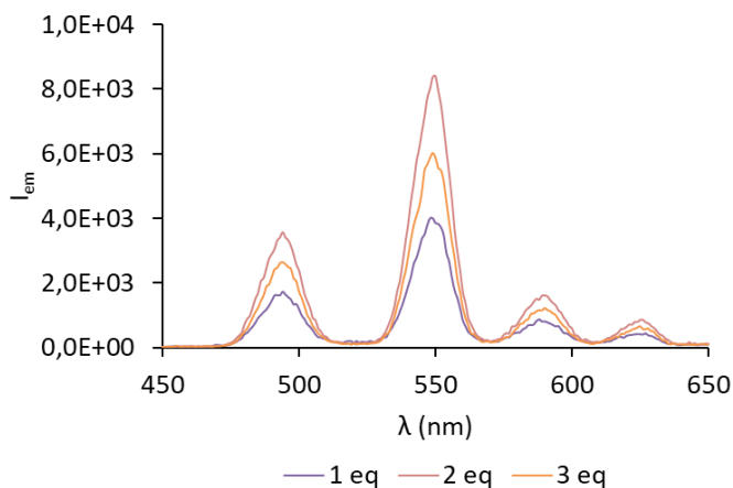
Figure IV.36. Spectres d'émission mesurés pour des batches d'une solution de [Yb_2L5] dans D_2O avec différentes quantités de TbCl_3 \cdot 6H_2O , après 6 jours à 60^\circ C ( \lambda_{exc} = 980 \text{ nm} , P_{980} = 1,08 \text{ W} , 10 scans).
