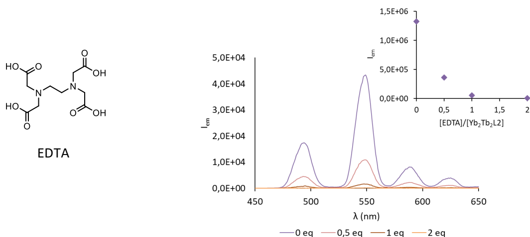
Figure IV.22. Spectres d'émission mesurés lors de l'ajout d'EDTA à une solution contenant le complexe hétéropolynucléaire à 0,56 mM dans D_2O et 1 équivalent supplémentaire de chaque cation Yb(III) et Tb(III) ( \lambda_{exc} = 980 nm, P_{980} = 1,08 W, 10 scans). Encart : Evolution de l'intensité d'émission en fonction du rapport [EDTA]/[Yb_2Tb_2L_2] .
