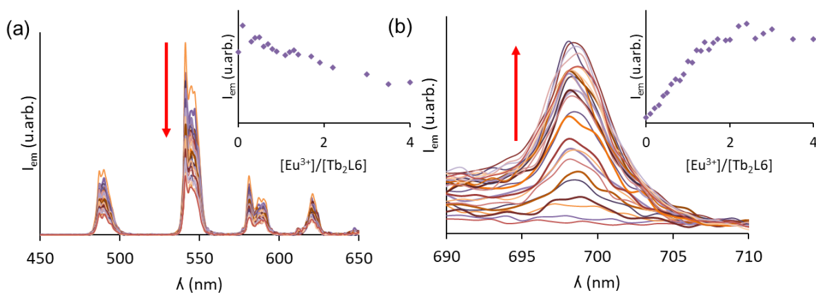
Figure 4. (a) Evolution de l'intensité de la luminescence de Tb(III) lors de l'ajout de quantités croissantes d'une solution de EuCl_3 \cdot 6H_2O à une solution de [Tb_2L6] ( \lambda_{exc} = 270\text{ nm} ). Encart : Evolution de l'intensité d'émission à 545 nm en fonction du rapport [Eu^{3+}]/[Tb_2L6] . (b) Evolution de l'intensité de la luminescence de Eu(III) lors de l'ajout de quantités croissantes d'une solution de EuCl_3 \cdot 6H_2O à une solution de [Tb_2L6] ( \lambda_{exc} = 270\text{ nm} ). Encart : Evolution de l'intensité d'émission à 698 nm en fonction du rapport [Eu^{3+}]/[Tb_2L6] .
