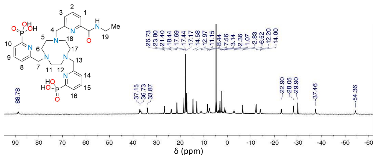
Figure II.8. Spectre RMN ^1\text{H} (400 MHz, 298 K, \text{D}_2\text{O} , pD=7,0) de [YbL1] et numérotation utilisée pour l'attribution des signaux dans le complexe [YbL1].
