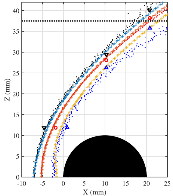
FIGURE 4.41 – Cylindre \varnothing 20 - 50 à Mach 4 : Pied de choc (●●●), centre de choc (●●●), maximum de densité (●●●), pied de choc Pitot (▼), centre de choc Pitot (○), maximum de pression Pitot (▲), pied de choc DSMC (+), centre de choc DSMC (+), maximum de pression DSMC (+).
