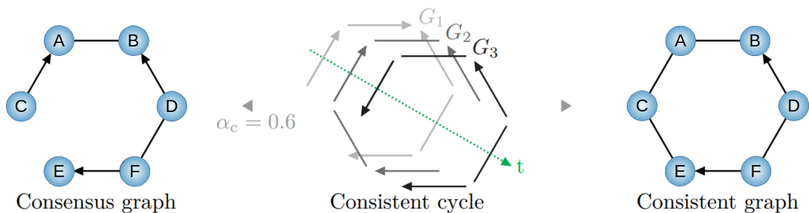
FIGURE 2.14 – Graphes consistant et consensus. Au milieu, le cycle consistant de taille 3. A droite, le graphe consistant en terme d'orientation. A gauche, graphe consensus avec \alpha_c = 0,6 .
