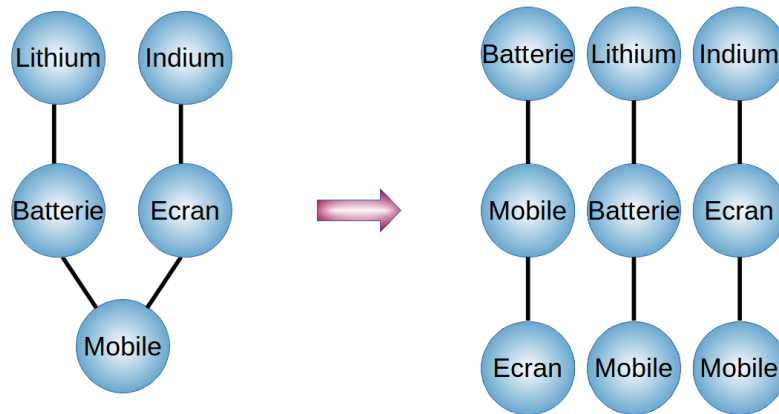
FIGURE 2.3 – Extraction des triplets ouverts. Un triplet ouvert est un ensemble de trois nœuds X, Y, Z \mid X - Z - Y et X \not\perp Y .
