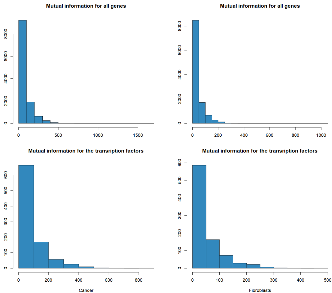
FIGURE 7.14 – Information mutuelle entre la variable traitement versus contrôle avec les gènes et les facteurs de transcription.
