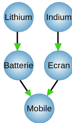
FIGURE 2.1 – Graphe causal attendu : le réseau attendu comporte des liens causaux g enuines (dont nous sommes s urs de la cause et de l'effet, repr esent es par des pointes de fl eches vertes) Lithium → Batterie , Batterie → Mobile , Indium → Ecran et Ecran → Mobile .
