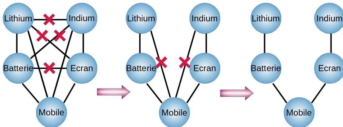
FIGURE 2.2 – Etape du squelette : A partir d'un r eseau complet, les ar etes sont retir ees sur le base de tests d'ind ependance non conditionnelle, puis conditionnelle pour parvenir au squelette.
