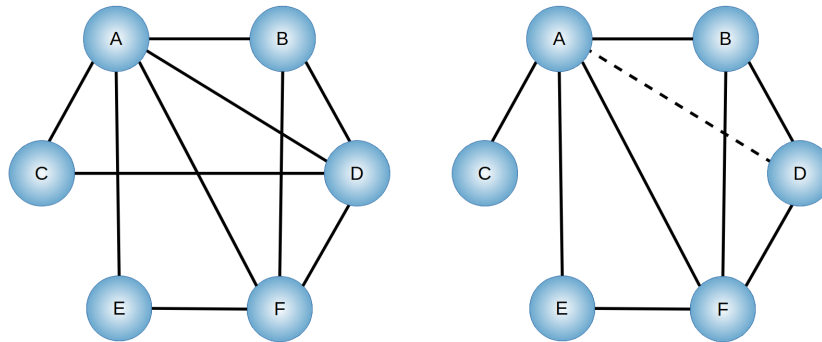
FIGURE 2.11 – Inconsistance au niveau du squelette. Le graphe de gauche illustre qu’à un moment antérieur de la reconstruction, il y avait un chemin entre A et D via C avec A \perp\!\!\!\perp D \mid \{C, F\} . Cependant, sur le squelette du graphe final à droite, il est possible de voir que l’arête entre C et D a été supprimée ultérieurement, et que C n’est donc plus dans un chemin entre A et D , ce qui rend l’ensemble de séparation C, F incohérent avec le graphe final.
