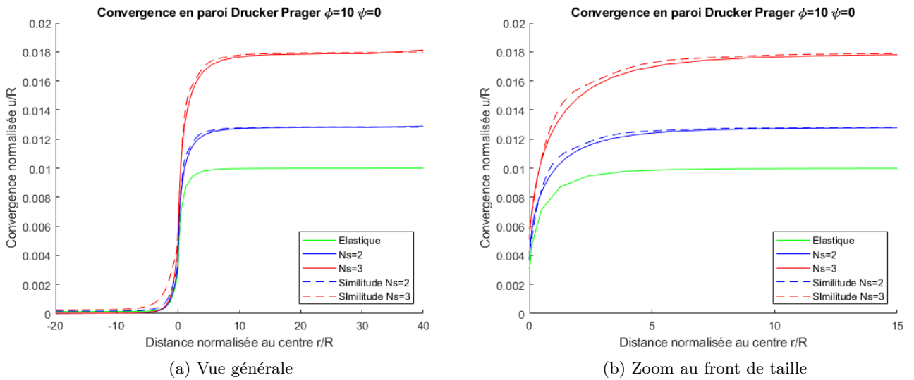
FIGURE D.11 – Profil longitudinal de convergence et vérification du principe de similitude
