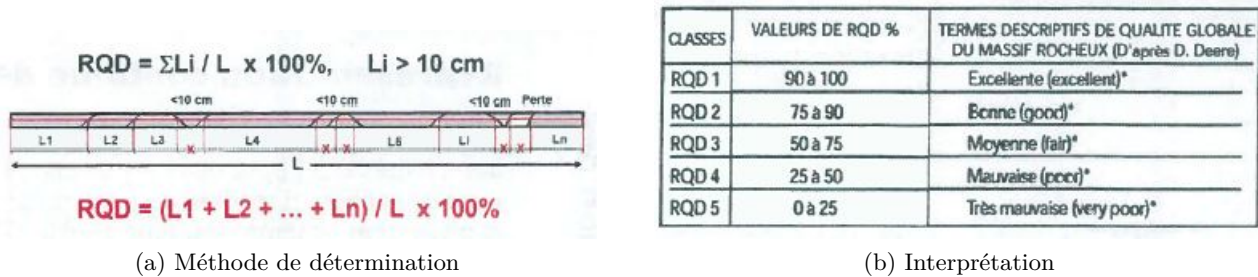
FIGURE 1.2 – Détermination et interprétation de l'indice RQD d'après [42]
