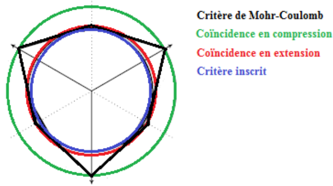
FIGURE 3.7 – Concordance entre Drucker-Prager et Mohr-Coulomb [95]
