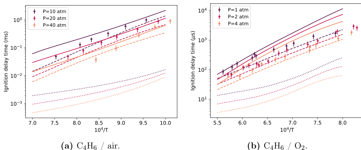
FIGURE I.4.5 Délai d'allumage pour deux mélanges avec C_4H_6 en conditions riches ( \phi = 2 ). Symboles : expérience [75]. Lignes pleines : modèle proposé. Tirets : modèle de Laskin et al. [7]. Lignes pointillées : modèle de Gross & Beckstead [5].
