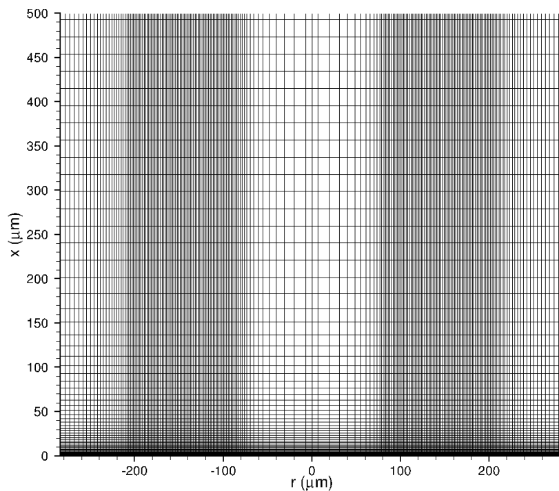
FIGURE II.2.12 Maillage employé pour le calcul de la flamme PA/PBHT. Diamètre de la particule de PA 400 \mu m , pression 20 atm.
