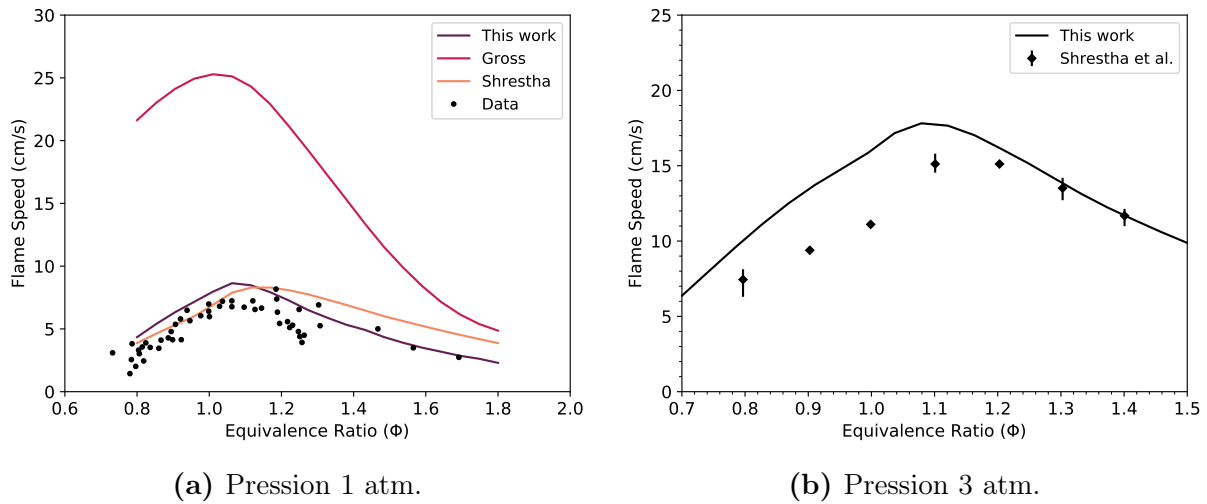
FIGURE I.3.2 Vitesse de flamme laminaire en fonction de la richesse pour des mélanges \text{NH}_3/\text{air} à 298 K et pour deux pressions. Symboles : expériences. (a) [58–63], (b) [64]. Traits : modèles.
