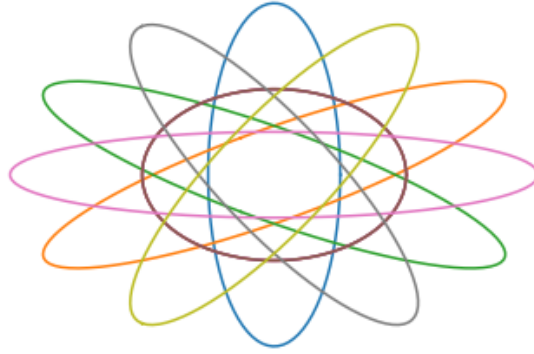
FIGURE 6.4: Ellipses autorisées pour les instances résolues par le modèle LinE
