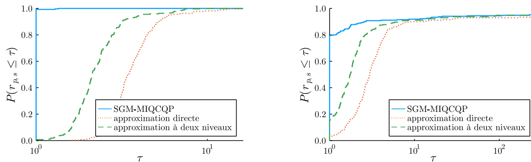
(a) Résultats pour les instances inv234
