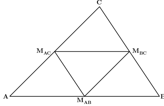
FIGURE 1.6: Exemple de raffinement d'une pièce de domaine triangulaire en quatre pièces par la méthode red refinement
