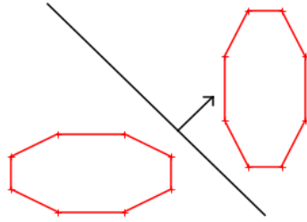
FIGURE 6.2: Séparation linéaire de l'approximation extérieure de deux ellipses par la droite noire
