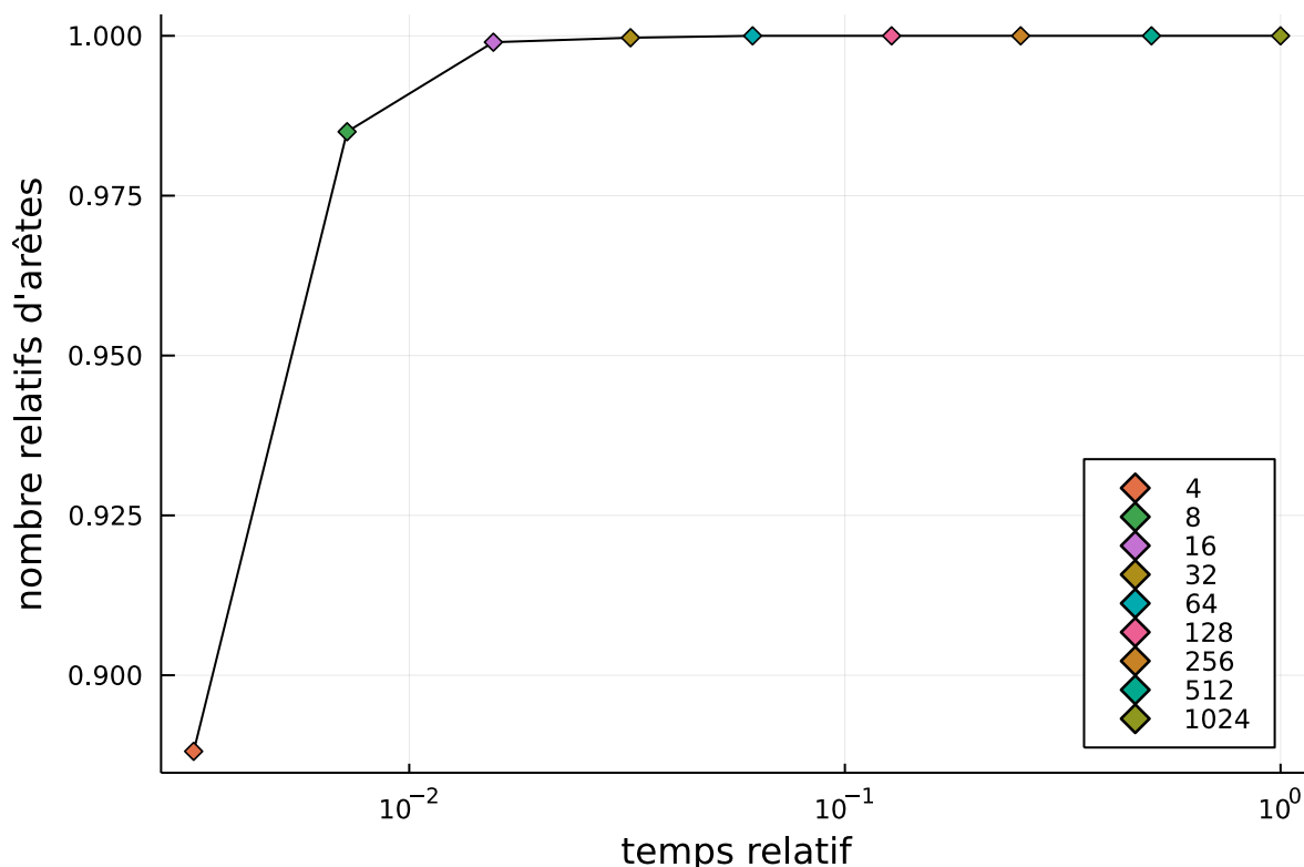
FIGURE 4.4: Proportion d'arêtes trouvées et temps de calcul en fonction du paramètre N_{\text{echantillons}}
