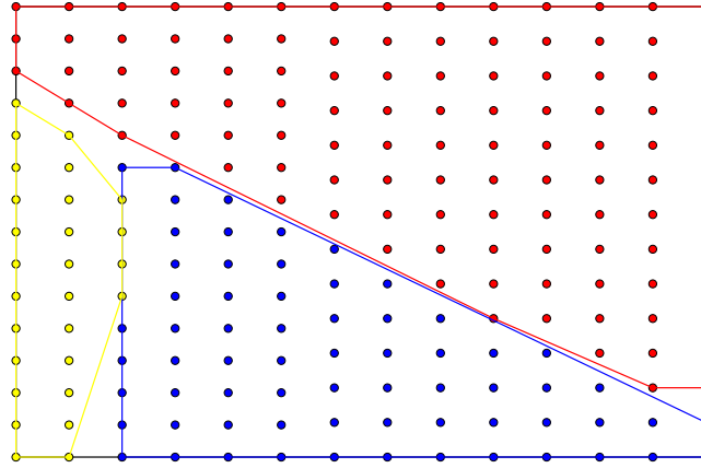
FIGURE 4.3: Exemple de solution du modèle MILP (4.23)-(4.40)
