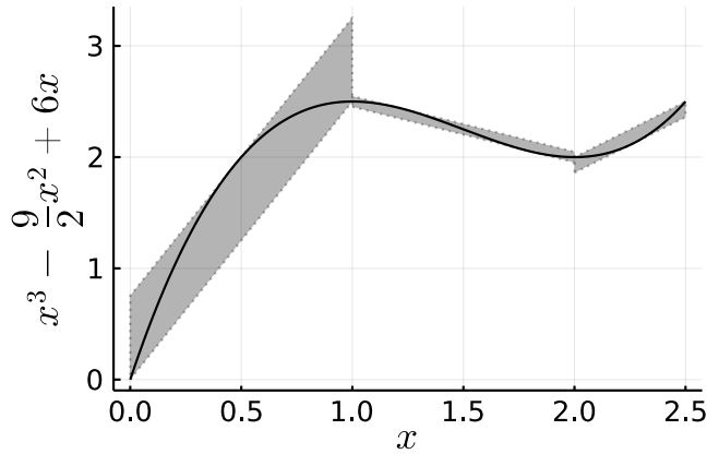
FIGURE 1.5: Enveloppes polygonales de la relaxation de la fonction x^3 - \frac{9}{2}x^2 + 6x sur [0, 2.5] avec les points de cassure 0, 1, 2 et 2.5.
