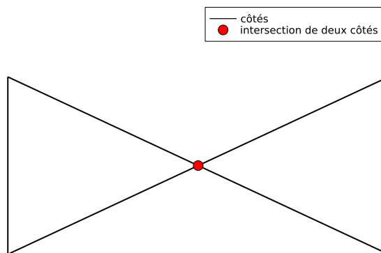
FIGURE 1: Exemple de polygone non simple à quatre côtés
