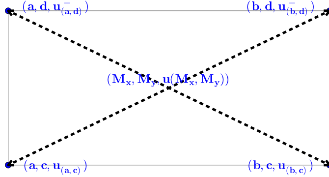
FIGURE 3.9: Schéma illustrant la construction d'une pièce du corridor intérieur PWL d'après le Lemme 23
