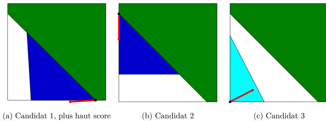
FIGURE 3.3: Itération 2 : pièces candidates pour la deuxième pièce de la trame
