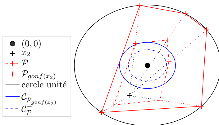
FIGURE 5.5: gonflement de \mathcal{P} par x_2 = (-0.25, -0.5)
