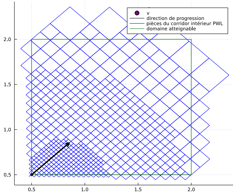
FIGURE 3.10: Un exemple de domaine des pièces du corridor intérieur PWL
