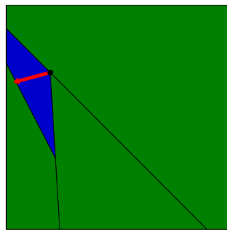
(a) Candidat 1, pièce qui traverse le corridor restant
