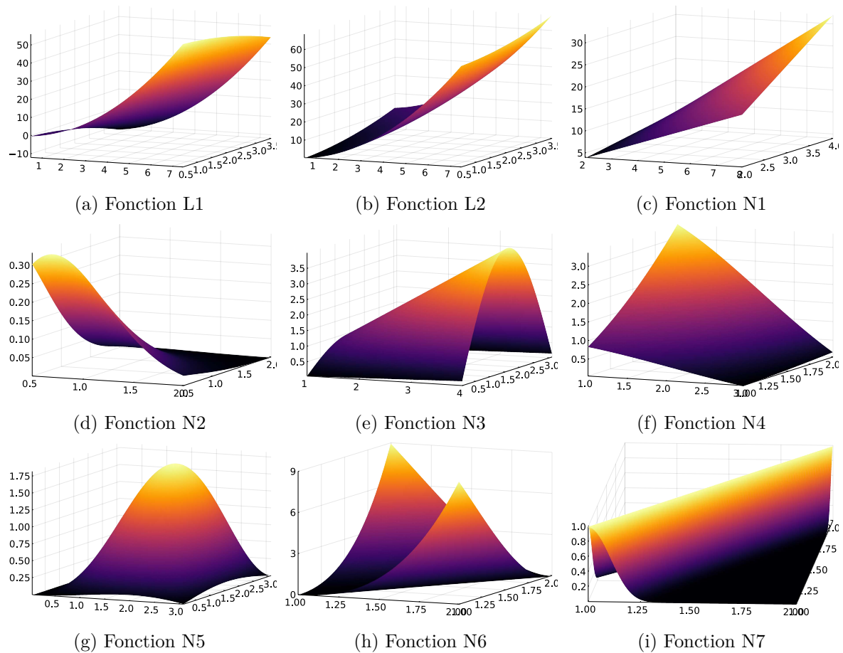
FIGURE 3.13: Toutes les fonctions du jeu d'instances de [Rebennack et Kallrath, 2015a]
