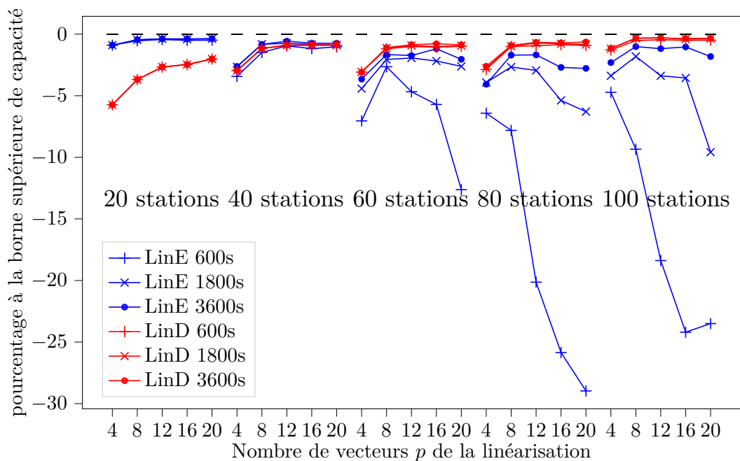
FIGURE 6.8: Résultats pour les instances à forte densité
