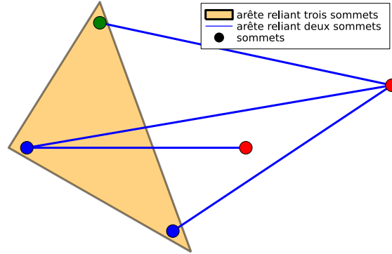
FIGURE 4.1: Exemple de coloration d'hypergraphe
