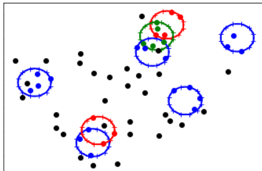
FIGURE 6.5: Exemple de solution réalisable avec le modèle LinD
