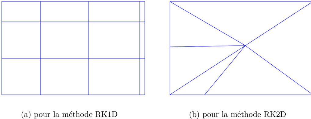
FIGURE 1.7: Exemple de subdivision du domaine de la fonction PWL pour différentes méthodes
