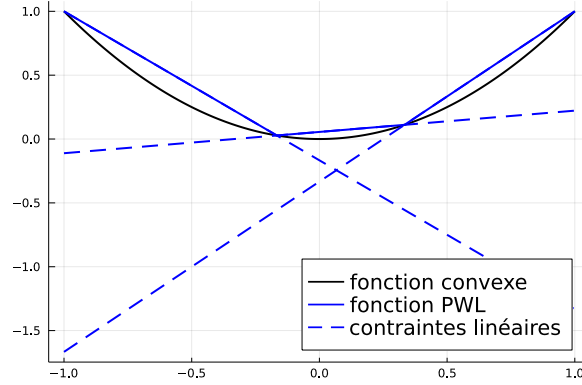
FIGURE 1.4: Exemple de formulation de fonction PWL convexe à trois pièces
