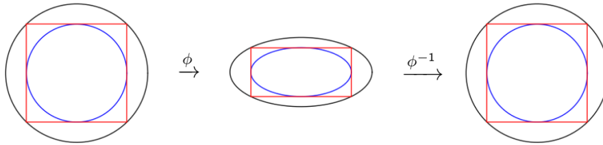
FIGURE 5.8: Transformation linéaire entre un cercle et une ellipse
