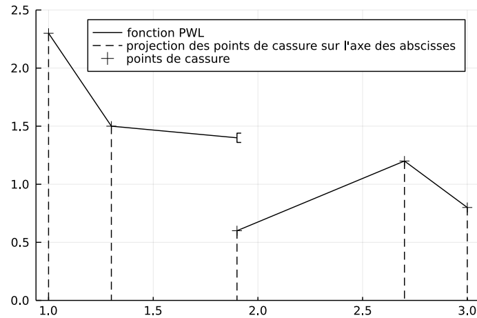
FIGURE 1.2: Fonction PWL d'une variable
