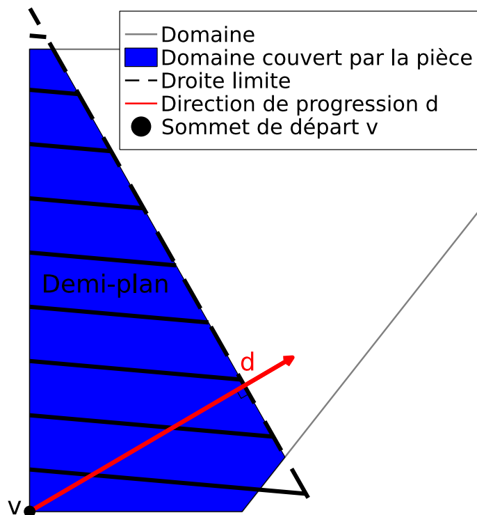
FIGURE 3.7: Représentation d'une solution de problème de pièce maximale dans la direction de progression
