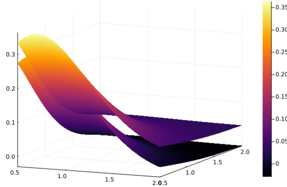
FIGURE 3.1: Corridor pour la fonction f(x, y) = xe^{-x^2-y^2} sur le domaine [0.5, 2.0] \times [0.5, 2.0] et l'erreur absolue de 0.03
