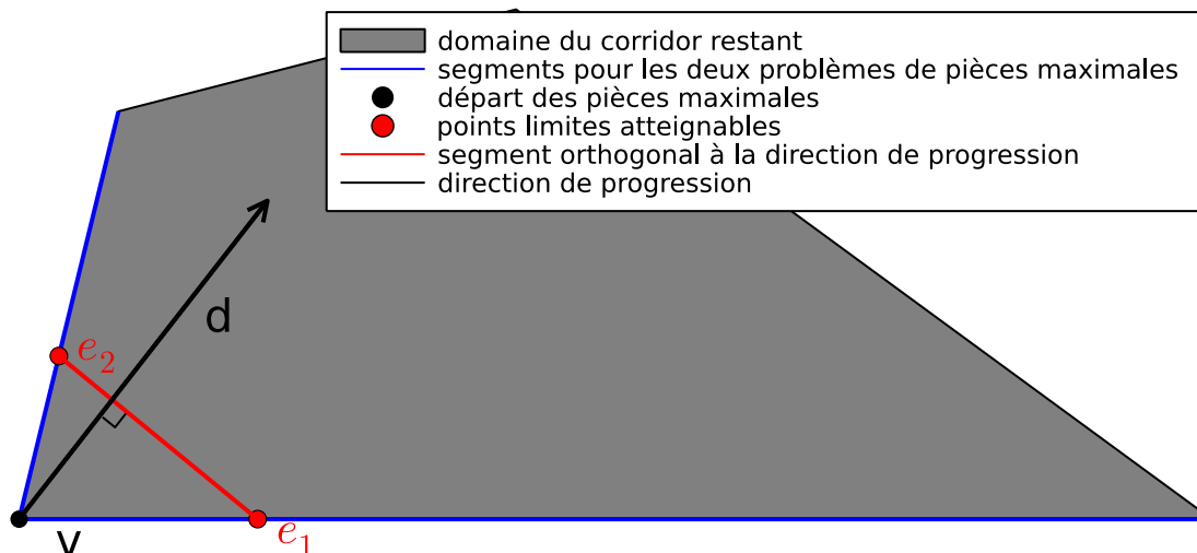
FIGURE 3.11: Construction de la direction de progression pour le composant ProMA
