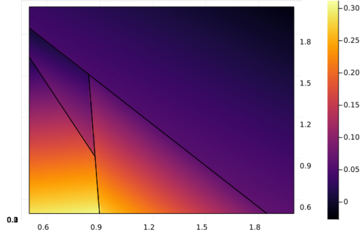
FIGURE 3.6: Valeurs de la fonction PWL construite
