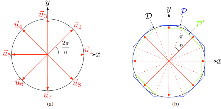
FIGURE 5.1: Linéarisation de la norme euclidienne pour 8 directions Camino et al. [2019]
