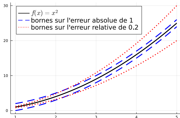
FIGURE 2.1: Seuils d'approximation avec les erreurs absolue et relative
