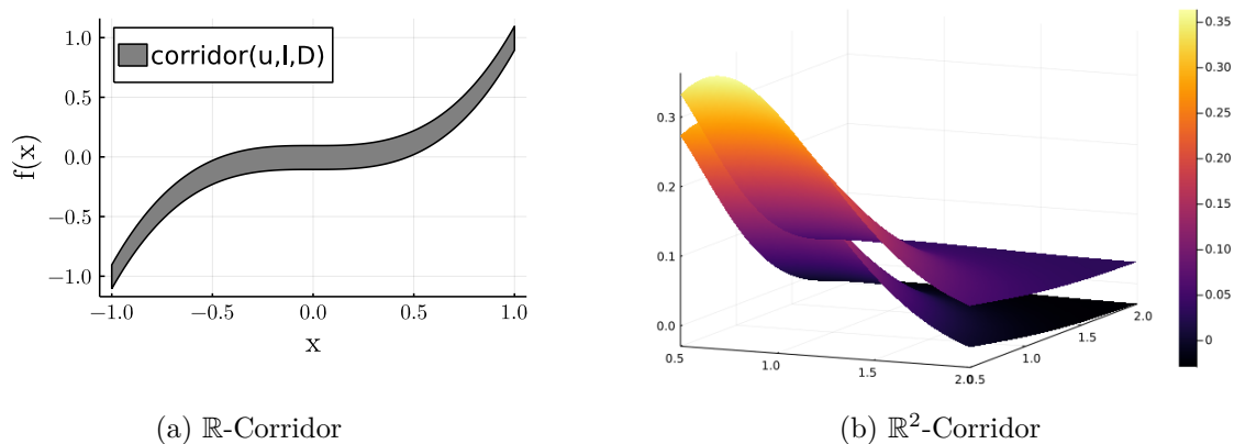
FIGURE 2.2: Deux exemples de corridors
