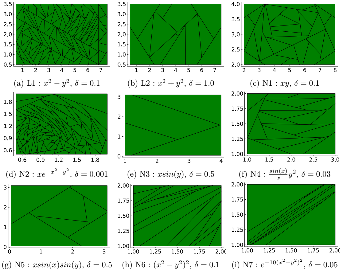
FIGURE 3.14: Exemples de solutions obtenues avec la méthode ProMA_VaT_95
