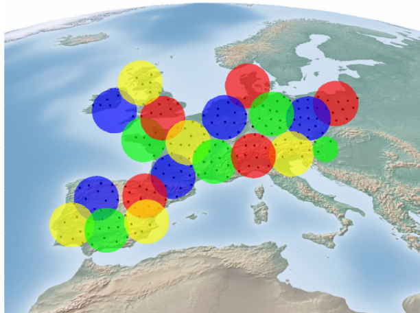
FIGURE 6.1: Exemple de solution du problème de placement de faisceaux avec seulement des faisceaux circulaires Camino et al. [2019]
