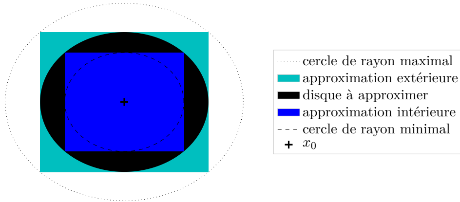
FIGURE 5.3: Encadrement du disque par les contraintes (5.3) et (5.4) pour p = 4 produits scalaires
