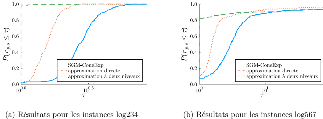
FIGURE 6.9: Profils de performances avec la fonction de coût en cybersécurité logarithmique
