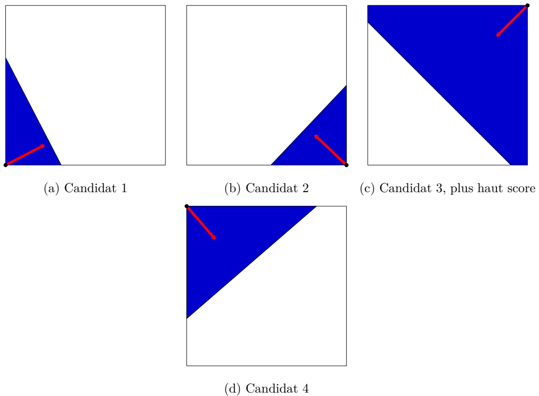
FIGURE 3.2: Itération 1 : pièces candidates pour la première pièce de la trame
