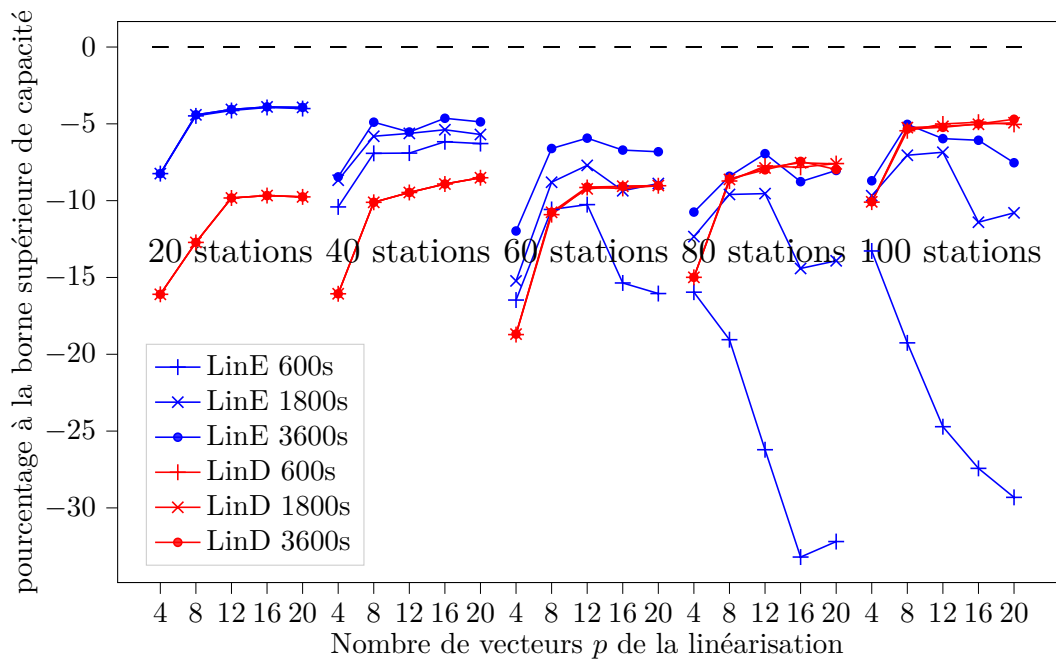
FIGURE 6.7: Résultats pour les instances à faible densité
