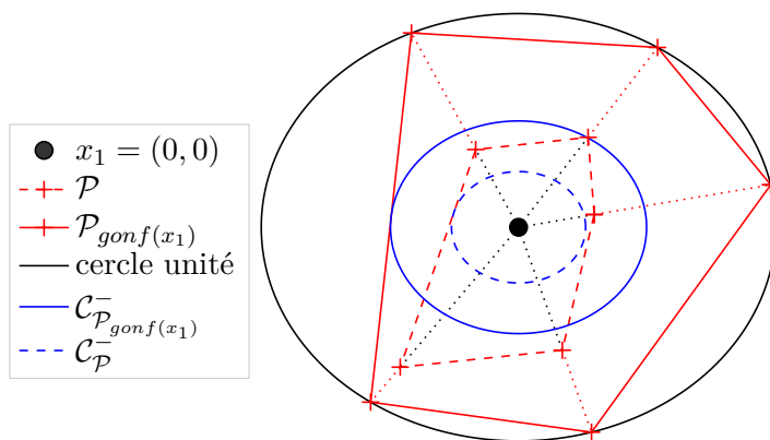
FIGURE 5.4: gonflement de \mathcal{P} par x_1 = (0, 0)
