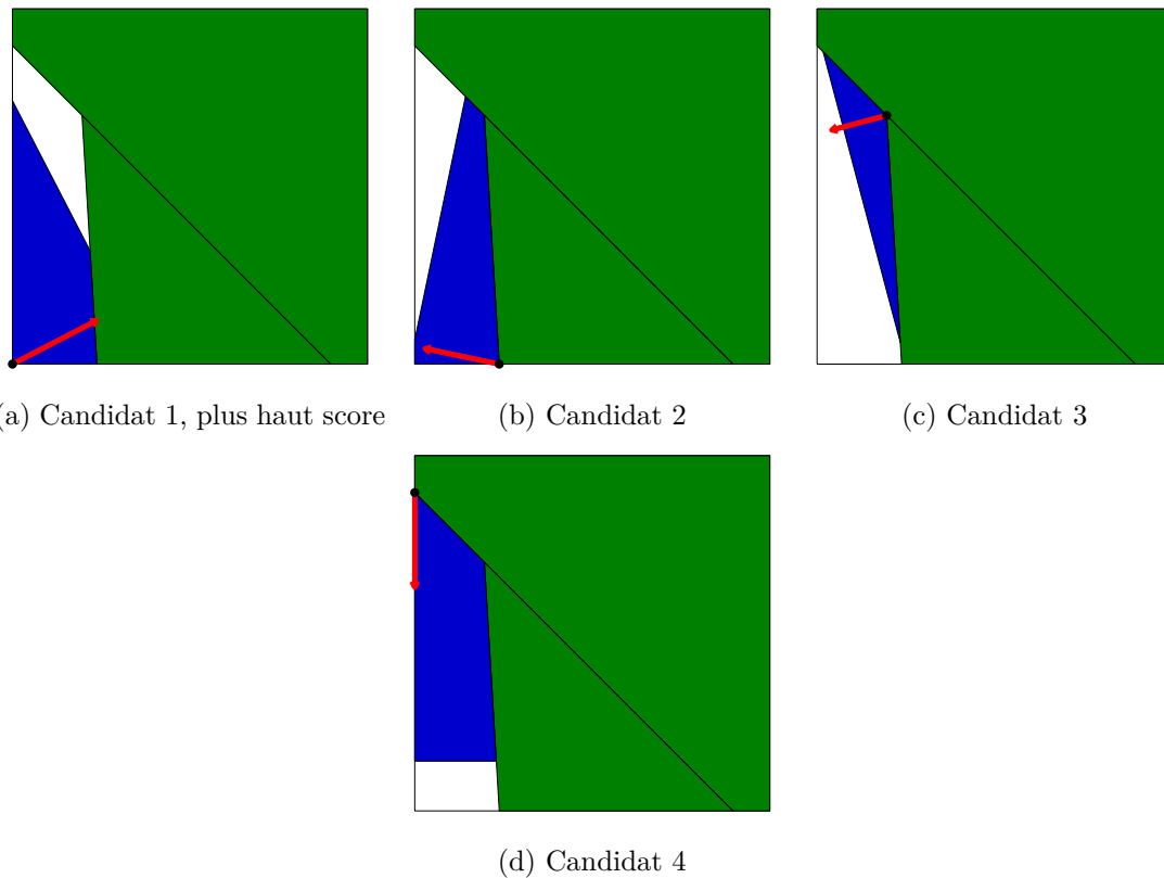
FIGURE 3.4: Itération 3 : pièces candidates pour la troisième pièce de la trame
