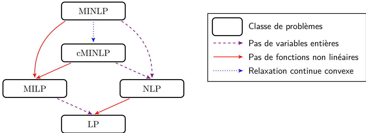
FIGURE 1.1: Sous-classes de problème MINLP
