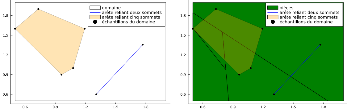
(a) Représentation d'un hypergraphe H avec deux arêtes d'incompatibilité (b) Superposition d'arêtes d'incompatibilité et d'une solution réalisable du \mathbb{R}^2 -CFP
