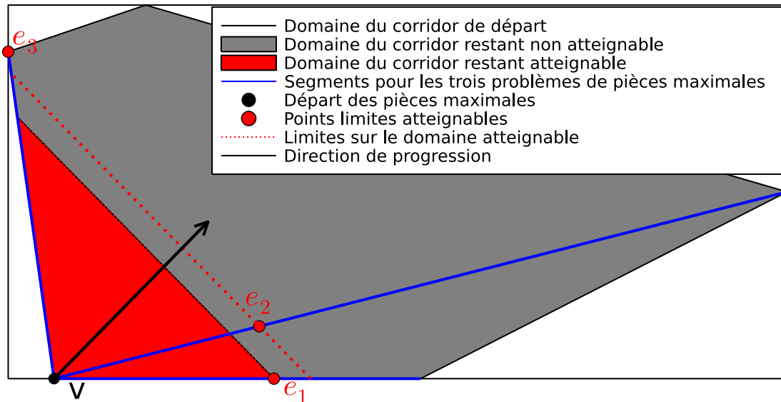
FIGURE 3.8: Construction du domaine atteignable du corridor restant
