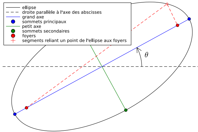
FIGURE 5.7: Représentation du vocabulaire de l'ellipse
