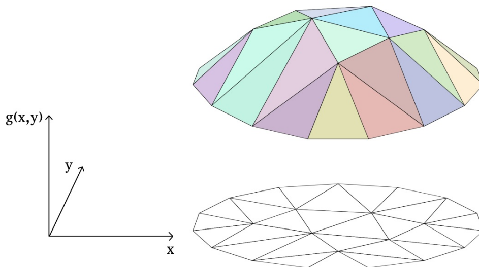
FIGURE 1.3: Fonction PWL de deux variables
