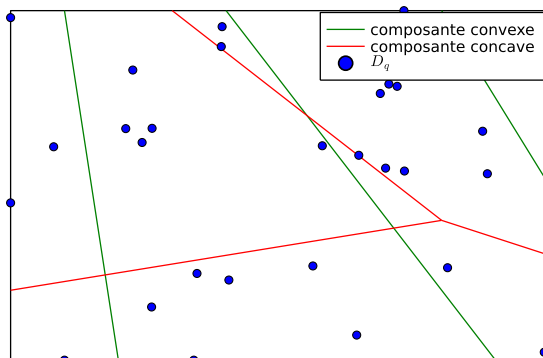
FIGURE 1.8: Représentation du domaine d'une fonction DC CPWL avec les points en lesquels l'erreur d'approximation est respectée
