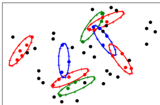
FIGURE 6.6: Exemple de solution réalisable avec le modèle LinE
