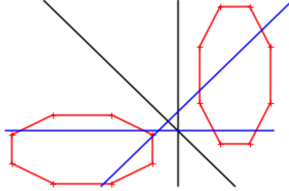
FIGURE 6.3: La séparation linéaire fonctionne avec les deux lignes noires mais ne fonctionne pas avec les deux lignes bleues
