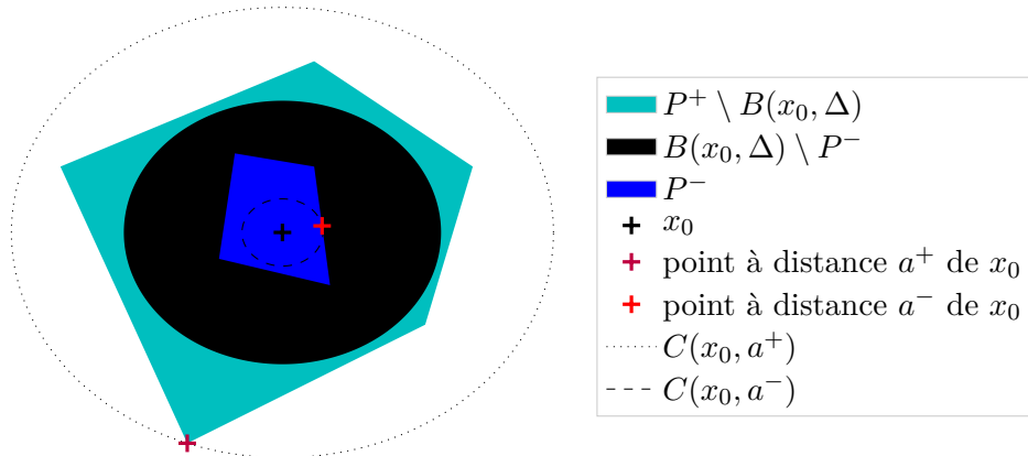
FIGURE 5.2: Illustration de la Définition 43
