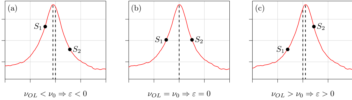
FIGURE 1.9 – Lecture du signal de part et d'autre de la résonance pour l'asservissement de la fréquence de l'oscillateur local. (a) \nu_{OL} < \nu_0 , (b) \nu_{OL} = \nu_0 , (c) \nu_{OL} > \nu_0 .
