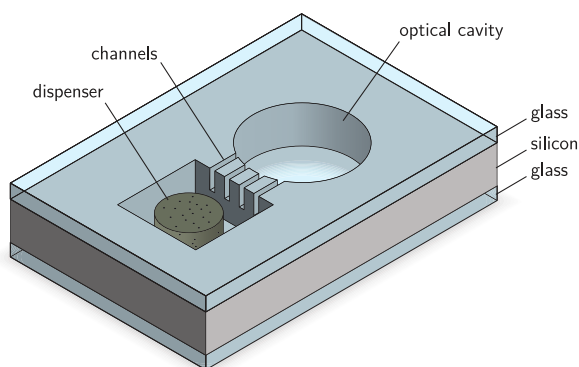
FIGURE 3.2 – À gauche, schéma de la micro-cellule (extrait de [29]). À droite, photographie d'une micro-cellule fabriquée au sein du laboratoire FEMTO-ST (prise par N. Passilly).
