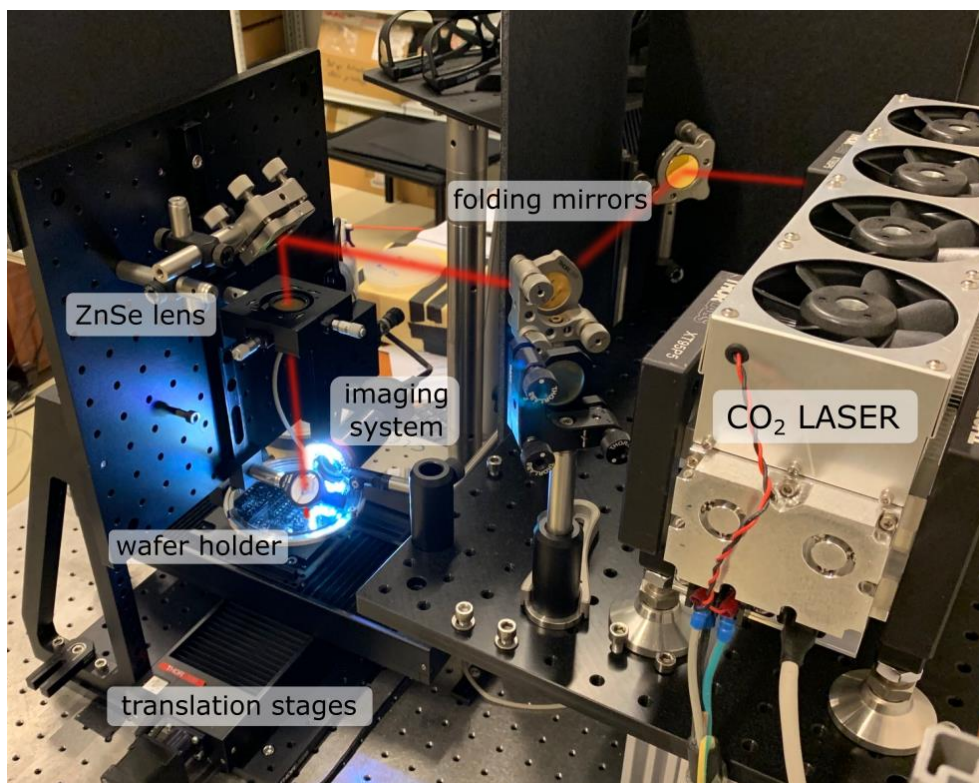
FIGURE 3.38 – Banc expérimental avec un laser CO 2 pour activer les vannes fermantes.
