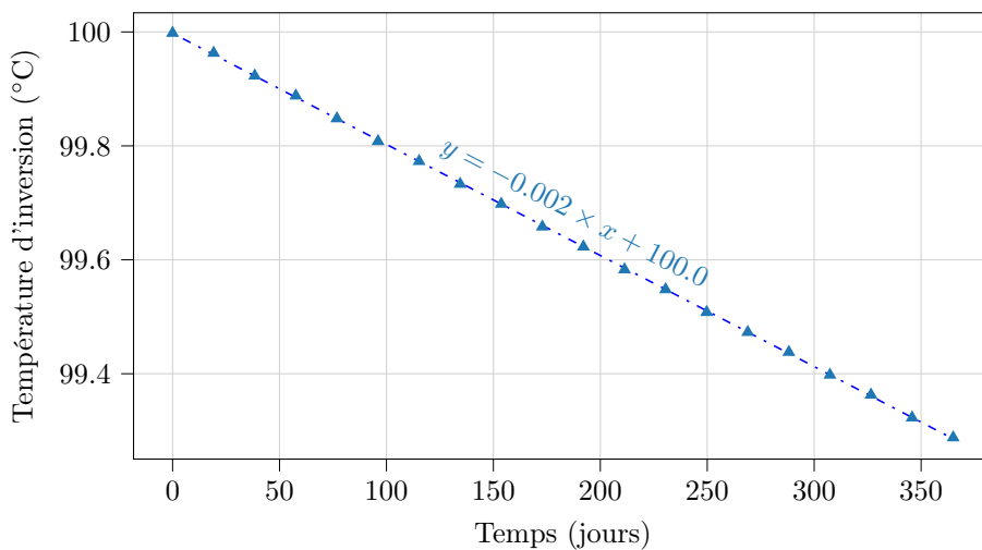
FIGURE 3.20 – Déplacement du point d'inversion en fonction du temps pour une cellule Cs-Ne-He à base d'ASG à 100^\circ\text{C} . Le déplacement calculé est supposément induit par une perméation progressive de l'hélium en dehors de la cellule.
