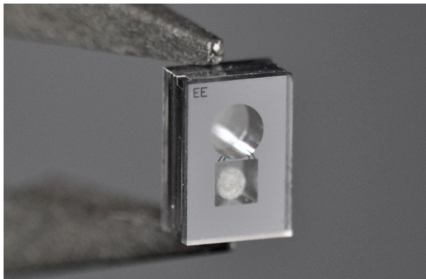
FIGURE 3.2 – À gauche, schéma de la micro-cellule (extrait de [29]). À droite, photographie d'une micro-cellule fabriquée au sein du laboratoire FEMTO-ST (prise par N. Passilly).
