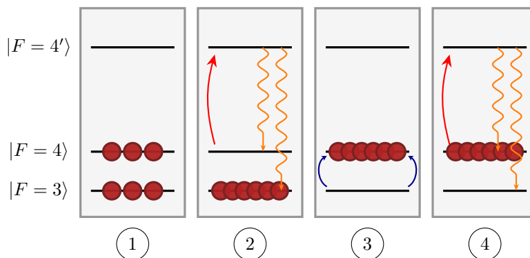
FIGURE 1.6 – Représentation graphique au niveau atomique de l'interrogation de Rabi. ① Les atomes sont présents de façon équiprobable dans les sous-niveaux fondamentaux hyperfins. ② Les atomes sont forcés à peupler le sous-niveau hyperfin |F = 3\rangle par pompage optique. ③ Les atomes interagissent avec le champ excitateur micro-onde qui entraîne le passage au niveau fondamental hyperfin supérieur |F = 4\rangle . ④ Le signal de résonance est mesuré.
