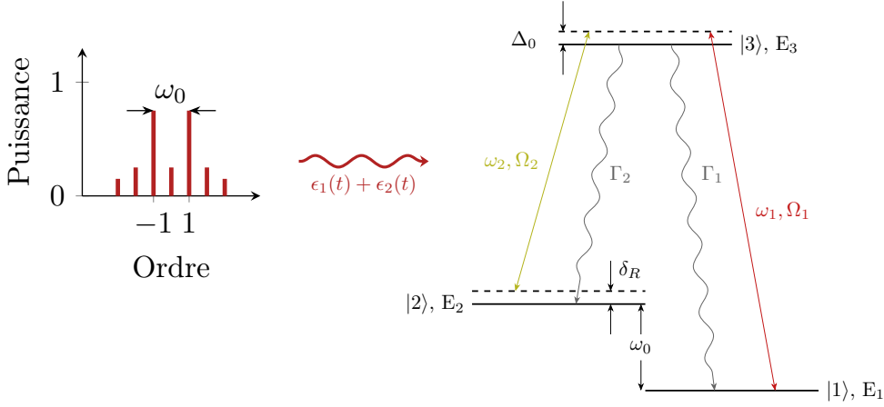
FIGURE 2.2 – Schéma- \Lambda d'un atome sondé par un champ polychromatique de fréquences \omega_1 et \omega_2 . On note \omega_0 la fréquence de résonance hyperfine, \Delta_0 le désaccord optique, \delta_R le désaccord en fréquence et \Gamma = \Gamma_1 + \Gamma_2 le taux de relaxation de l'état excité. Le spectre multifréquence du laser avec sa répartition en puissance est représenté avec la présence résiduelle de la porteuse et d'harmoniques.
