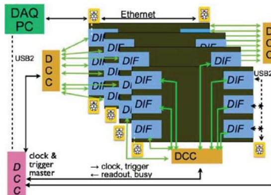
FIGURE 4.6 – Synoptique de l’architecture du système d’acquisition de TOMUVOL.
