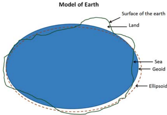
FIGURE 5.2 – Exemple de modélisation de la surface de la Terre [93].
