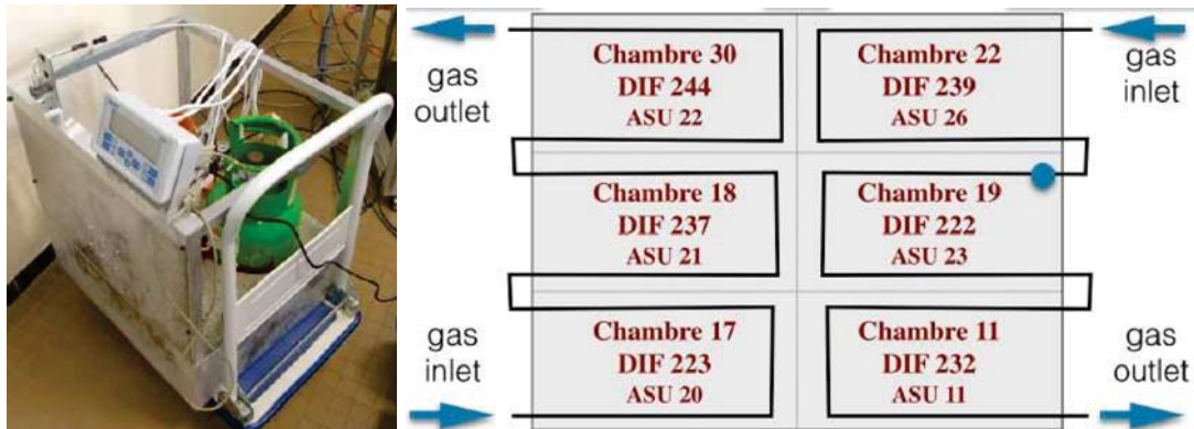
FIGURE 4.5 – Gauche : structure abritant le système de gaz ; droite : Schéma de l’écoulement du gaz à travers un plan de détection. Les quatre plans de détection utilisent quatre entrées de gaz différentes fonctionnant à des débits fixes, mais à l’intérieur d’un plan, l’entrée est divisée de telle sorte que les côtés droit et gauche partagent le débit ; les trois chambres de chaque côté sont enchaînées.
