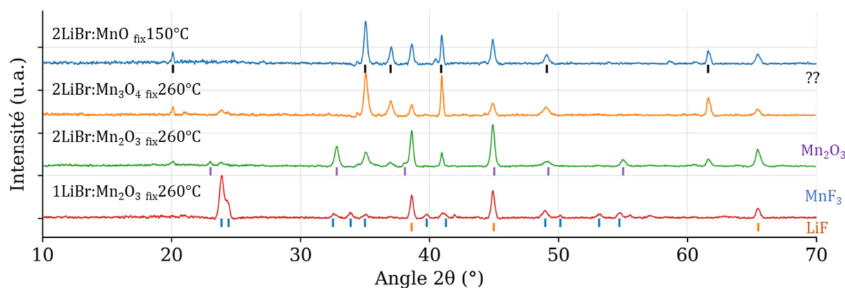
Figure 149. Diffractogrammes X sur poudre des échantillons de la série des fluorations one-pot à base de LiBr réalisées à température d'oxyfluoration de leur précurseur oxyde, acquis pendant 1h sous argon.
