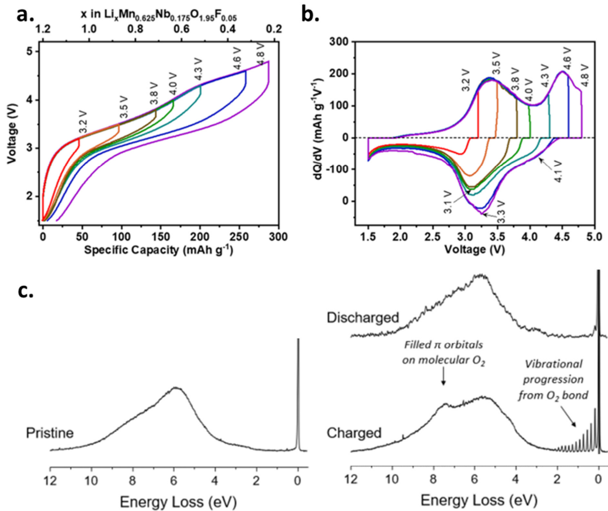
Figure 15. (a) Courbes de cyclage galvanostatique réalisées à 20 \text{ mA}\cdot\text{g}^{-1} entre 1.5 \text{ V} et une borne supérieure indiquée sur la figure a 32 . (b) Dérivée de la capacité fonction du potentiel pour les courbes de la figure a 32 . (c) RIXS au seuil K de l'oxygène pour un CDRS de formule brute \text{Li}_x\text{Mn}_{0.625}\text{Nb}_{0.175}\text{O}_{1.95}\text{F}_{0.05} réversiblement chargé jusqu'à \text{Li}_{0.8}\text{MnO}_2\text{F} 33
