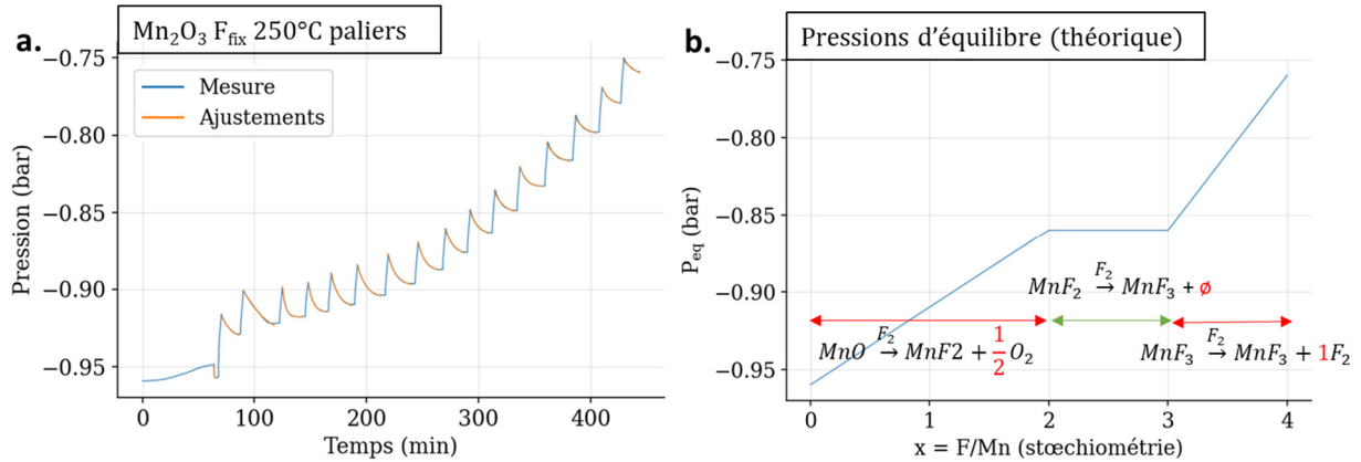
Figure 33. (a) Pression in-situ fonction du temps et ajustement exponentiel des parties décroissantes. (b) Illustration de l'évolution de la pression fonction du temps pour une expérience à injection lente et continue de fluor. Les équations bilan correspondant aux réaction successives permettent d'établir un lien entre pente de pression et stœchiométrie de produit de réaction gazeux.
