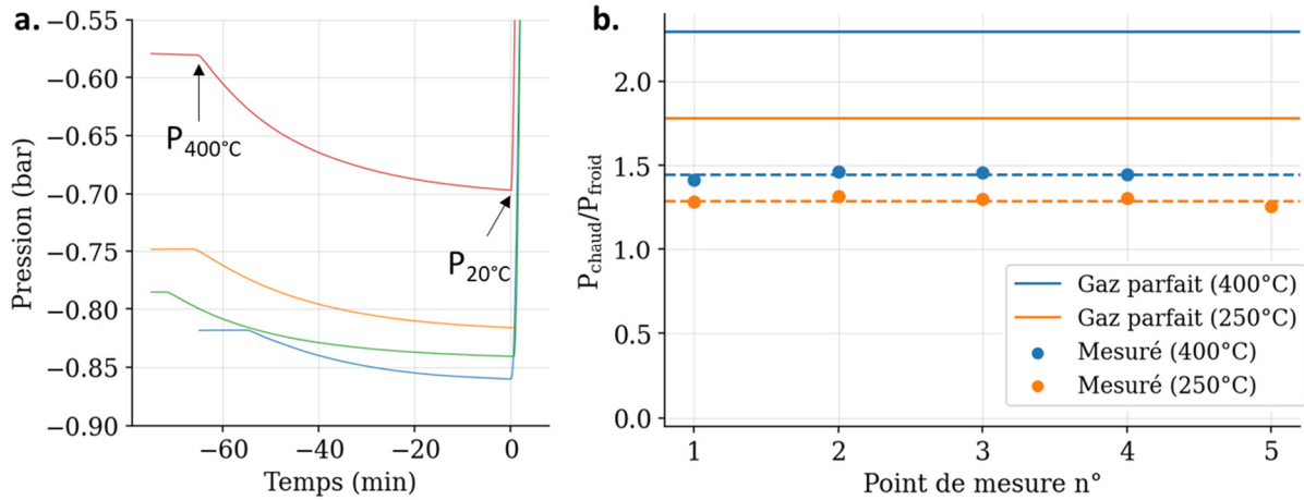
Figure 32. (a) Pression in-situ fonction du temps pour cinq étapes de trempe ( rouge : MnO F var 400°C, orange : F 2 F var 400°C, vert : Li 2 MnO 3 :MnO broyé F fix 400°C mécano-broyé en pré-traitement et bleu : MnO F fix 400°C) (b) Ratios pression à chaud / pression à froid mesurée (points), moyennes de ces séries de ratios (lignes pointillées) et ratios théoriques calculés via la loi des gaz parfaits (lignes pleines).
