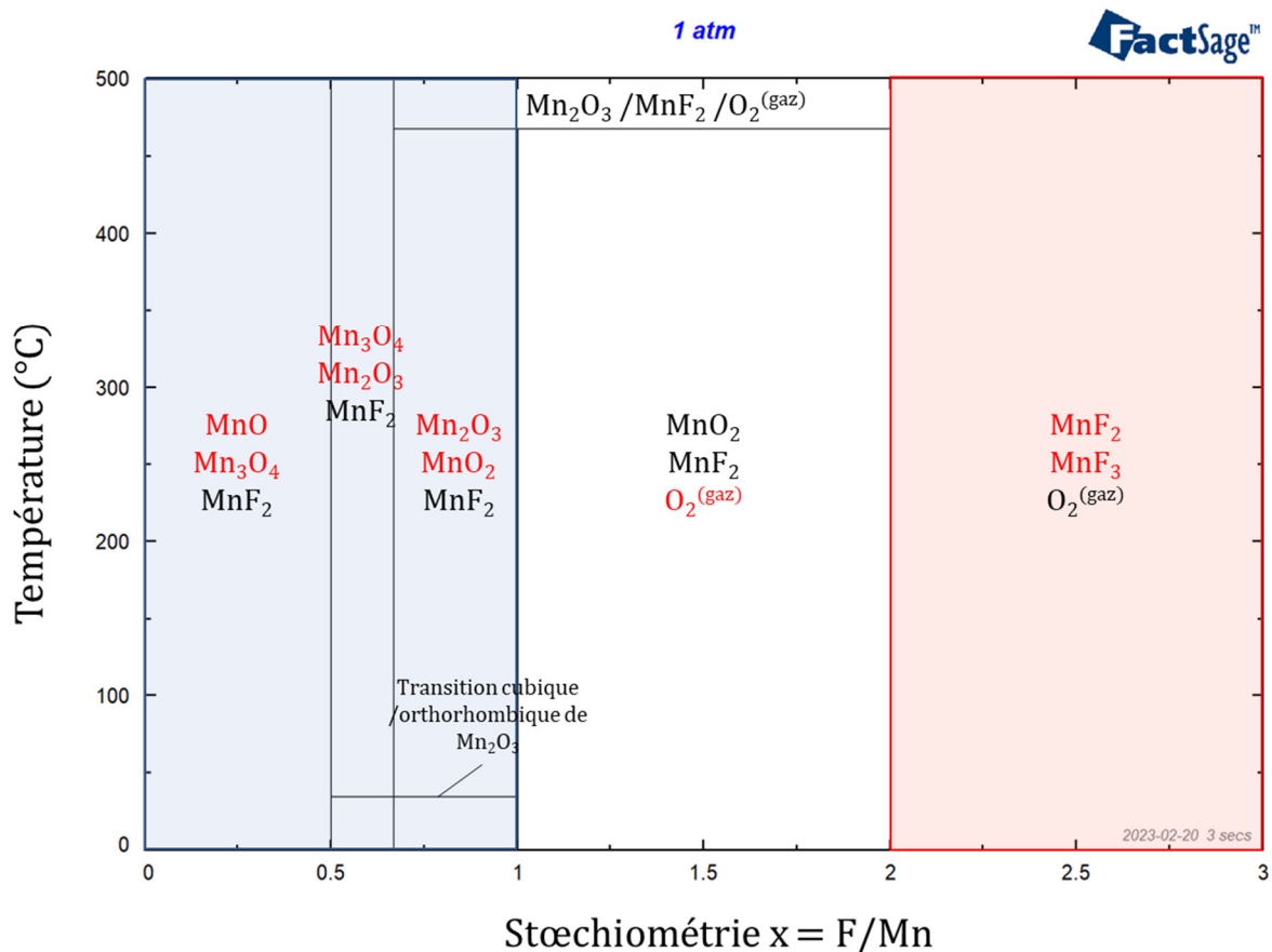
Figure 57. Diagramme de phase du binaire \text{MnO}/\text{F}_2(\text{gaz}) calculé avec le logiciel Factsage. Les couleurs représentent la séparation du diagramme en trois sections : bleu pour les faibles stœchiométries en fluor, blanc pour les moyennes et rouge pour les hautes.
