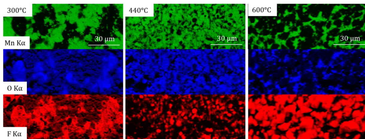
Figure 100. Cartographies EDX de la surface des produits de la série des calcinations sous vide à stœchiométrie Li 2 O :MnOF de 1 :1.
