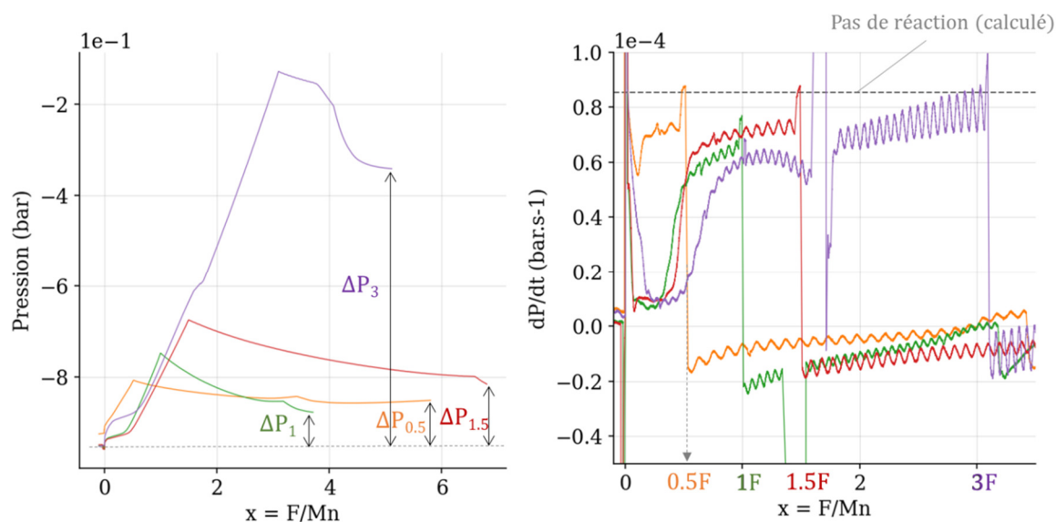
Figure 76. Pressions fonction du temps acquises durant les fluorations sous-stœchiométriques à 260°C du précurseur Mn_3O_4 . Les deltas de pression avant et après réaction mesurés à température ambiante sont indiqués sur le graphe. Dérivée temporelle de ces mêmes pressions, représentées sur un graphique dont l'axe de temps (abscisse) a été converti en axe de stœchiométries en utilisant le débit constant d'injection comme constante de conversion.
