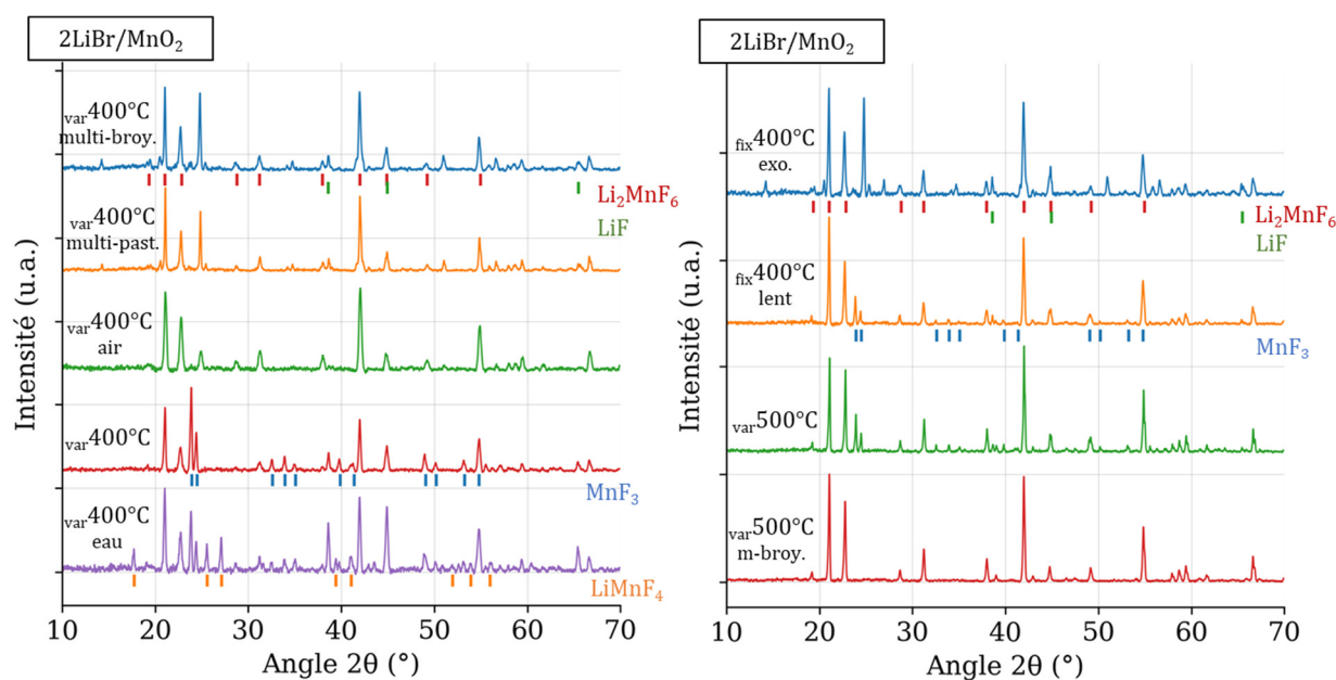
Figure 140. Diffractogrammes X sur poudre des produits de la série des fluorations one-pot à base de \text{LiBr} et \text{MnO}_2 , acquis pendant 1h sous argon.
