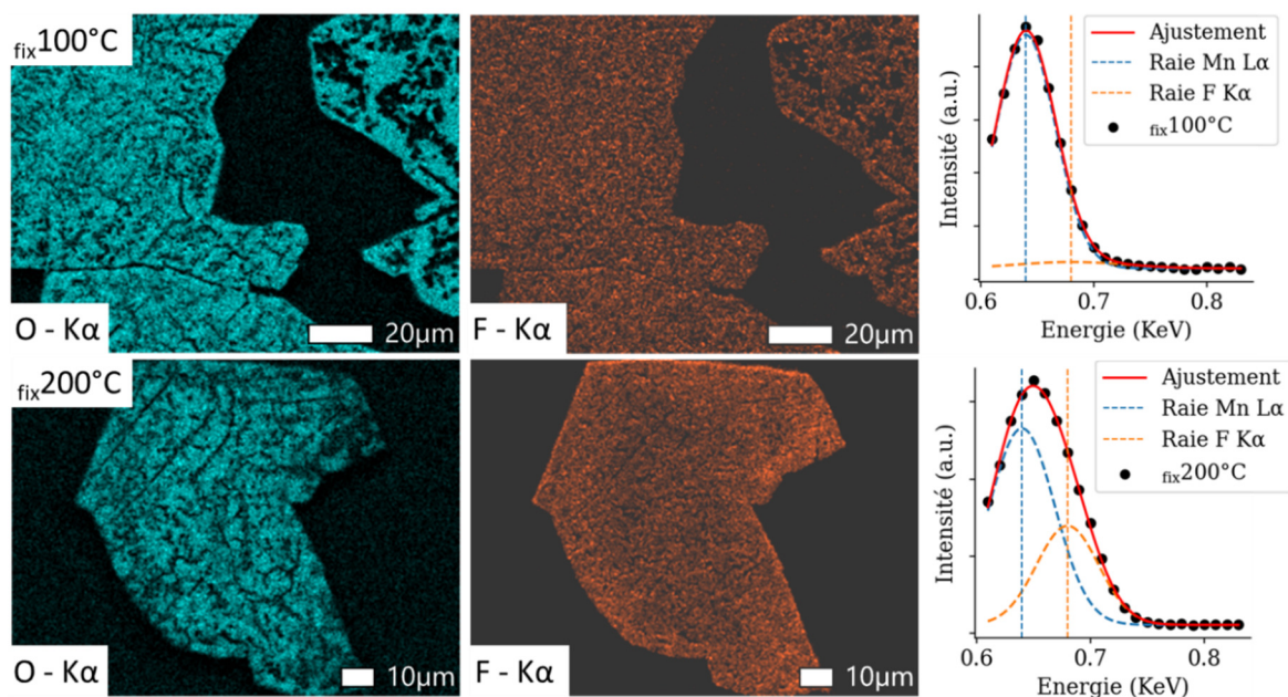
Figure 66. Cartographies EDX en coupe des produits « \text{fix}100^\circ\text{C} » et « \text{fix}200^\circ\text{C} » de la série des fluorations cinétiques. Un spectre EDX ponctuel a été acquis pour chaque produit et la déconvolution des pics Mn L \alpha et F K \alpha est représentée à droite des cartographies correspondantes.
