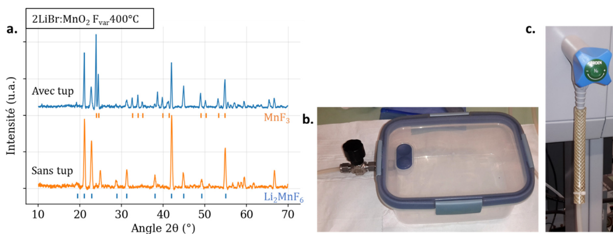
Figure 26. (a) Diffractogrammes sur poudre des produits de deux synthèses identiques en tous points excepté l'utilisation ou non du tupperware protecteur avant et après fluoration. (b) Photographie du tupperware. (c) photographie du raccord du tupperware au réseau d'azote
