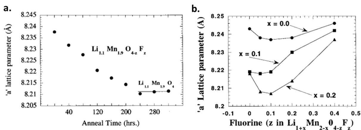
Figure 22. (a) Variation du paramètre de maille a fonction de la durée de synthèse par calcination à 800°C. (b) Variation du paramètre de maille a fonction de la concentration en fluor pour 4 stœchiométries en lithium différentes
