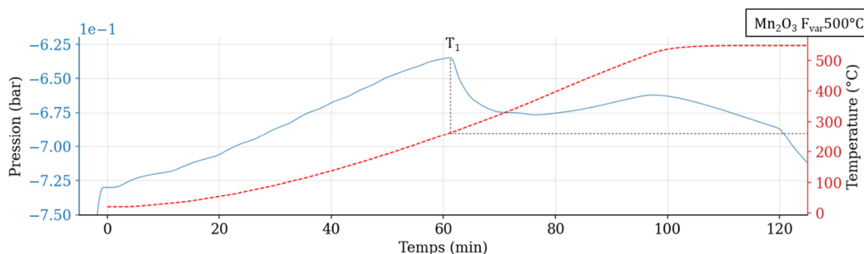
Figure 80. Résultats du protocole d'exploration de l'axe des températures appliqué à la fluoration de Mn 2 O 3 . La courbe de pression acquise est tracée en bleu avec la courbe de température de calibration en rouge. La température critique T 1 est mesurée par lecture graphique.
