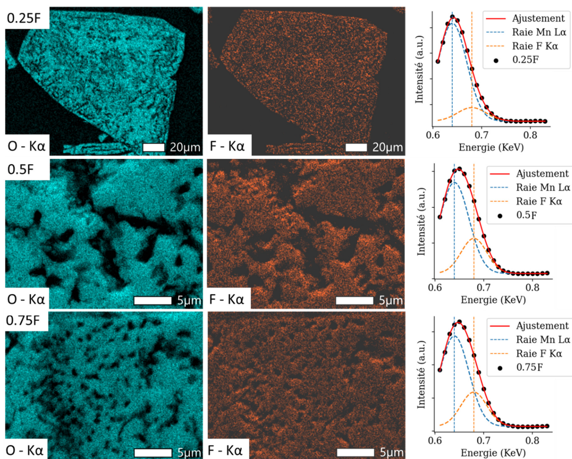
Figure 70. Cartographies EDX en coupe de produits de la série des oxyfluorations sous-stœchiométriques. Un spectre EDX ponctuel a été acquis pour chaque produit et la déconvolution des pics Mn L \alpha et F K \alpha est représentée à droite des cartographies correspondantes.
