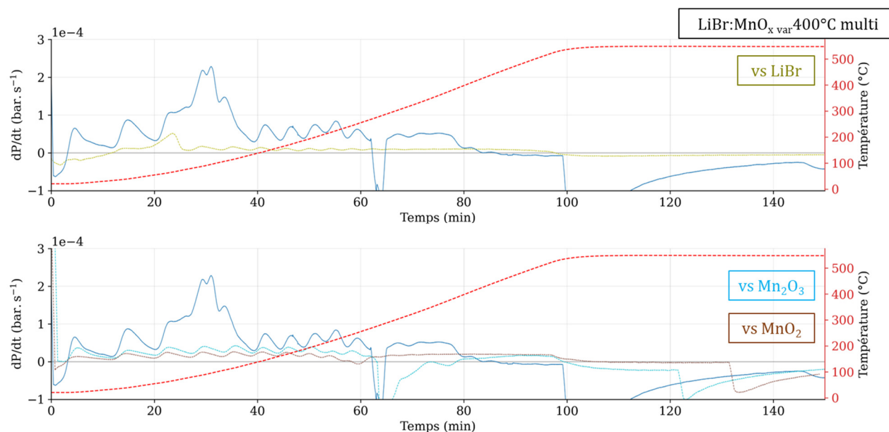
Figure 139. Protocole d'exploration de l'axe des températures appliqué à la préparation « 2LiBr:MnO x » (Mn 2 O 3 et MnO 2 ) avec une rampe de 5°C.min -1 jusqu'à 500°C. En témoin, les protocoles d'exploration de l'axe des températures appliqués à LiBr, à Mn 2 O 3 et à MnO 2 sont également tracés.
