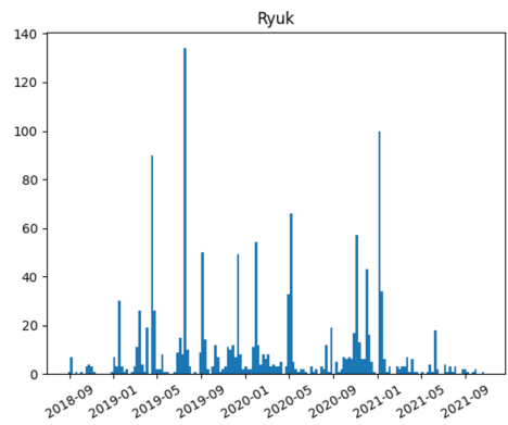
b) Ryuk
