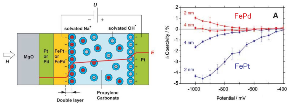
Figure 6.10: Schéma du déclenchement électrolytique d'un film de FePt ou FePd montrant la formation d'une double couche électrique sous un potentiel appliqué U (à gauche). Changements de la coercivité du FePd (rouge) et du FePt (bleu) en fonction du potentiel appliqué pour différentes épaisseurs de films (droite). Adapté de [27].
