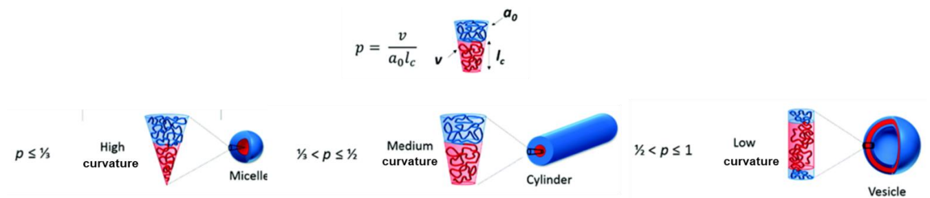
Figure II-2. Les diverses morphologies obtenues selon les différentes valeurs du paramètre d'empilement critique et la courbure du polymère
