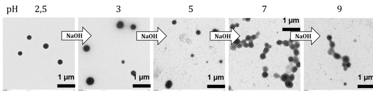
Figure V-5. Images TEM de l'échantillon contenant PAA 32 - b -PVP 59 (0.05%wt), ions Gd^{3+} (0.7 mM) et les AuNPs formées in situ ([Au]=500 µM) à différentes valeurs de pH suite à l'ajout d'une solution NaOH (1M)
