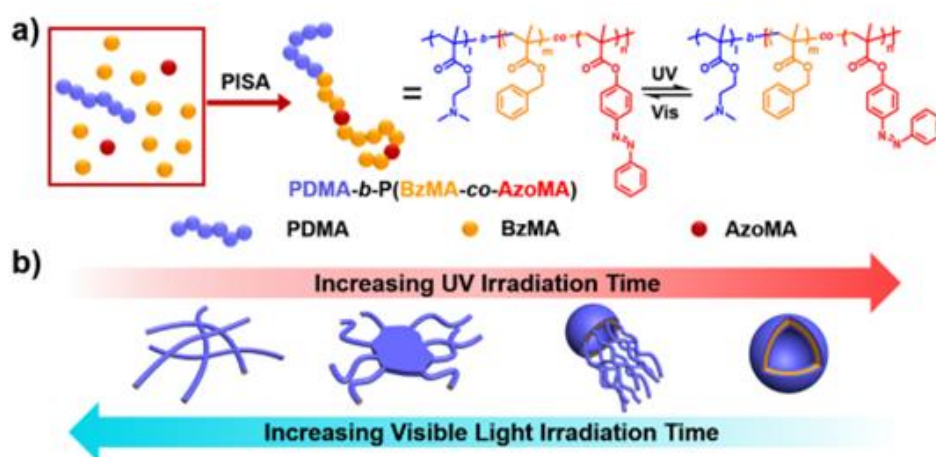
Figure II-3. (a) Préparation et isomérisation de copolymères sensible à la lumière et (b) Aperçu mécanistique des morphologies obtenues, des bâtonnets jusqu'aux vésicules, de manière photo-réversible. Le polymère à blocs a été obtenu à travers une polymérisation PISA, c'est-à-dire un processus d'autoassemblage induit par polymérisation des monomères.
