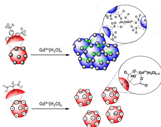
Figure IV- 3. Schéma des interactions entre les AuNP@citrate, les AuNP@BSPP et les ions Gd^{3+}
