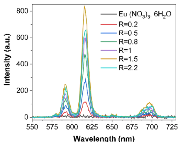
Figure III- 3. Spectres d'émission ( \lambda_{\text{ex}}=256 nm) des échantillons HPICs \text{Eu}^{3+} / PAA- b -PVP à différents ratios R
