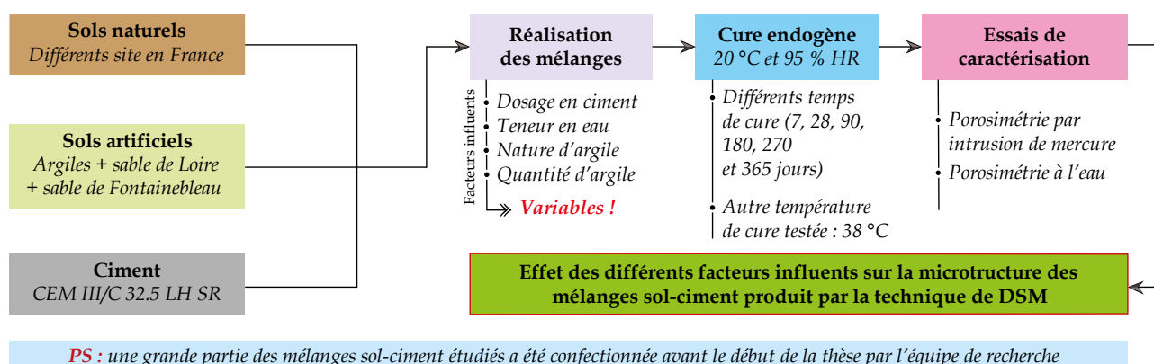
Fig. 95. Organigramme illustrant la démarche expérimentale adoptée pour l'étude des caractéristiques des pores des matériaux DSM
