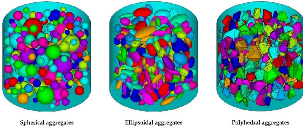
Fig. 44. Eprouvettes cylindriques avec différentes formes d'agrégats générées par la courbe de Fuller (Xu et al. 2016)
