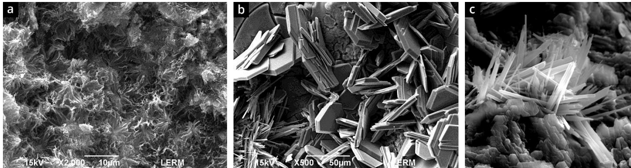
Fig. 291. Observations au MEB des hydrates : (a) CSH ; (b) Portlandite ( http://doc.lerm.fr/pouzzolanite-activite-pouzzolanique-et-hydraulite/ ) ; (c) ettringite (Pospišil et al. 2008)
