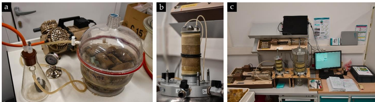
Fig. 66. (a) Saturation des échantillons de DSM sous vide ; (b) Montage d'une échantillon dans une membrane étanche ; (c) Dispositif de mesure de la perméabilité à l'eau dans une cellule triaxiale
