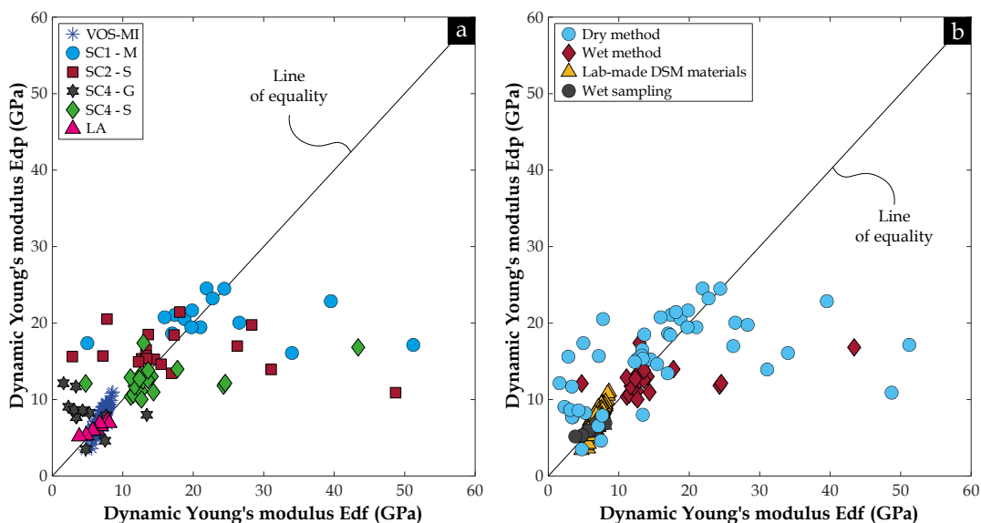
Fig. 193. Module d'Young dynamique E_{dp} basé sur la mesure de la vitesse d'ondes de compression V_p versus module d'Young dynamique E_{df} basé sur la mesure de fréquence de résonance f : (a) En représentant l'origine des échantillons ; (b) Mêmes données mais en indiquant la méthode de DSM utilisée sur site d'où proviennent les sondages carottés (sèche ou humide), les matériaux confectionnés en laboratoire et la méthode de prélèvement par voie humide [207 données]
