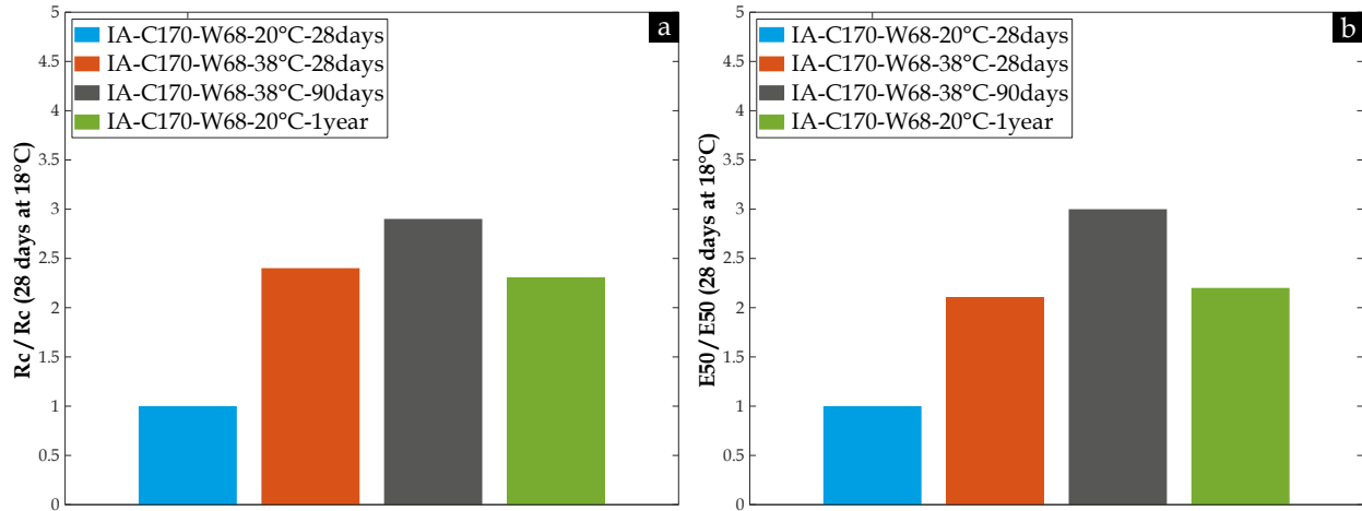
Fig. 106. Effet de la température de cure sur les propriétés mécaniques des matériaux DSM à base d'illite Arvel et une teneur en ciment CEM III/C de 170 kg/m 3 : (a) R_c ; (b) E_{50}
