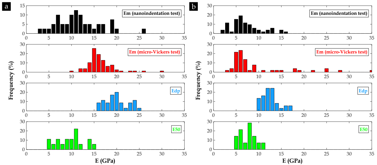
Fig. 341. Histogrammes illustrant les valeurs du module d'Young E_m évaluées par les tests de nanoindentation et de micro-dureté Vickers à l'échelle locale sur la matrice de sol-ciment, ainsi que les modules d'Young dynamique E_{dp} et statique E_{50} mesurés à l'échelle des éprouvettes décimétriques de DSM pour les deux carottes : (a) SC1-M ; (b) SC4-S
