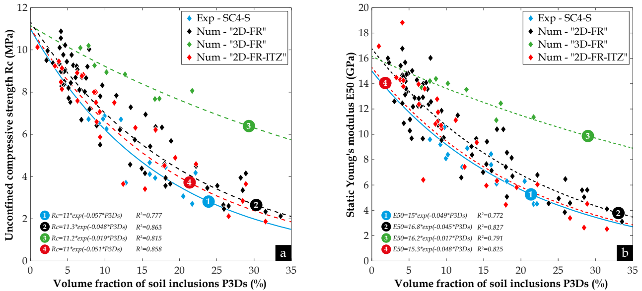
Fig. 260. Variation en fonction de la fraction volumique des inclusions de sol P 3Ds des propriétés mécaniques calculées sur les différents modèles géométriques "2D-FR", "3D-FR" et "2D-FR-ITZ", en comparaison aux valeurs expérimentales obtenues sur les éprouvettes de SC4-S : (a) R c ; (b) E 50
