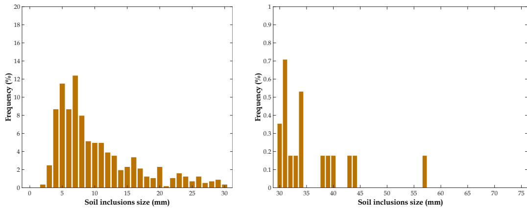
Fig. 311. Distribution de taille d'inclusions de sol en 2D des éprouvettes de SC2-S : (gauche) < 30 mm ; (droite) > 30 mm
