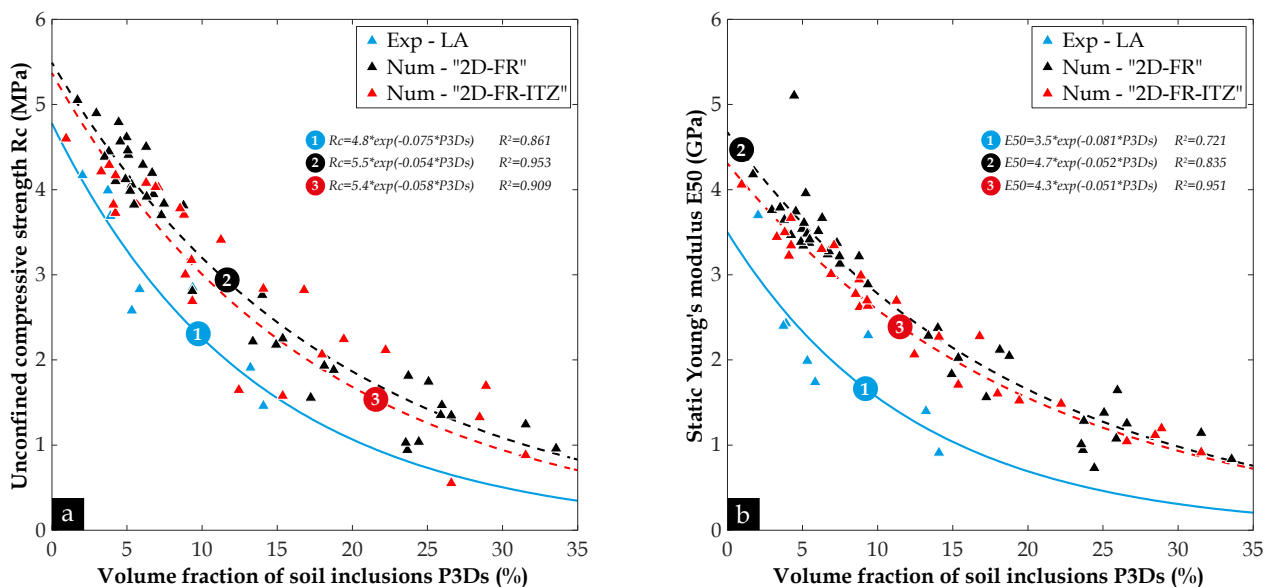
Fig. 261. Variation en fonction de la fraction volumique des inclusions de sol P 3Ds des propriétés mécaniques calculées sur les différents modèles géométriques "2D-FR" et "2D-FR-ITZ", en comparaison aux valeurs expérimentales obtenues sur les éprouvettes de LA : (a) R c ; (b) E 50
