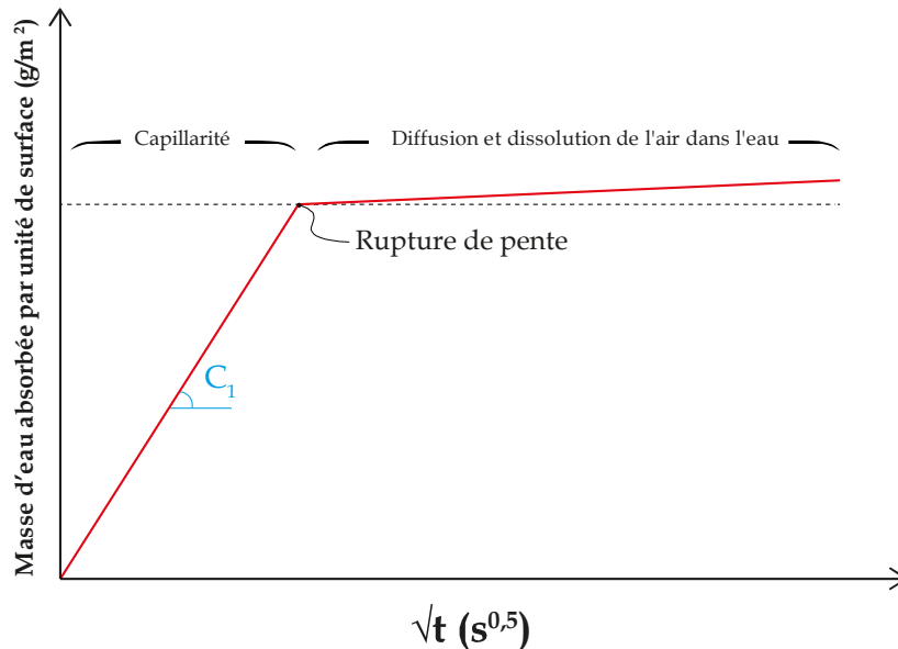
Fig. 69. Prise de poids cumulée en eau par unité de surface en fonction de la racine carrée du temps
