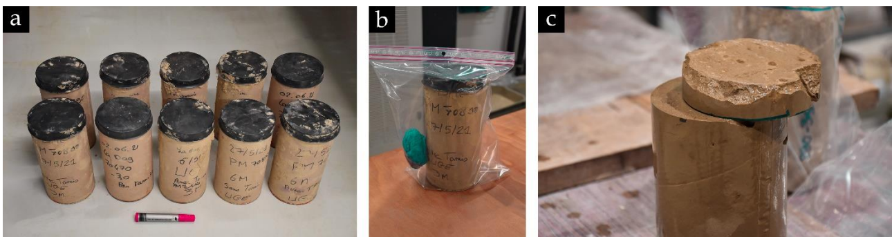
Fig. 52. (a) Huit éprouvettes moulées sur le site LA stockées en laboratoire ; (b) Eprouvette dans une double enveloppe hermétique ; (c) Eprouvette retaillée pour le test de résistance à la compression simple
