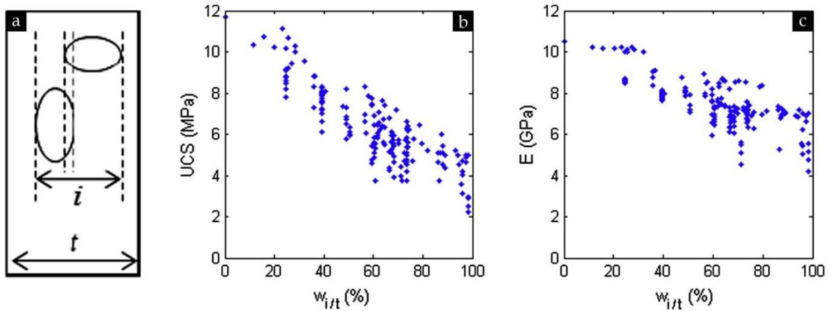
Fig. 32. (a) Illustration de la définition du rapport W_{i/t} ; (b) et (c) Relation entre la résistance à la compression et le module d'Young, respectivement, et le rapport W_{i/t} (Van Lysebetten et al. 2014)
