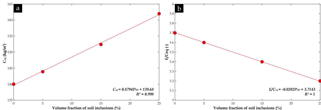
Fig. 64. Effet de la fraction volumique d'inclusions de sol sur : (a) Dosage en ciment équivalent C_{\text{eq}} ; (b) Rapport E/C_{\text{eq}}
