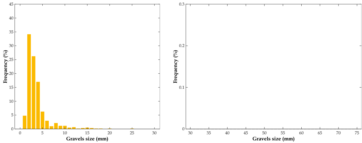
Fig. 317. Distribution de taille de graviers en 2D des éprouvettes de SC3-R : (gauche) < 30 mm ; (droite) > 30 mm
