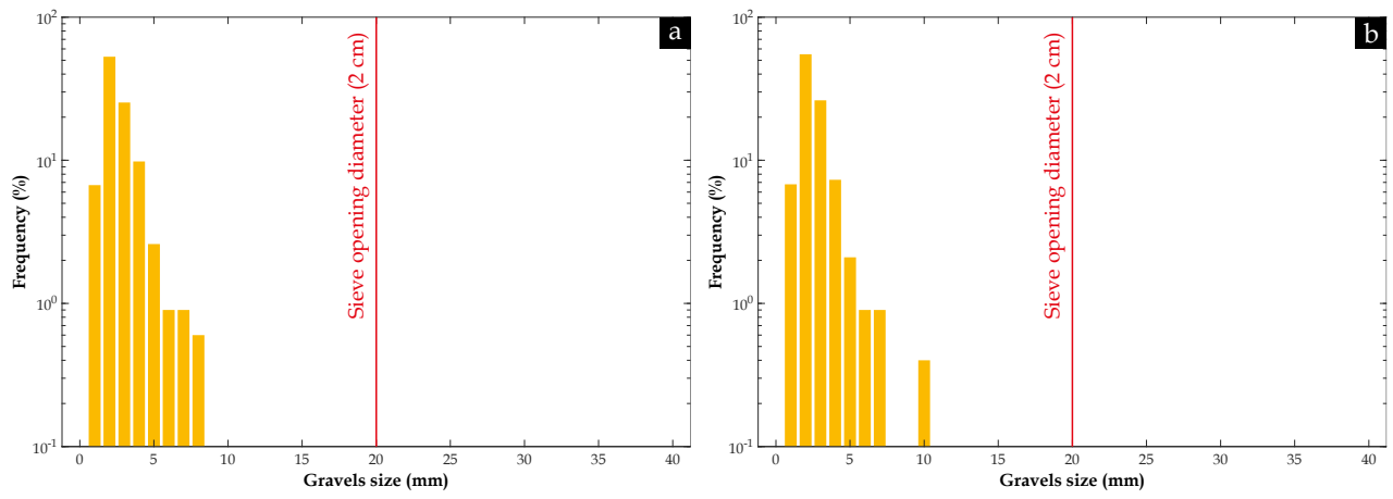
Fig. 332. Distribution de taille de graviers en 2D sur les découpes des 8 éprouvettes de LA : (a) 4 éprouvettes sans aucun criblage ; (b) 4 éprouvettes avec criblage au tamis à une maille de taille 20 mm
