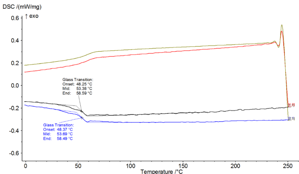
Figure 2.6 Analyse DSC pour l'adhésif polymérisé
