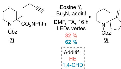
Schéma 113 : Cyclisation décarboxylante de l'ester de phthalimide 7j
