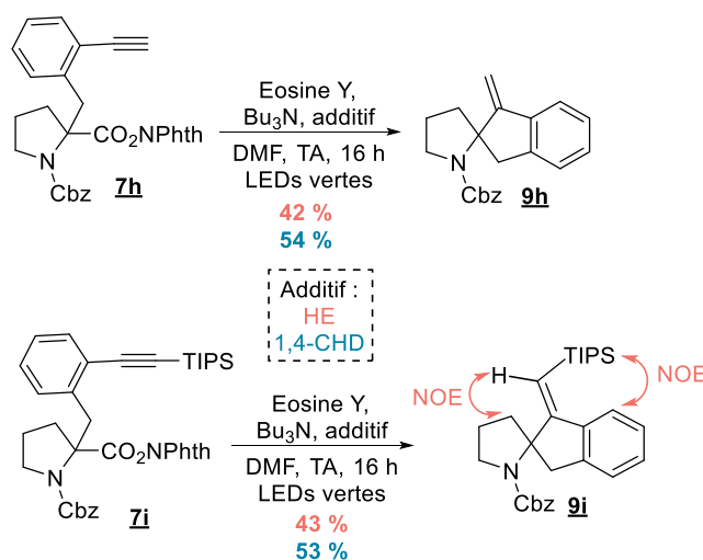
Schéma 106 : Catalyse photoredox des esters de phthalimidoyle 7h et 7i
