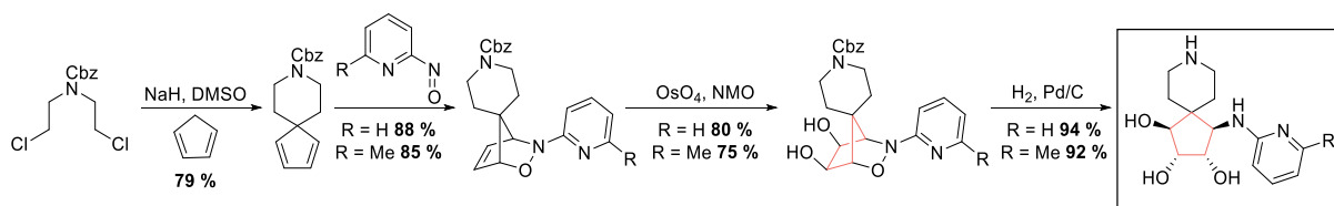
Schéma 19 : Utilisation de la réaction de nitroso Diels-Alder pour la formation d'un spiro-iminosucre
