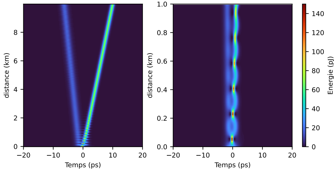
FIGURE 3.26 – Simulation numérique de (1.11) avec l'enregistrement 3.14 en condition initiale. \gamma = 1,3 \text{ W}^{-1} \text{ km}^{-1} , \beta_2 = -22 \text{ ps}^2/\text{km} , z = 1,10 \text{ km} À grande distance de propagation 10 km, l'impulsion se sépare en deux. Sur la distance de l'expérience (1 km) l'impulsion commence à se séparer bien que la simulation soit intégrable.
