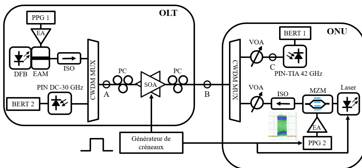
FIGURE 3.41 – Montage expérimental de test de technique d'AGC sur une transmission à 50 Gbit/s NRZ-OOK amplifiée à l'aide d'un SOA commun.
