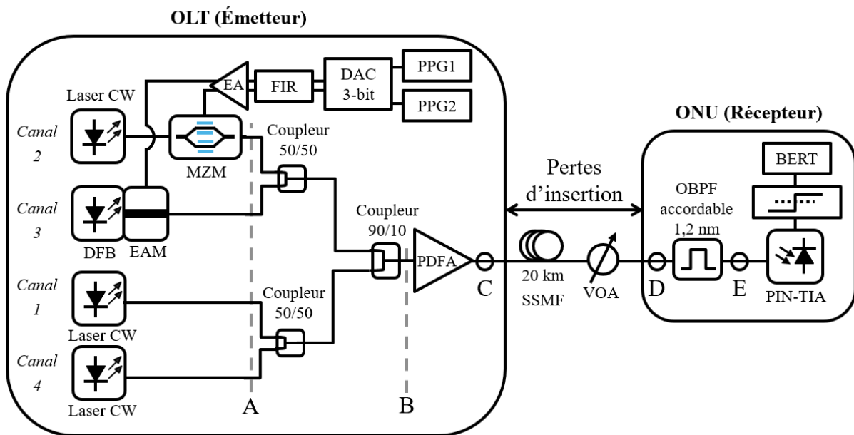
FIGURE 4.18 – Schéma expérimental du banc de test pour une longueur WDM à 4 longueurs d'onde à 100 Gbit/s avec un PDFFA booster.
