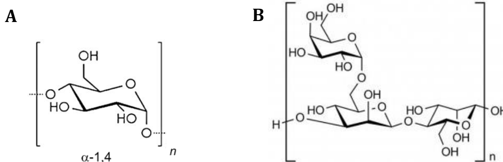
Figure 29. Représentation schématique des polymères de maltodextrine (A) et de galactomannane (B).
