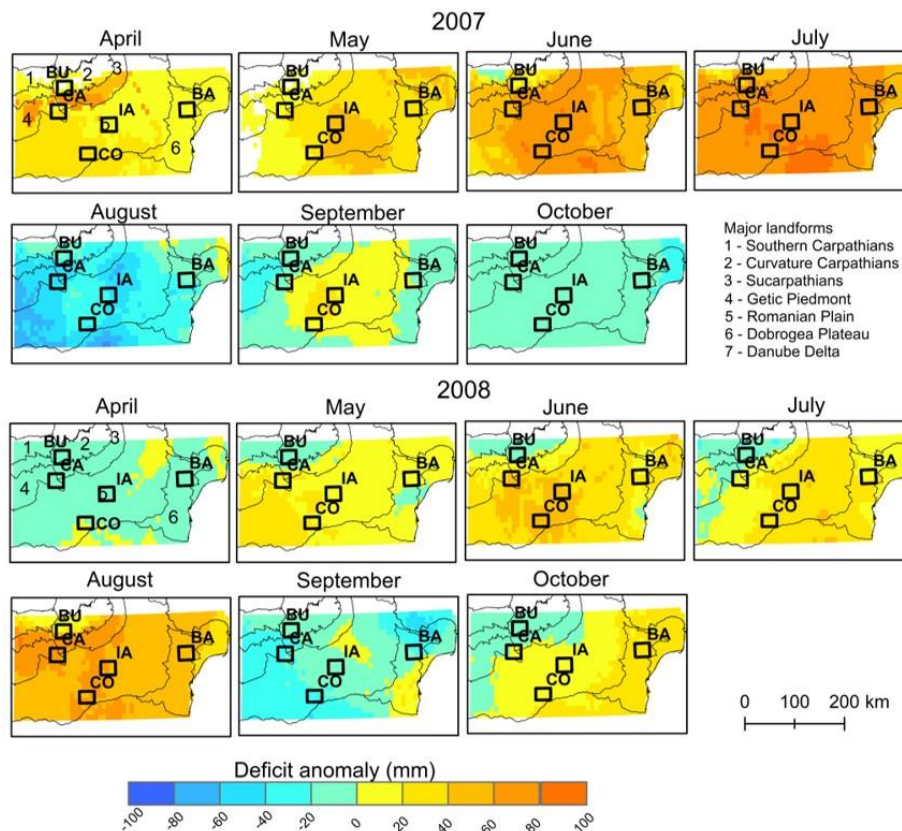
Figure 8.7 Anomalie raster-CWD mensuelle en 2007 et 2008 dans cinq zones d'étude : Babadag (BA), Bucegi (BU), Cândești (CA), Comana (CO) et Ialomița (IA).
