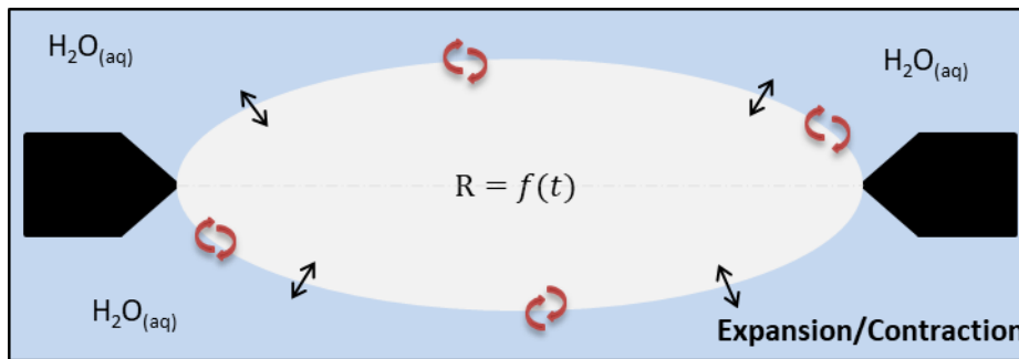
FIGURE 4.2 | Schéma de la phase de post-claquage. Les pointes noires représentent les électrodes d'un rayon de 50 \mu\text{m} , la partie bleue l'eau liquide et la partie blanche la phase gazeuse correspondant à notre domaine de simulation. Les doubles flèches indiquent que cette phase gazeuse subit des cycles d'expansion/contraction. Les flèches bordeaux représentent la diffusion de la phase gazeuse vers le liquide.
