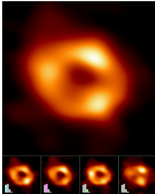
FIGURE 1.4 – Images reconstruites de Sgr A* créées par la collaboration EHT en combinant les images obtenues par les observations de l’EHT. L’image principale ( haut ) a été produite en moyennant plusieurs milliers d’images reconstruites, en utilisant plusieurs méthodes, qui ajustent les données observées. L’image moyennée montre les caractéristiques qui apparaissent le plus et réduit les particularités peu fréquentes. Les milliers d’images produites ont été regroupées en quatre catégories présentant les mêmes caractéristiques. Les quatre images en bas montrent l’image moyennée ainsi que la proportion d’image de chaque catégorie. Les trois premières montrent une forme d’anneau, mais avec une distribution différente de luminosité. Ces catégories représentent la majeure partie des images observées. La hauteur des barres indique le poids de chaque image dans l’image principale. Crédit : EHT Collaboration
