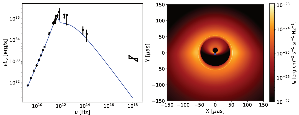
FIGURE 5.18 – Gauche : Spectre associé au meilleur ajustement du modèle de tore+jet (voir Table 5.1) pour l'état quiescent de Sgr A* ( \chi_{red}^2 = 0,91 avec ndof=27 ). Les données proviennent de [Bower, 2015] pour \nu < 50 GHz, [Brinkerink, 2015] pour les deux points autour de 100 GHz, [Liu, 2016] pour le point à 492 GHz, [Marrone, 2006] pour le point 690 GHz, [von Fellenberg, 2018] pour les limites supérieures dans l'infrarouge lointain, [Witzel, 2018] pour les données dans l'infrarouge moyen, et [Baganoff, 2001] pour le nœud papillon en rayons X. On note que, comme pour [Vincent, 2019b], les données relatives aux rayons X n'ont pas été ajustées, car nous n'avons pas pris en compte l'émission Bremsstrahlung ou Compton inverse. Droite : Image du meilleur ajustement à 2,2 \mu\text{m} du modèle de tore+jet avec un champ de vision de 300 \mu\text{as} vu avec une inclinaison de 20^\circ et un PALN de \pi rad. La barre de couleur donne les valeurs de l'intensité spécifique en unités cgs en échelle logarithmique. L'émission de la région extérieure provient du jet arrière, et l'émission proche du centre provient de la partie avant du jet. Le centroïde du jet est représenté par le point bleu à \sim(0, -2, 2) .
