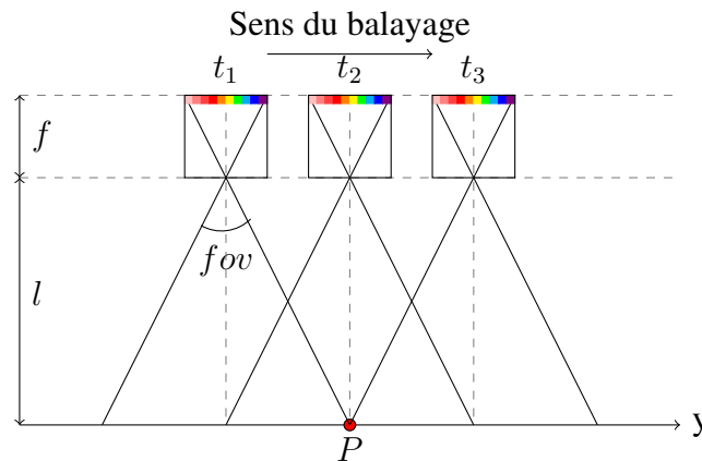
(a) Vue schématique de côté de l'observation d'une scène par notre caméra.
