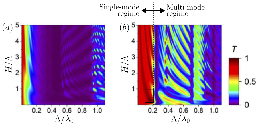
Figure 4.4: Cartographie théorique de la transmission en incidence normale de la configuration T-TM composée d'un substrat de GaAs et de 50 nm d'or, pour (a) la polarisation TE, et (b) la polarisation TM. Le rectangle noir représente la gamme de valeurs utilisées pour la période du réseau et la hauteur des dents de semi-conducteur lors de l'optimisation de la structure. Ces images proviennent de [2].
