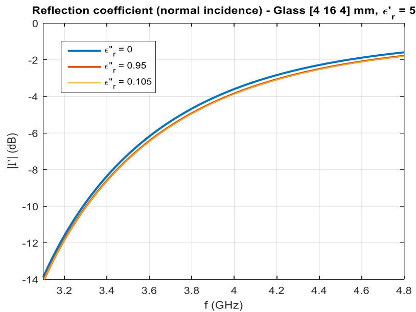
Figure 32 Evolution du coefficient de réflexion |\Gamma| en fonction de la fréquence pour différentes valeurs de pertes diélectriques du verre.
