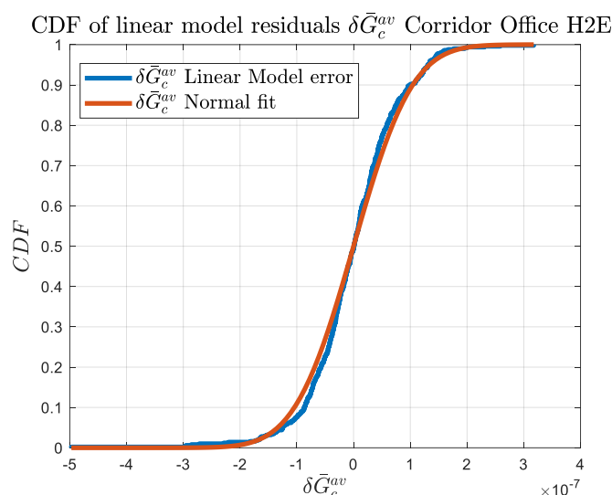
Figure 52 CDF des résiduels \delta\bar{G}_c^{av} . Corridor Office (H2E).
