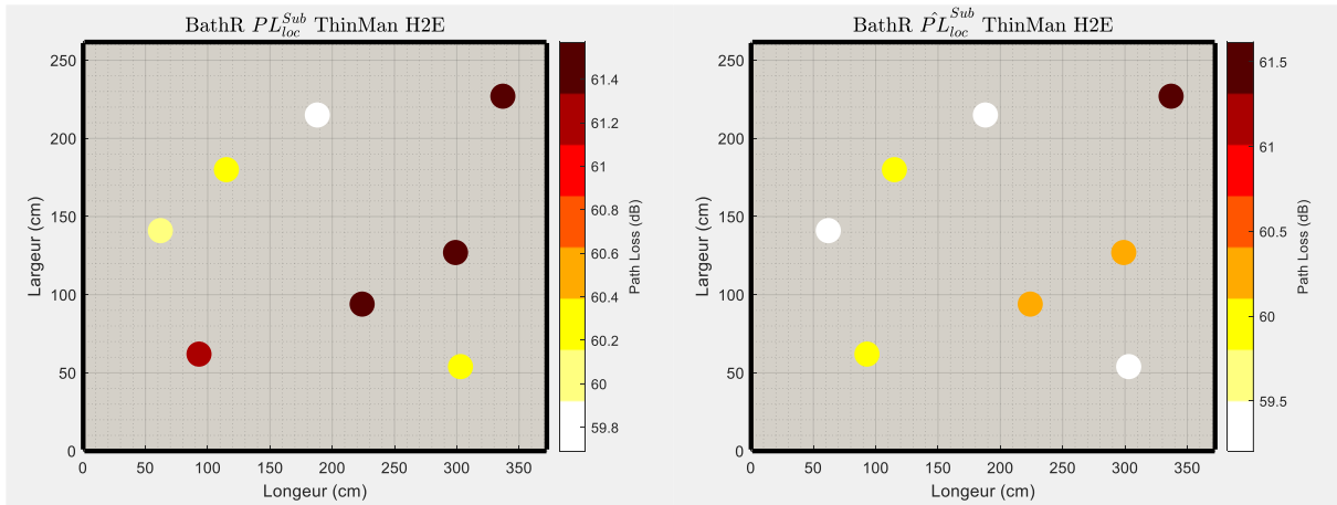
Figure_Annexe 120 PL_{loc}^{Sub} et \widehat{PL}_{loc}^{Sub} : Salle de bain, H2E.
