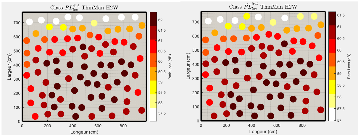
Figure_Annexe 122 PL_{loc}^{Sub} et \widehat{PL}_{loc}^{Sub} : Classe, H2W.
