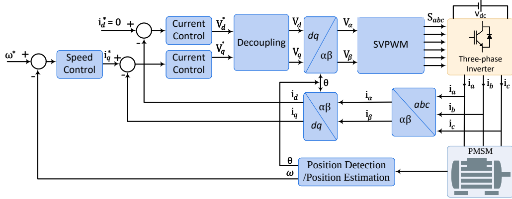
Figure 6.3: Schéma de la commande FOC du PMSM.
