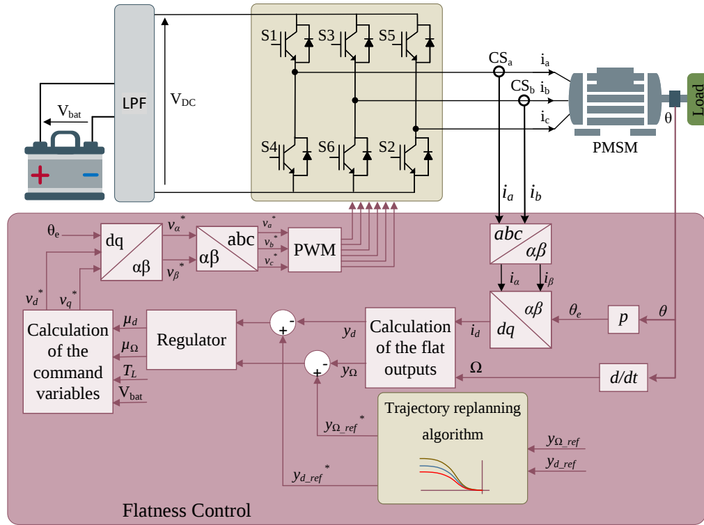
Figure 6.4: Schéma de la commande d'un PMSM basée sur la planéité.
