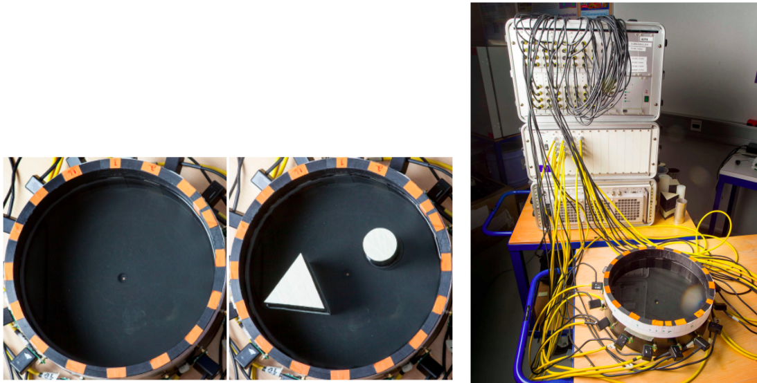
Fig. 6.6 : À gauche : une configuration expérimentale pour la collecte de données EIT en 2D avec une configuration homogène et une autre avec deux inclusions plastiques. À droite : le système de mesure KIT4 à l'Université de Eastern-Finland [80]. Images issues de [80]
