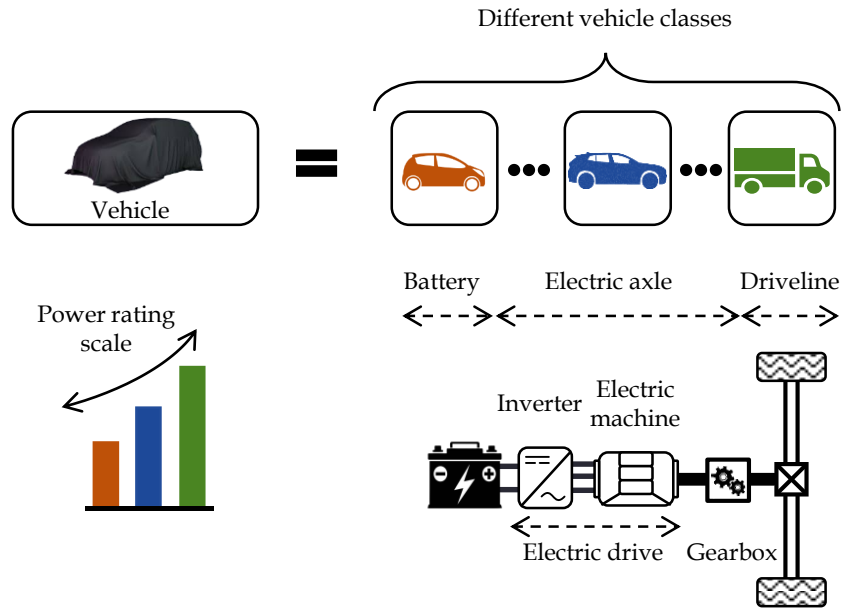
Fig. 79: Powertrain layout
