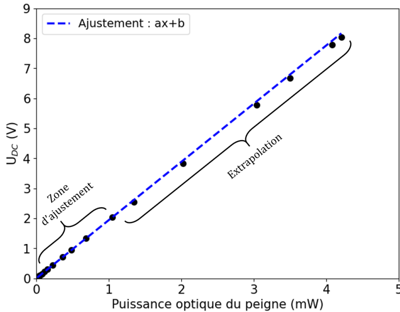
FIGURE 4.8 – Variation de la tension continue U_{DC} en fonction de puissance optique du peigne. En traits bleus : Ajustement linéaire avec la fonction ax + b ( a=1,94 V/mW, b \simeq 0 ).
