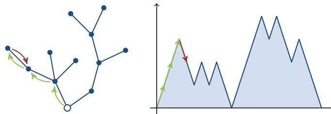
FIGURE 4 – Un arbre t (ordonné) et sa fonction de contour.
