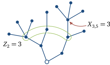
FIGURE 1 – Un arbre de Galton-Watson et le processus sous-jacent.
