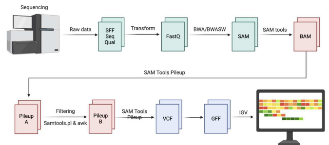
Fig. 2.3.: NGS workflow
