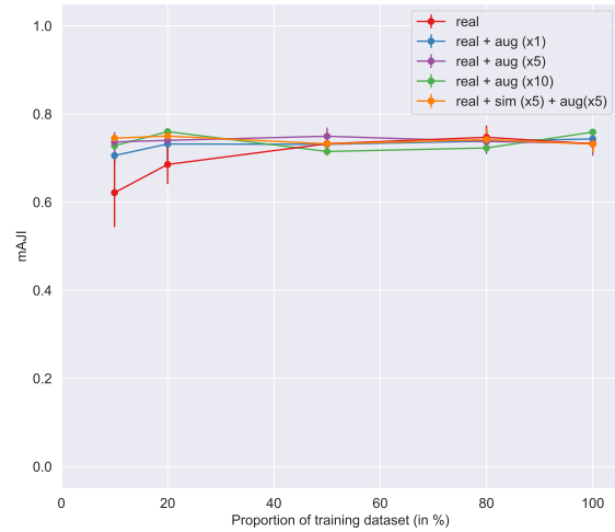
(d) Cellpose perf. on DSB 2018, data augmentation.
