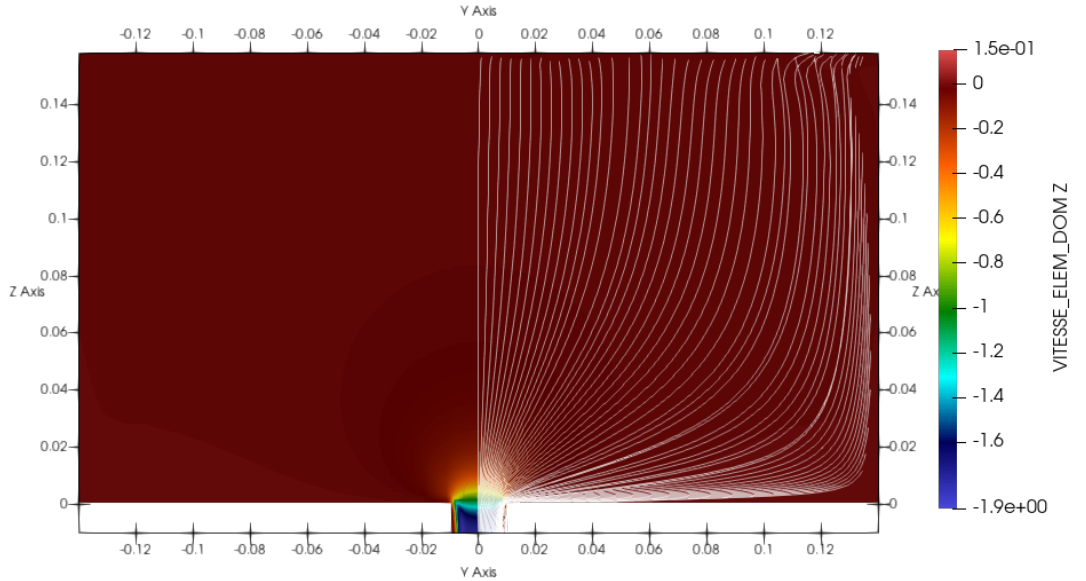
FIGURE 1.1 : Simulation numérique réalisée avec TrioCFD. Cas d'une vidange sans rotation. La colorimétrie représente la composante axiale de la vitesse en \text{m.s}^{-1} . Les lignes de courant sont tracées à droite. Les lignes de courant sont verticales proches de l'interface, alors qu'elles convergent toutes vers la section de vidange en proximité de celle-ci.
