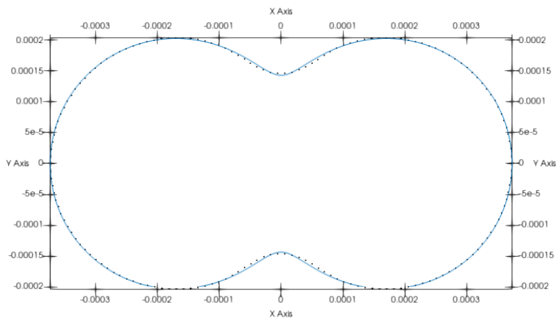
FIGURE 6.2 : a. Profils paramétriques pour (a) t = 0.001 s, (b) t = 0.004 s et (c) t = 0.008 s. La représentation paramétrique d'Hopper est donnée en trait continu bleu, les résultats numériques sont en pointillés. Le décalage temporel induit par la discrétisation en t = 0 s est pris en compte dans les profils comparés.
