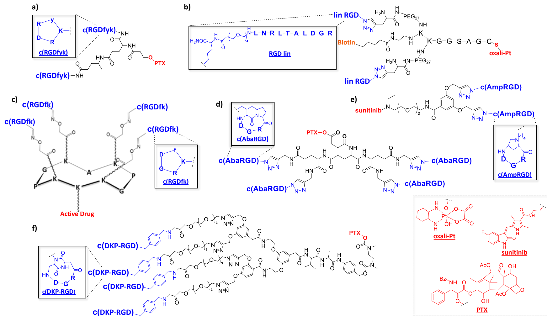
Figure 13 : Structures de constructions multimériques de RGD. a) c(\text{RGD}) -paclitaxel; b) « c(\text{RGD}) -Y-shaped peptide core»; c) «tetrameric c(\text{RGD}) -containing cyclodecapeptide»; d) « c(\text{AbaRGD}) -glutamic acide dendrons»; e) ligation c(\text{AmpRGD}) -triazole/ether/amide. Adapté de la revue de Cossu et al. 178
